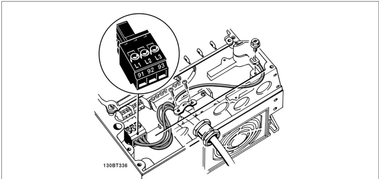
圖 4.6: 如何在不使用主電源斷開連接開關的情況下連接至主電源與接地。請注意此處使用了電纜線夾鉗。
