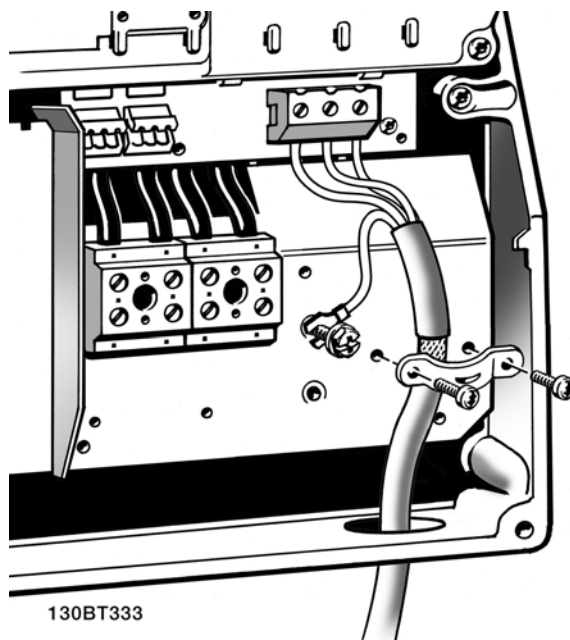
圖 4.14: 首先將馬達地線終接，然後將馬達 U、V 與 W 電線放進端子並鎖緊。請確保馬達電纜線外部絕緣已從 EMC 夾鉗下移除。
