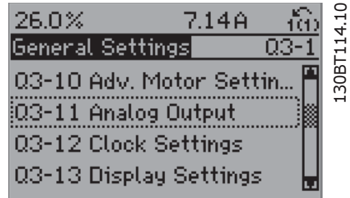
图 6.6: 步骤 5: 使用向上/向下导航键向下滚动到目标选项, 比如 03-11 模拟输出。按 [OK] (确定)。
