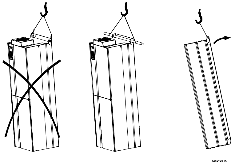
图 3.1: 对于较重的变频器, 请使用提升设备。首先以墙面安装方式安装两个较低的螺栓, 然后将变频器抬起放在这两个较低的螺栓上, 最后使用两个较高的螺栓将变频器靠近墙面拧紧。
