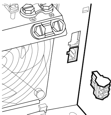
图 4.36: B3 的继电器连接端子。出厂时只由一个挡板。
