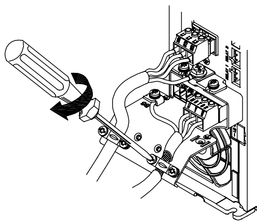
图 4.17: 安装电缆夹, 以确保机架和屏蔽丝网达到 360 度连接。注意, 请去除电缆夹下面电动机电缆的外部绝缘层。
