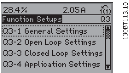
图 6.5: 步骤 4: 随即会显示功能设置选项。选择 03-1 一般设置。按 [OK] (确定)。
