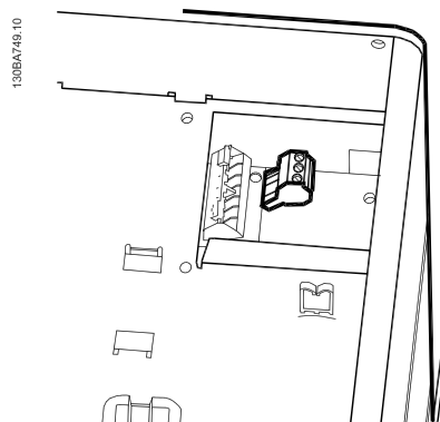
Bild 4.37: Plintar för reläanslutningar för C3 och C4. Sitter i det övre högra hörnet på frekvensomformaren.
