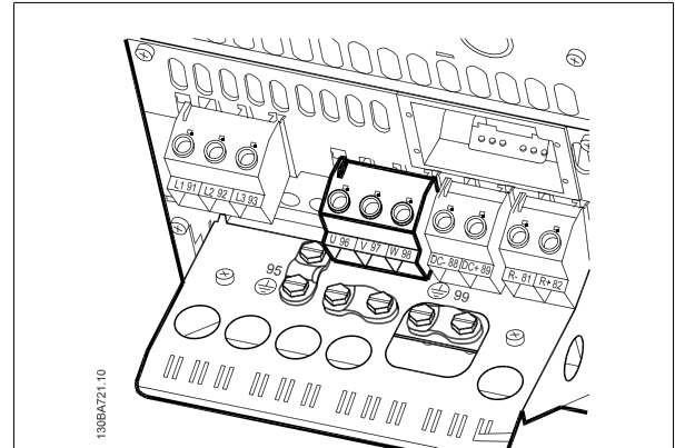
Bild 4.22: Avsluta först motorns jordanslutning, placera sedan motorns U-, V- och W-ledningar i plinten och dra åt. Se till att den yttre isoleringen på motorkabeln tas bort under EMC-klämman.
