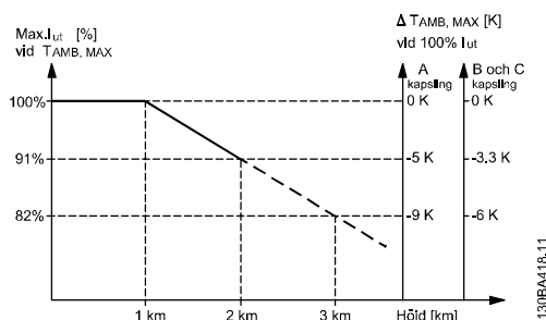
Bild 9.1: Nedstämpling av utström visavi höjd vid T_{AMB, MAX} för ramstorlekar A, B och C. Vid höjdskillnader över 2 km kontakta Danfoss om PELV.
