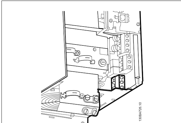
Bild 4.21: Avsluta först motorns jordanslutning, placera sedan motorns U-, V- och W-ledningar i plinten och dra åt. Se till att den yttre isoleringen på motorkabeln tas bort under EMC-klämman.
