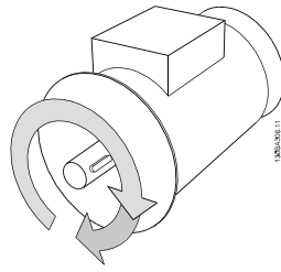
Bild 4.49: Steg 9: Byt ut två motorledningar om du inte får önskad rotationsriktning.
