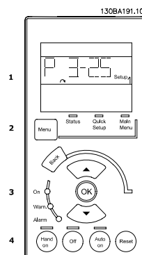
Bild 6.1: Numerisk LCP (NLCP)
