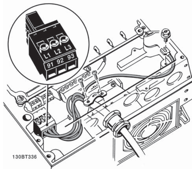
Εικόνα 4.7: Τρόπος σύνδεσης δικτύου ρεύματος και γείωσης χωρίς γραμμή διακόπτη απόζευξης δικτύου ρεύματος. Λάβετε υπόψη ότι χρησιμοποιείται σφιγκτήρας καλωδίου.
