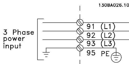
Εικόνα 4.2: Ακροδέκτες για δίκτυο ρεύματος και γείωση.
