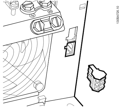
Çizim 4.35: B3 röle bağlantıları için terminaller. Fabrikada yalnızca tek bir röle girişi takılır. İkinci röle gerekirse, takma kapağını çıkarın.
