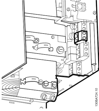
Çizim 4.30: B3 için fren bağlantı terminali.
