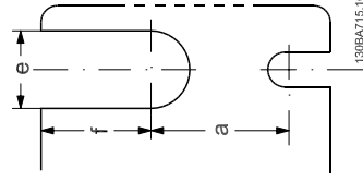
Çizim 3.2: Üst ve alt montaj delikleri. (yalnızca B4+C3+C4)
