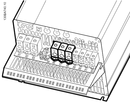
Çizim 4.25: Öncelikle motorun toprak bağlantısını kesin, ardından motordaki U, V ve W tellerini uygun terminallere yerleştirin ve sıkıştırın. Motor kablosunun dış yalıtımının EMC kelepçesinin altından çıkartıldığından emin olun.
