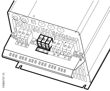
Çizim 4.24: Öncelikle motorun toprak bağlantısını kesin, ardından motordaki U, V ve W tellerini uygun terminallere yerleştirin ve sıkıştırın. Motor kablosunun dış yalıtımının EMC kelepçesinin altından çıkartıldığından emin olun.
