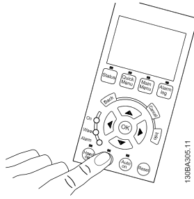
圖 4.44: 步驟 4: 將裝置上電並按下 [Off] (關閉) 按鈕。在此狀態下，馬達不應轉動。按下 [Off] 可在任何時間停止馬達。請注意 [Off] 按鈕的 LED 應當亮起。如果警報或警告正在閃爍，請參閱第 7 章有關此部分的說明。
