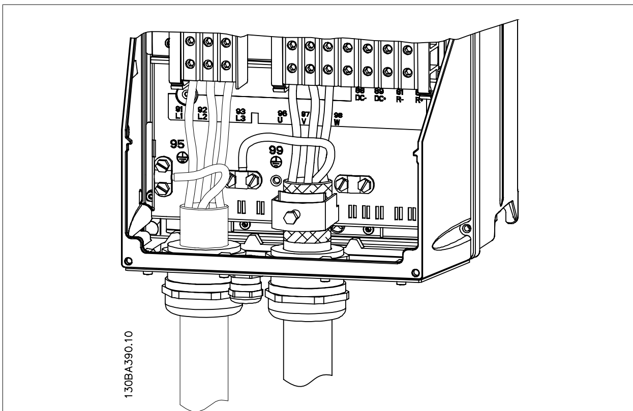
圖 4.23: 首先將馬達以端接方式接地，然後將馬達 U、V 與 W 電線放進端子並扭緊。請確保位於 EMC 夾鉗下方的馬達電纜線外部絕緣已取下。
