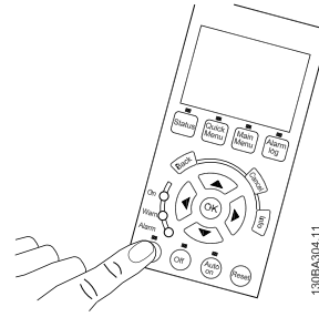
圖 4.45: 步驟 5: 按下 [Hand on] 按鈕，按鈕上的 LED 應當亮起且馬達可能轉動。
