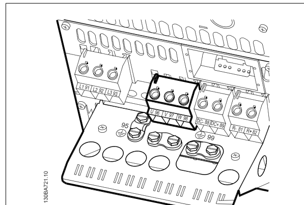
圖 4.22: 首先將馬達以端接方式接地，然後將馬達 U、V 與 W 電線放進端子並扭緊。請確保位於 EMC 夾鉗下方的馬達電纜線外部絕緣已取下。
