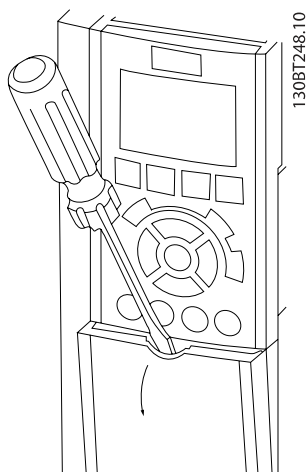
Disegno 4.32: Accesso ai morsetti di controllo per le custodie A2, A3, B3, B4, C3 e C4
