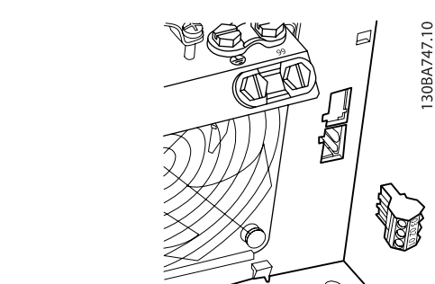
Disegno 4.29: Morsetti per i collegamenti relè per B3. Un solo ingresso relè è fornito dalla fabbrica. Quando è necessario il secondo relè, togliere il pezzo che copre il foro passacavo.
