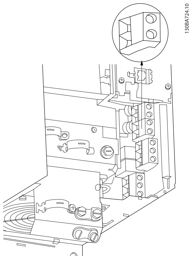
Disegno 4.24: Morsetto di collegamento freno per B3.
