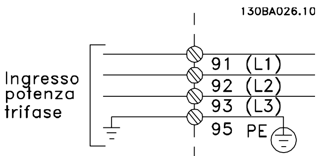
Disegno 4.2: Morsetti per la rete e la messa a terra.
