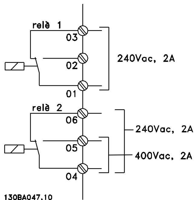
Disegno 4.31: Morsetti per i collegamenti relè per C3 e C4. Posizionati nell'angolo superiore destro del convertitore di frequenza.
