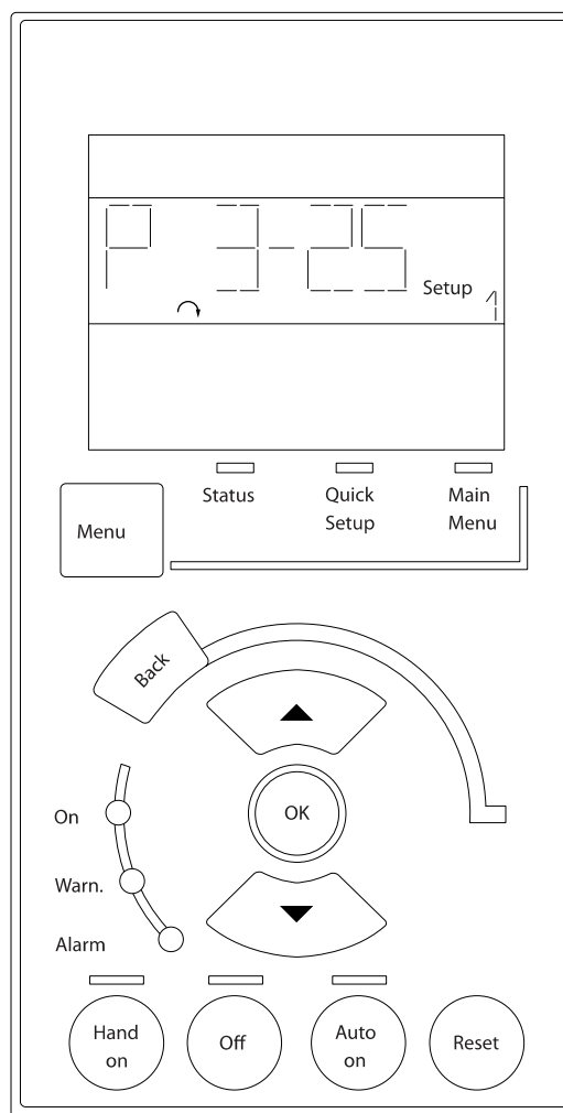
Disegno 6.1: LCP numerico (NLCP)
