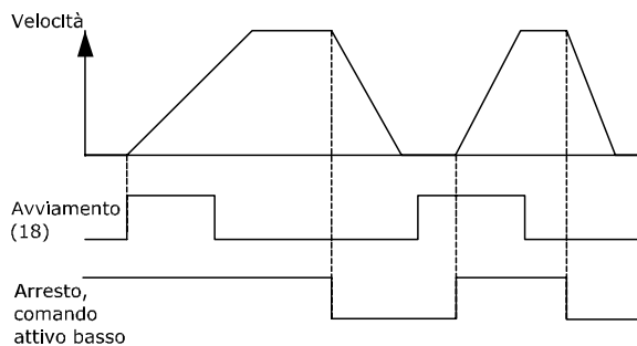
Disegno 5.5: Morsetto 37: solo disponibile con arresto di sicurezza!
