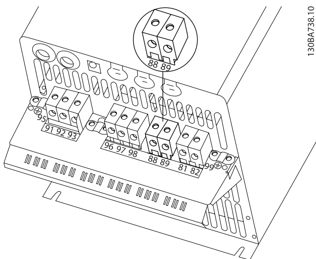
Disegno 4.22: Collegamenti bus CC per custodia C3.
