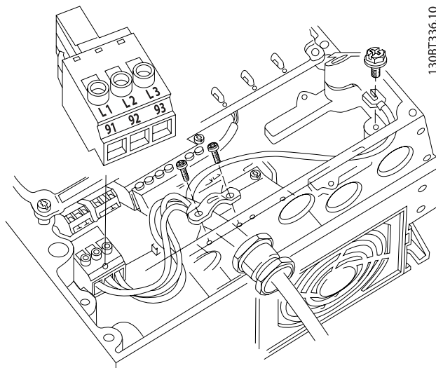
Disegno 4.7: Come effettuare il collegamento alla rete e messa a terra senza sezionatore di .. Tenere presente che viene utilizzato un pressacavo.
