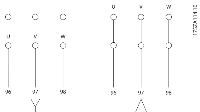
Disegno 4.16: Morsetti per il collegamento del motore
