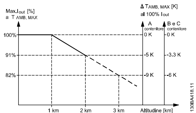
Disegno 9.1: Declassamento della corrente di uscita rispetto all'altitudine, con T_{AMB, MAX} per telai di taglia A, B e C. Per altitudini superiori ai 2000 m, contattare Danfoss per informazioni sulle caratteristiche PELV.
