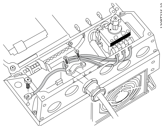
Disegno 4.8: Collegamento alla rete e messa a terra con sezionatore di rete.
