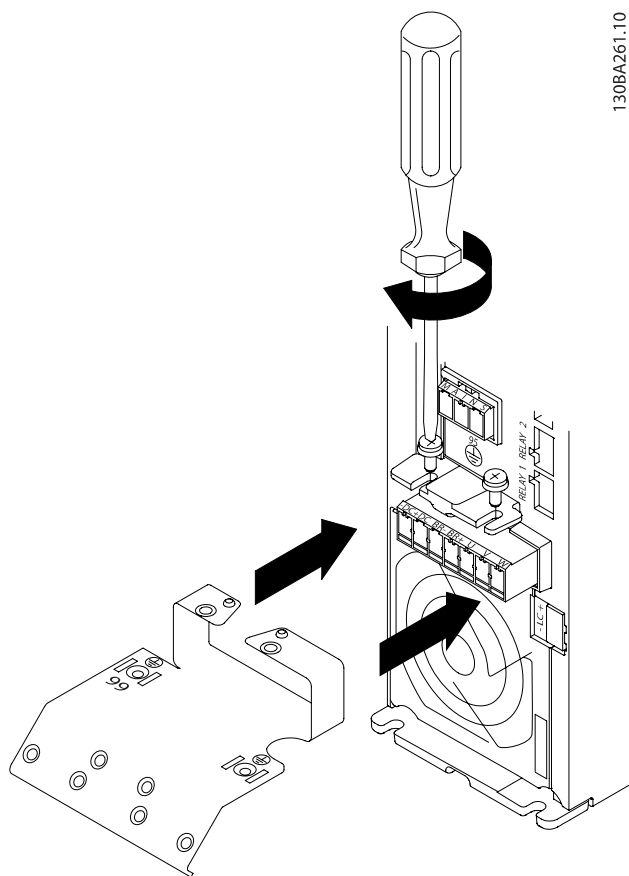
Disegno 4.3: Prima inserire le due viti sulla piastra di montaggio, spingerle in posizione e serrarle completamente
