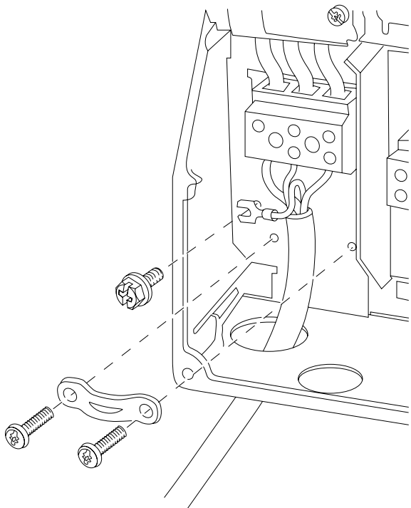
Disegno 4.9: Collegamento alla rete e messa a terra per B1 e B2
