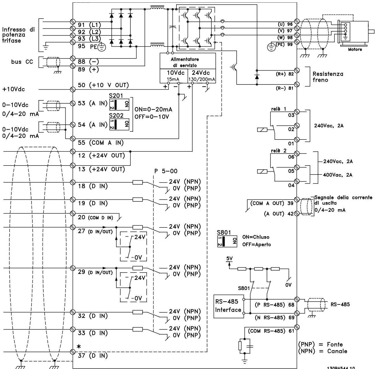
Disegno 4.1: Grafico mostrante tutti i morsetti elettrici. (Il morsetto 37 è solo presente per unità con funzione di arresto di sicurezza).
