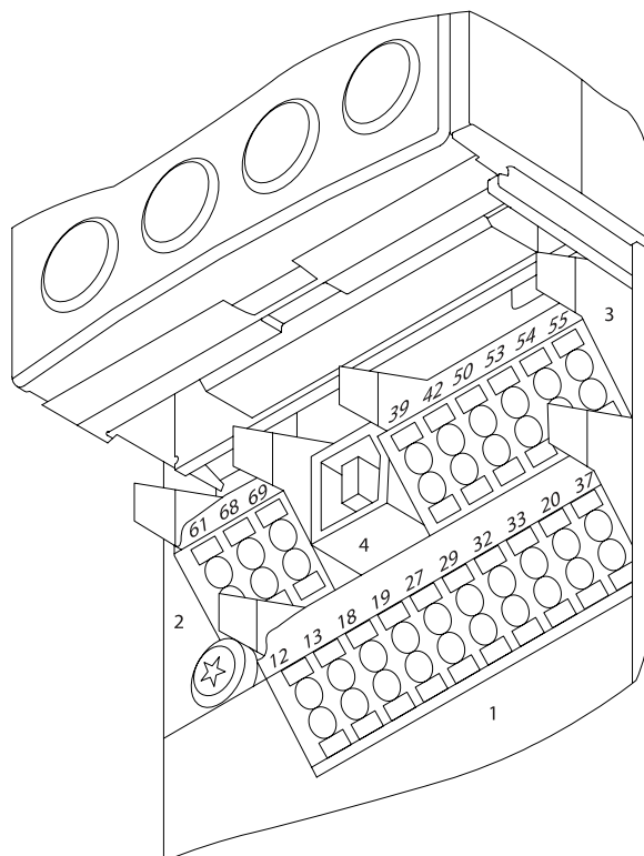
Disegno 4.34: Morsetti di controllo (tutte le custodie)
