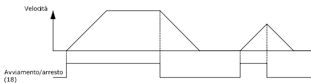
Disegno 5.4: Morsetto 37: solo disponibile con arresto di sicurezza!
