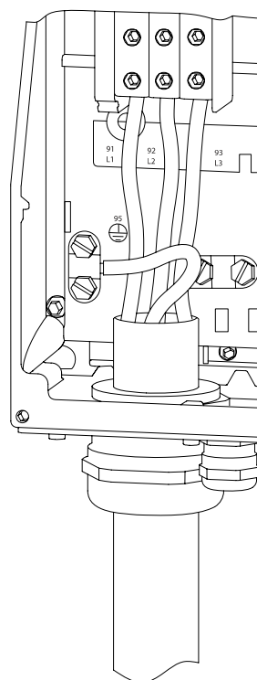
Disegno 4.13: Collegamento alla rete e messa a terra per C1 e C2.
