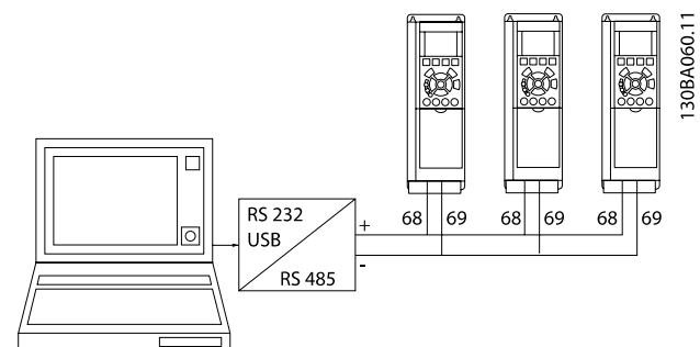
Bild 5.2: Anslutningsexempel.
