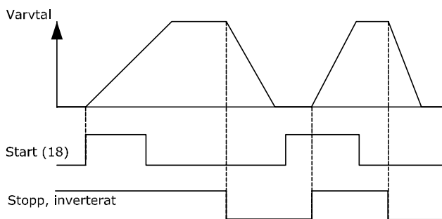
Bild 5.5: Plint 37: Endast tillgänglig med funktion för säkerhetsstopp!
