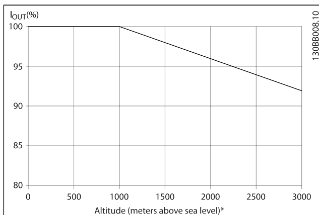
Nedstämpling av utström visavi höjd vid T AMB, MAX för ramstorlekar D, E och F.
