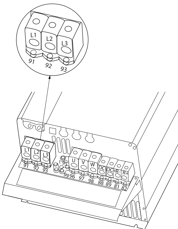
Bild 4.15: Så här ansluter du C4 till nät och jordning.
