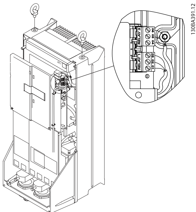
Bild 4.28: Plintar för reläanslutning (Ramstorlekar C1 och C2). Reläanslutningarna visas i håltagningarna med reläkontakterna (från tillbehörspåsen) monterade.
