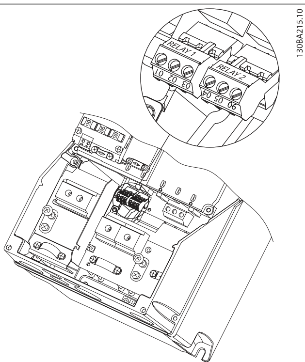
Plintar för reläanslutning (kapslingar A4, A5, B1 och B2).
