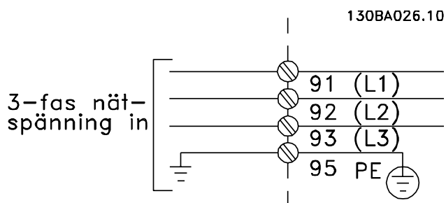
Bild 4.2: Plintar för nät och jordning.
