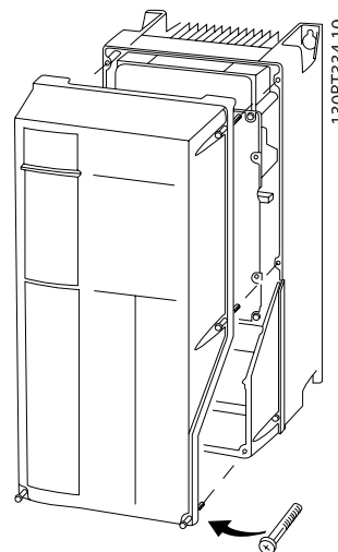
Bild 4.33: Åtkomst till styrplintar för A4-, A5-, B1-, B2-, C1- och C2-kapslingar
