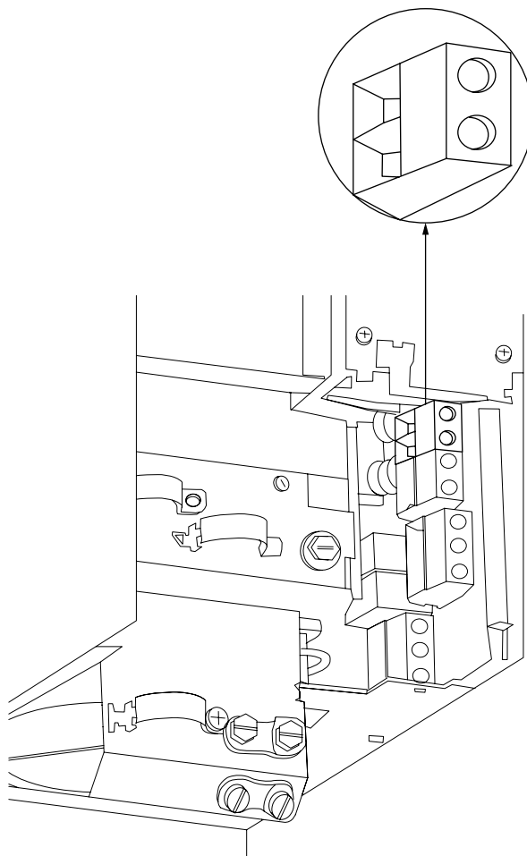
Bild 4.20: Likströmsbussanslutningar för kapsling B3.
