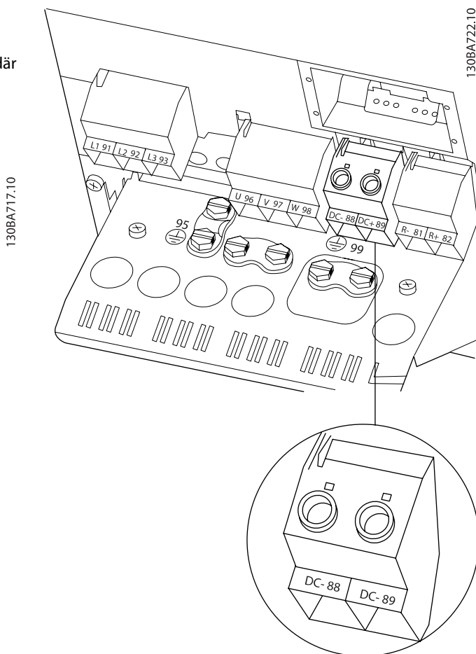
Bild 4.21: Likströmsbussanslutningar för kapsling B4.
