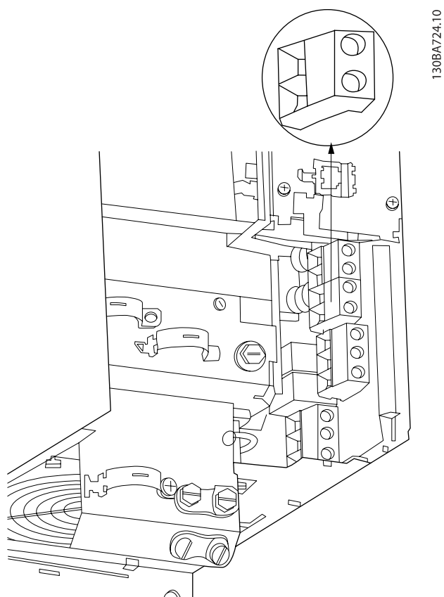
Bild 4.24: Bromsanslutningsplinten för B3.
