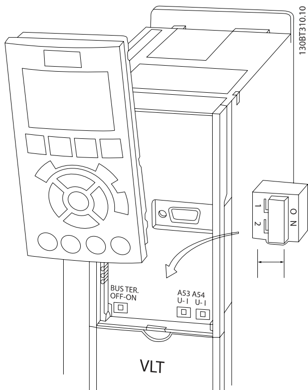
Bild 4.44: Brytarnas placering.
