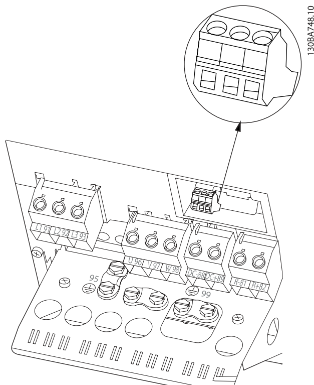
Bild 4.30: Plintar för reläanslutning B4.
