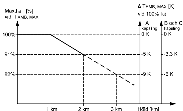
Bild 9.1: Nedstämpling av utström visavi höjd vid T AMB, MAX för ramstorlekar A, B och C. Vid höjdskillnader över 2 km kontakta Danfoss om PELV.
