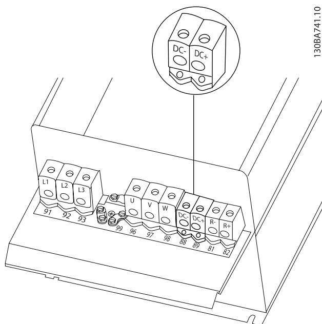
Bild 4.23: Likströmsbussanslutningar för kapsling C4.
