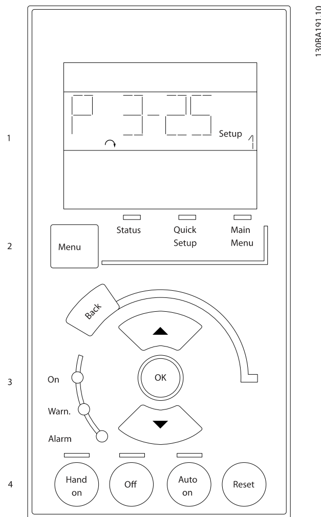
Bild 6.1: Numerisk LCP (NLCP)
