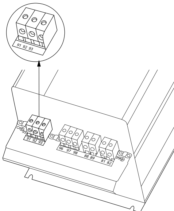
Bild 4.14: Så här ansluter du C3 till nätet och jordning.
