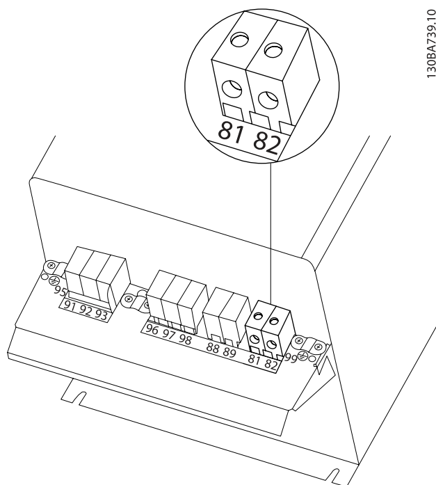
Bild 4.26: Bromsanslutningsplinten för C3.
