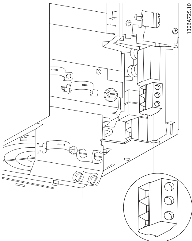
Bild 4.10: Så här ansluter du till nät och jordning för B3 utan RFI.
