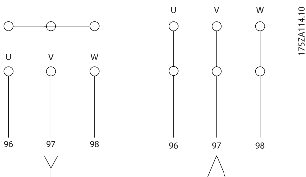
Bild 4.16: Plintar för motoranslutning
