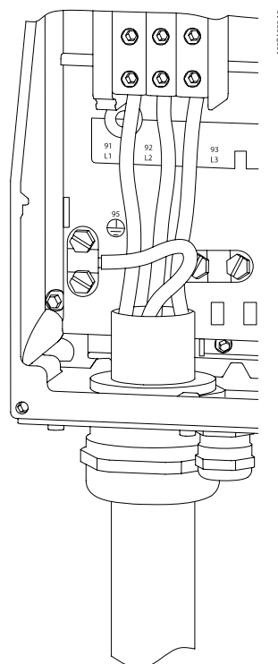
Bild 4.13: Så här ansluter du C1 och C2 till nät och jordning.
