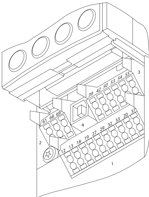
Bild 4.34: Styrplintar (alla kapslingar)
