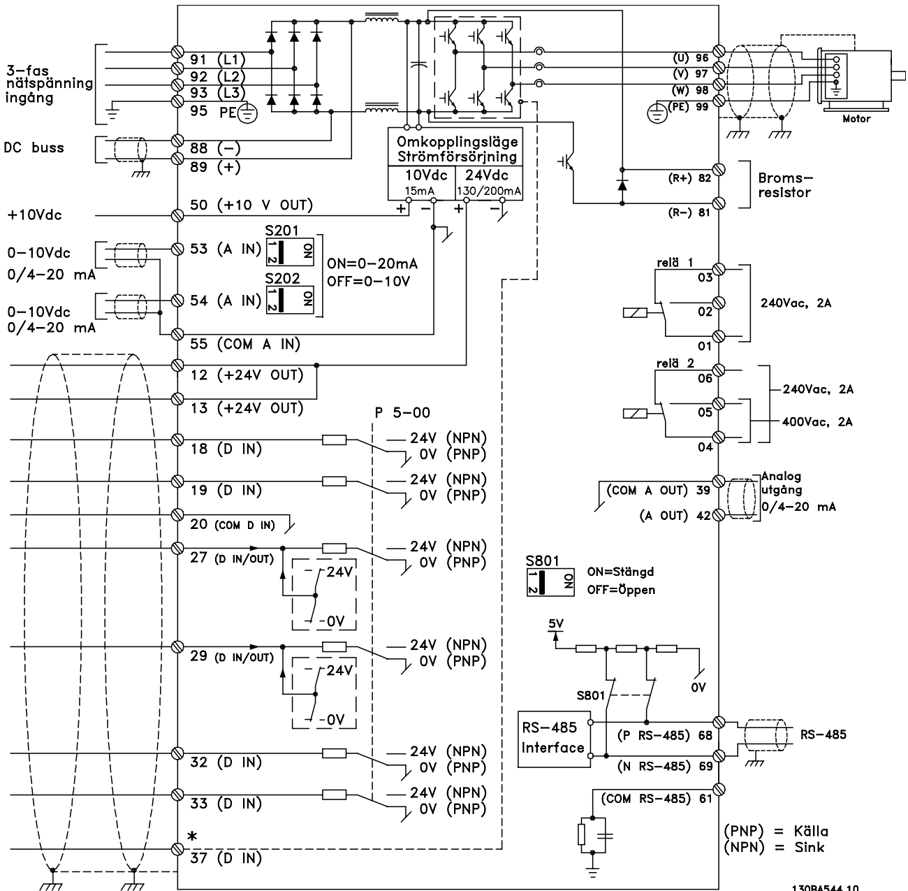
Bild 4.1: Diagram över alla elektriska plintar. (Plint 37 fungerar enbart med enheter som har funktionen säkerhetsstopp.)
