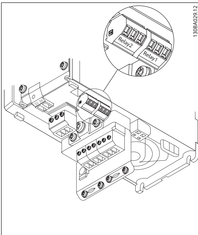
Plintar för reläanslutning (A2- och A3-kapslingar).
