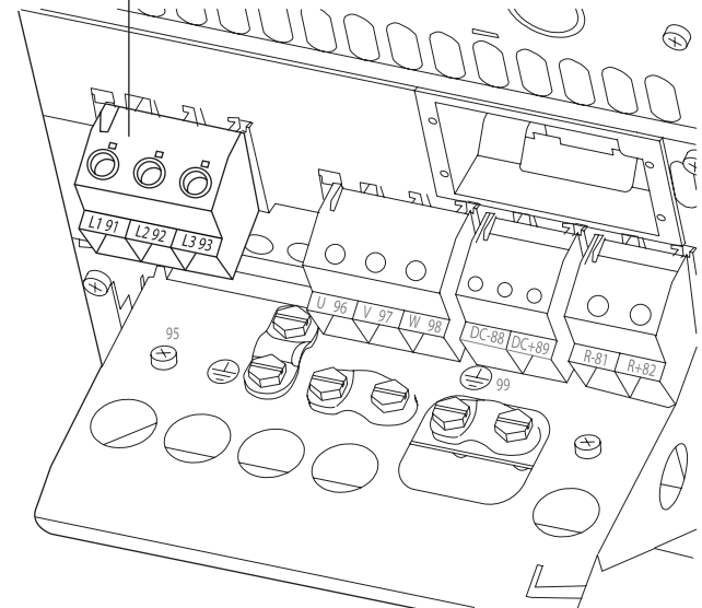
Kuva 4.12: Verkkovirran ja maadoituksen kytkeminen B4-runkokokoon.
