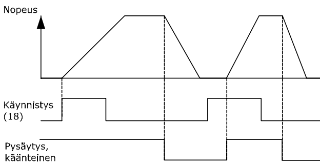
Kuva 5.5: Liitin 37: Saatavana vain turvapysäytystoiminnon yhteydessä!
