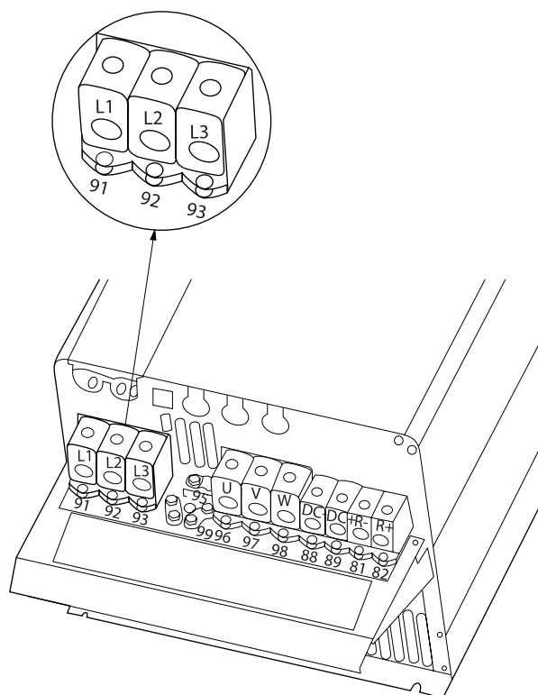
Kuva 4.15: C4 kytkeminen verkkovirtaan ja maadoitukseen.
