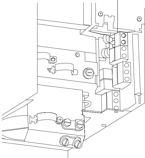
Kuva 4.20: Tasavirtaväyläyhteiset koteloon B3.
