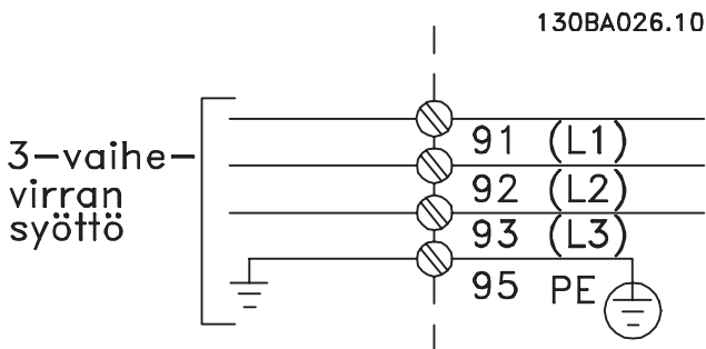
Kuva 4.2: Verkkovirta- ja maadoitusliittimet.
