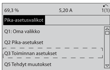
Kuva 7.3: Vaihe 3: Vieritä kohtaan Toimintoasetukset navigointinäppäimillä ylös/alas. Paina [OK]-näppäintä.
