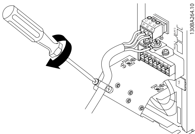
Kuva 4.6: Kiristä lopuksi verkkovirtajohdinten tukikiinnike.
