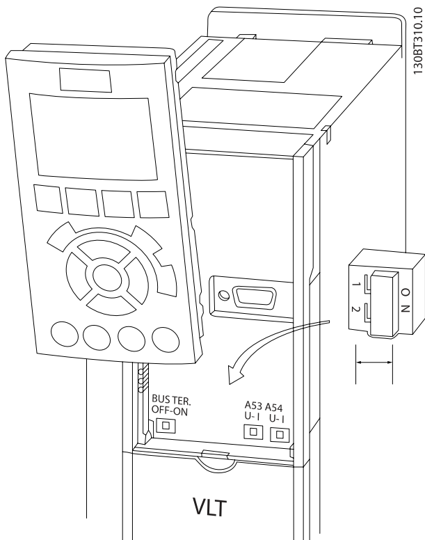
Kuva 4.44: Katkaisinten sijainti.
