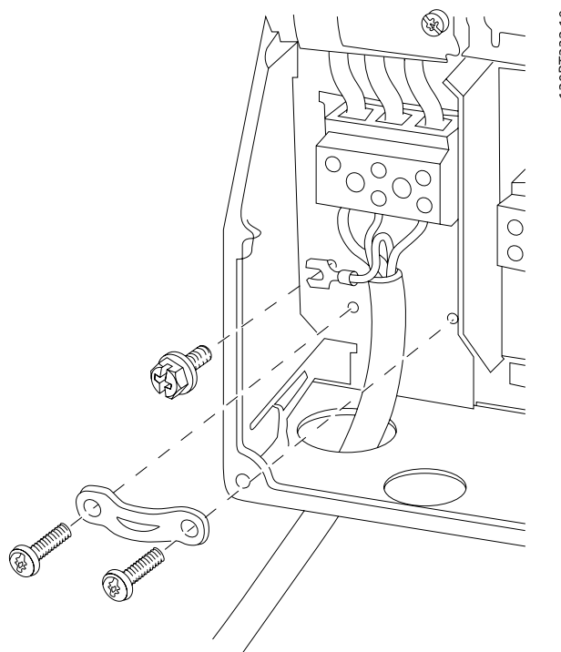
Kuva 4.9: Mallien B1 ja B2 kytkeminen verkkovirtaan ja maadoitukseen
