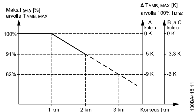
Kuva 9.1: Lähtövirran redusointi suhteessa korkeuteen lämpötilassa T AMB, MAX runkoko'ille A, B ja C. Kun korkeus on yli 2 km, ota yhteyttä Danfoss-yhtiöön keskustellaksesi PELV-jännitteestä.
