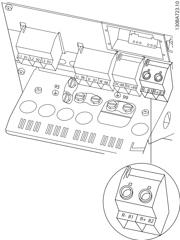
Kuva 4.25: Jarruliitosliitin malliin B4.
