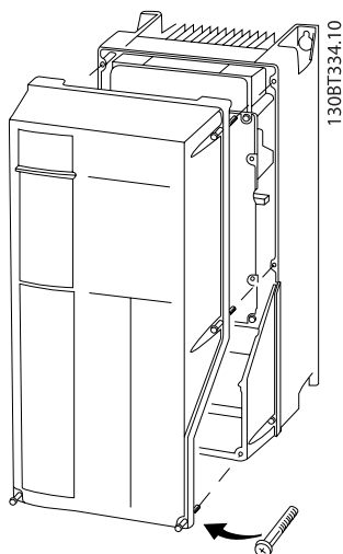
Kuva 4.33: A4-, A5-, B1-, B2-, C1- ja C2-kotelointien ohjausliitinten käyttömahdollisuus
