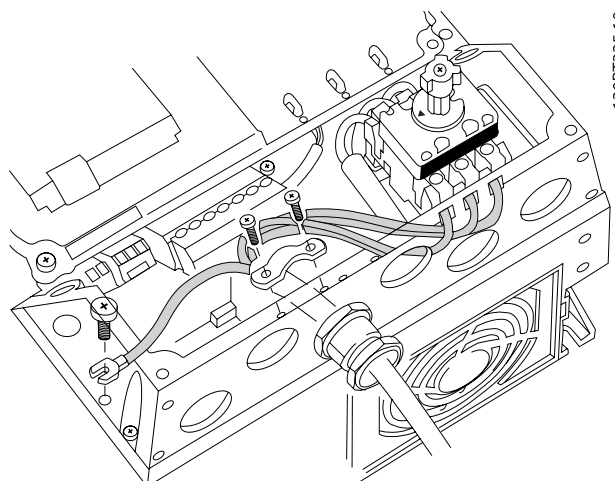
Kuva 4.8: Kytkeminen verkkovirtaan ja maadoitukseen katkaisimen avulla.
