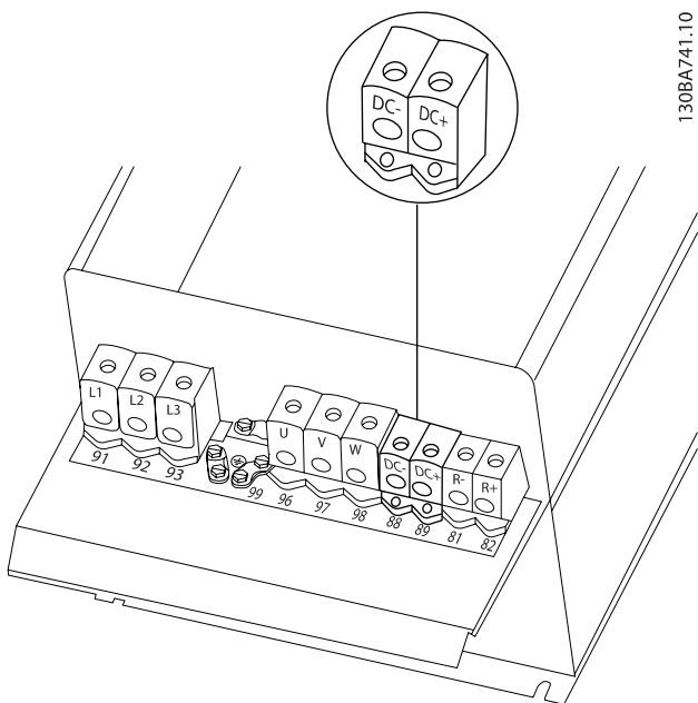
Kuva 4.23: Tasavirtaväyläyhteudet koteloon C4.
