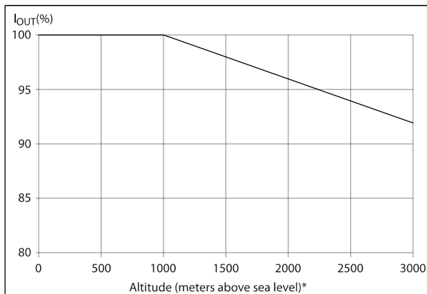
Lähtövirran redusointi suhteessa korkeuteen lämpötilassa T AMB, MAX runkoko'ille D, E ja F.
