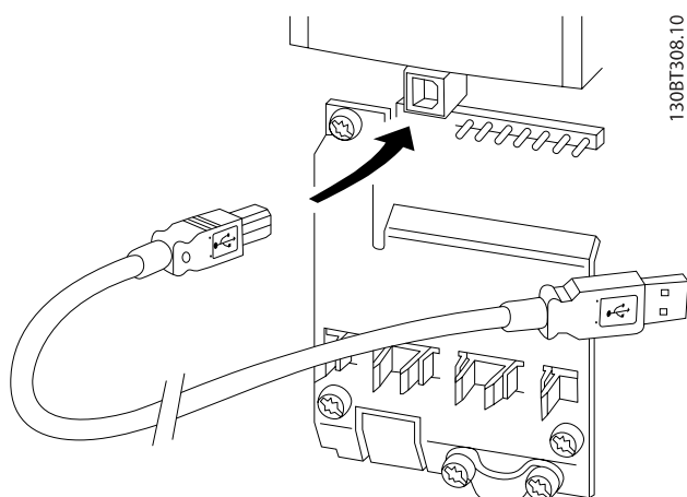
Kuva 5.3: Latso ohjaukskaapelin liitännät jaksosta Ohjausliittimet .
