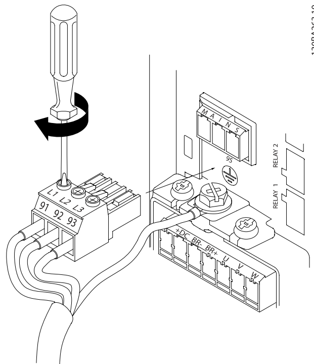
Kuva 4.5: Asenna sitten verkkovirtapistoke ja kiristä johtimet.
