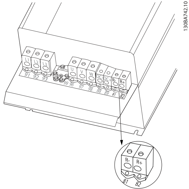
Kuva 4.27: Jarruliitosliitin malliin C4.
