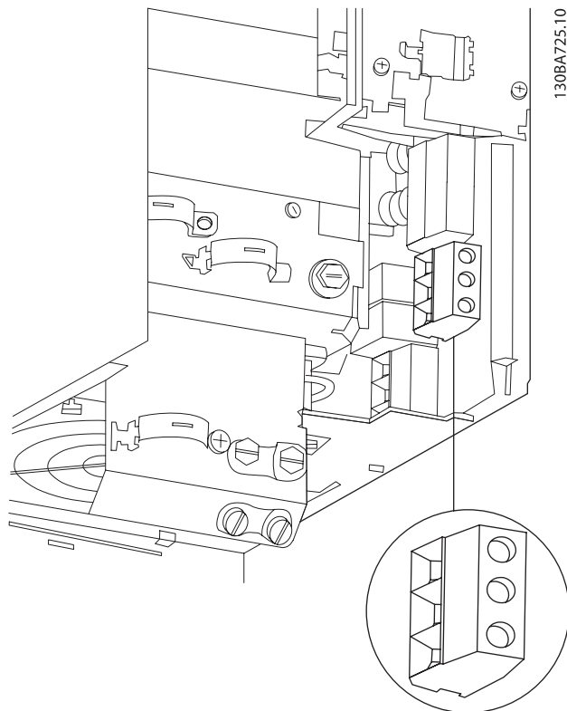
Kuva 4.10: Verkkovirran ja maadoituksen kytkeminen B3-malliin ilman RFI-suodatinta.
