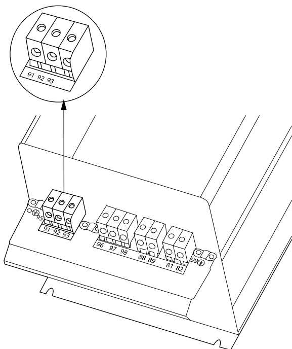
Kuva 4.14: C3 verkkovirtaan ja maadoitukseen.
