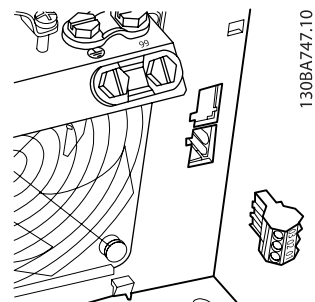
Kuva 4.29: Releiliitäntöihin tarvittavat liittimet B3-koteloon. Tehtaalla asennetaan valmiiksi vain yksi reletulo. Kun tarvitaan toinen rele, poista ejektori.
