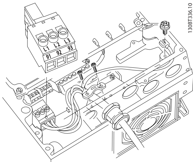
Kuva 4.7: Kytkeminen verkkovirtaan ja maadoitus ilman verkkovirran katkaisinta. Huomaa, että tässä käytetään kaapelin vedonpoistinta.
