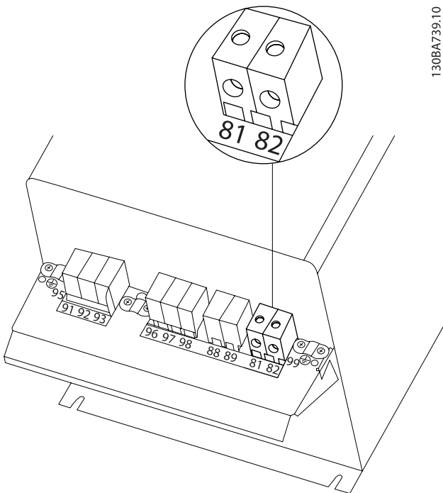
Kuva 4.26: Jarruliitosliitin malliin C3.
