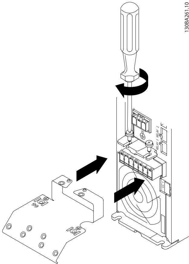
Kuva 4.3: Kiinnitä ensin molemmat ruuvit asennusaluistaan, työnnä se paikalleen ja kiristä kokonaan.
