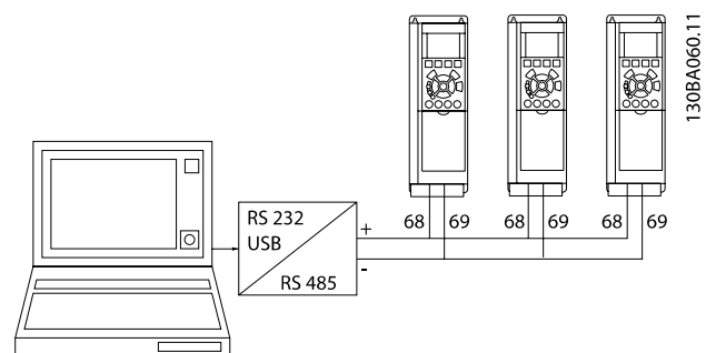
Kuva 5.2: Kytkentäesimerkki.
