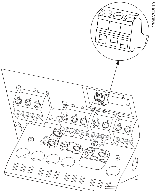
Kuva 4.30: Releliitäntöihin tarvittavat liittimet B4-koteloon.
