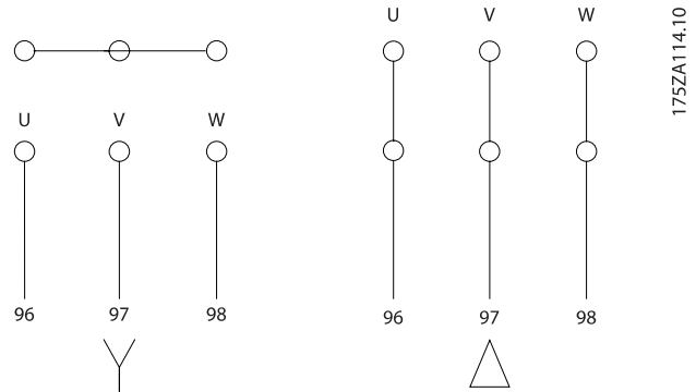
Kuva 4.16: Moottorin kytkennässä käytettävät liittimet
