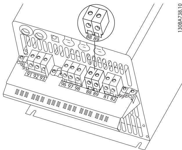
Kuva 4.22: Tasavirtaväyläyhteiset koteloon C3.
