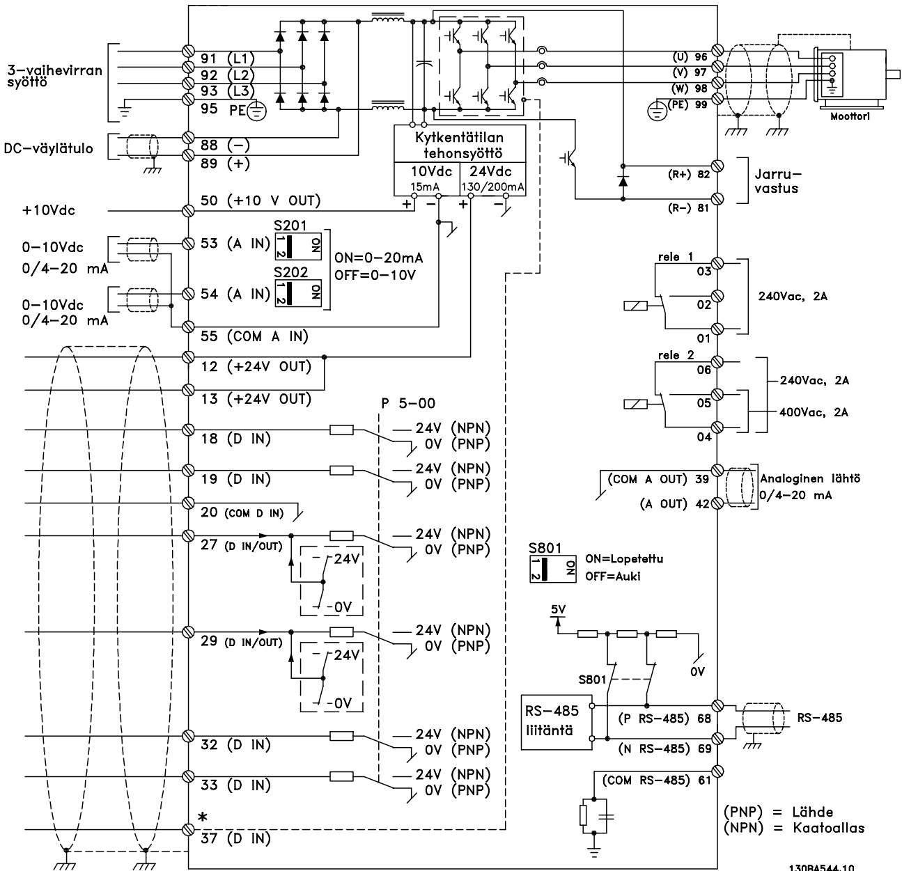
Kuva 4.1: Kaavio, jossa näkyvät kaikki sähköliittimet. (Liitin 37 vain laitteissa, joissa on turvapäätystoiminto.)
