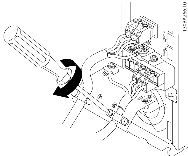
Kuva 4.18: Kiinnitä kaapelin vedonpoistin varmistaaksesi 360 asteen liittännän alustan ja suojausken välillä. Varmista, että moottorikaapelin ulommainen eristys on poistettu vedonpoistimen alta.
