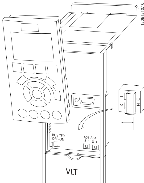
Εικόνα 4.44: Θέση διακοπών.
