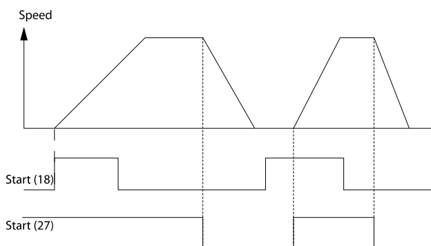
Εικόνα 5.5: Ακροδέκτης 37: Διατίθεται μόνο με λειτουργία ασφαλούς διακοπής!
