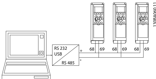
Εικόνα 5.2: Παράδειγμα σύνδεσης.
