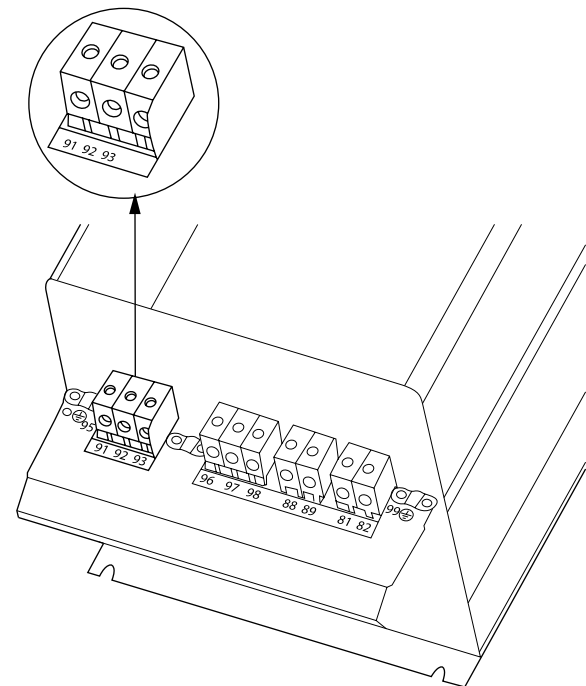
Εικόνα 4.14: Τρόπος σύνδεσης του C3 στο δίκτυο ρεύματος και στη γείωση.
