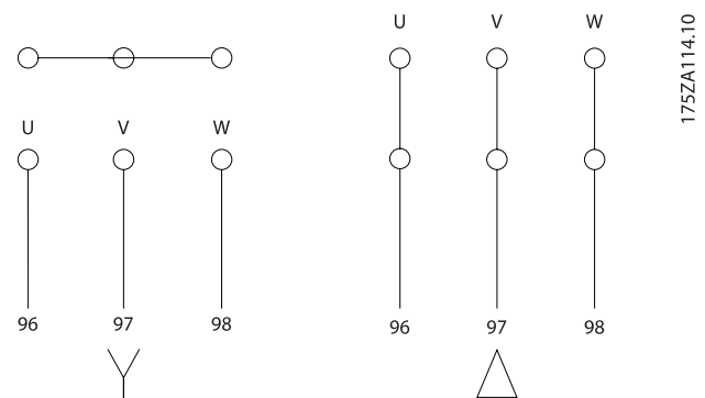
Εικόνα 4.16: Ακροδέκτες για σύνδεση κινητήρα
