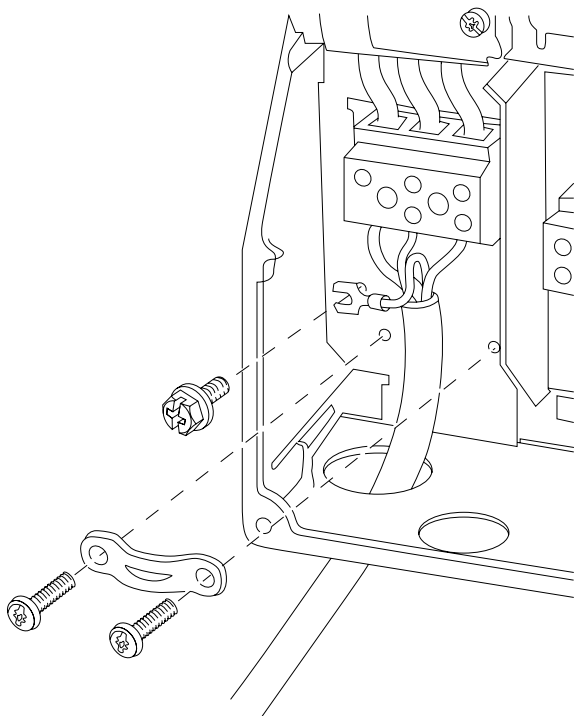
Εικόνα 4.9: Σύνδεση με το δίκτυο ρεύματος και γείωση για B1 και B2
