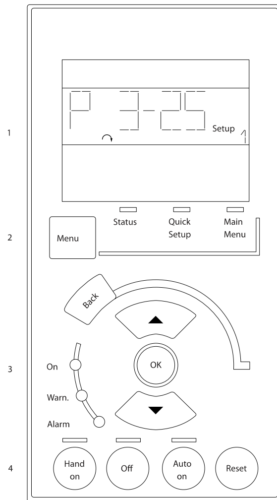
Εικόνα 6.1: Αριθμητικό LCP (NLCP)
