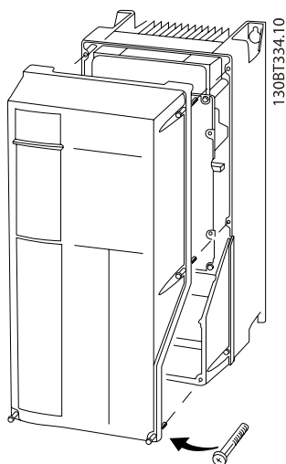
Εικόνα 4.33: Πρόσβαση στους ακροδέκτες σημάτων ελέγχου για τα περιβλήματα A4, A5, B1, B2, C1 και C2
