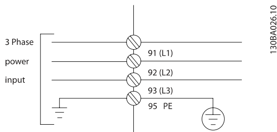
Εικόνα 4.2: Ακροδέκτες για δίκτυο ρεύματος και γείωση.
