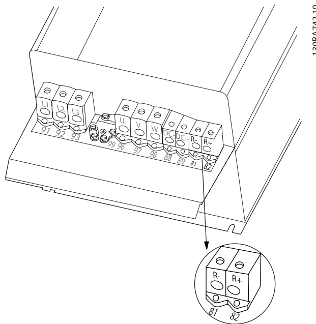
Εικόνα 4.27: Ακροδέκτης σύνδεσης πέδης για μέγεθος μονάδας 34.
