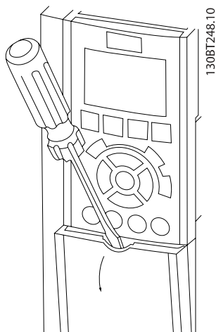
Εικόνα 4.32: Πρόσβαση στους ακροδέκτες σημάτων ελέγχου για τα περιβλήματα A2, A3, B3, B4, C3 και C4
