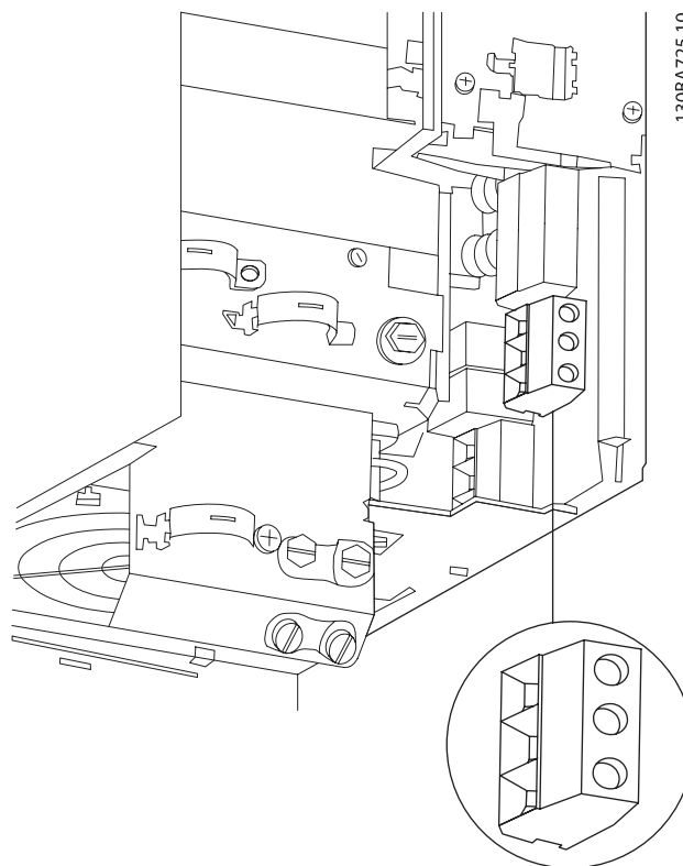
Εικόνα 4.10: Τρόπος σύνδεσης σε δίκτυο ρεύματος και γείωση για B3 χωρίς RFI.
