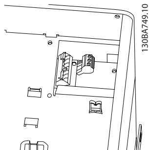
Εικόνα 4.31: Ακροδέκτες για συνδέσεις ρελέ για C3 και C4. Βρίσκονται στην άνω δεξιά γωνία του μετατροπέα συχνότητας.
