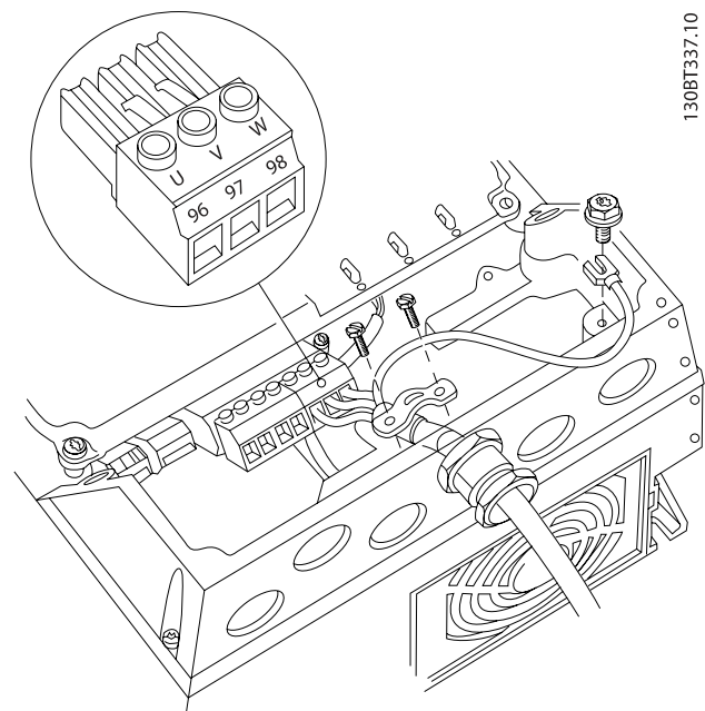
Εικόνα 4.19: Πρώτα συνδέστε τη γείωση, στη συνέχεια τοποθετήστε τα καλώδια U, V και W του κινητήρα στον ακροδέκτη και βιδώστε τα. Βεβαιωθείτε ότι η εξωτερική μόνωση του καλωδίου κινητήρα έχει αφαιρεθεί κάτω από το σφιγκτήρα EMC.
