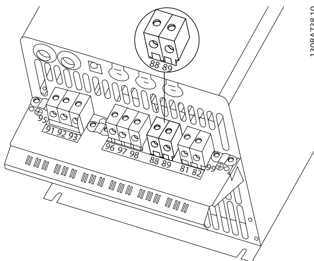
Εικόνα 4.22: Συνδέσεις διαύλου DC για περίβλημα C3.
