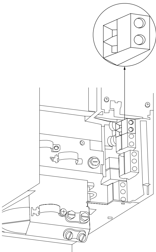
Εικόνα 4.20: Συνδέσεις διαύλου DC για περίβλημα B3.
