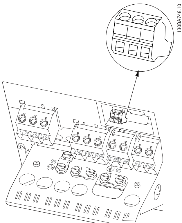
Εικόνα 4.30: Ακροδέκτες για συνδέσεις ρελέ για Β4.
