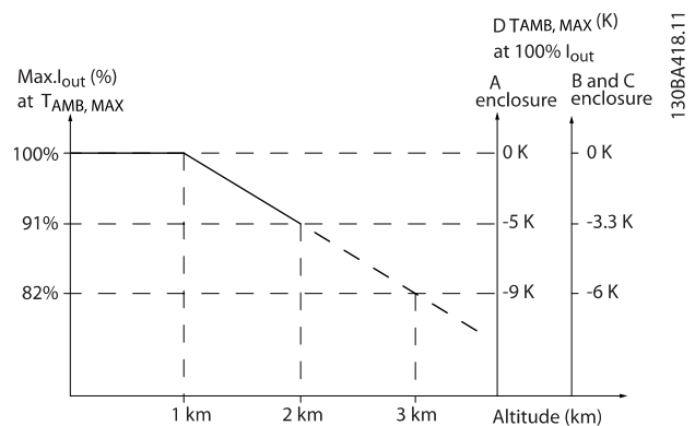
Εικόνα 9.1: Ο υποβιβασμός του ρεύματος εξόδου έναντι του υψόμετρου σε T_{AMB, MAX} for μεγέθη πλαισίου A, B και C. Σε υψόμετρα που ξεπερνούν τα 2 χλμ., επικοινωνήστε με την Danfoss για την πολύ χαμηλή τάση προστασίας PELV.
