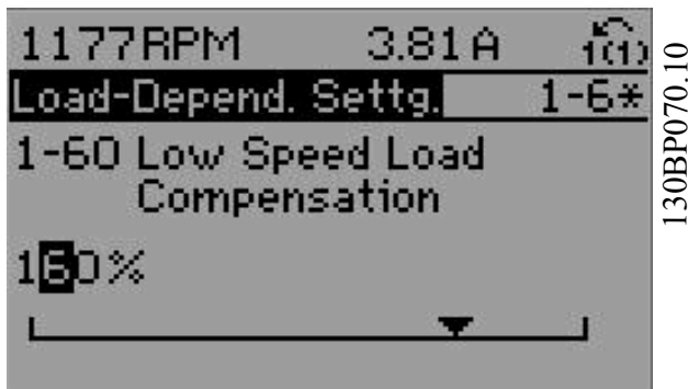
Εικόνα 7.11: Παράδειγμα οθόνης.
