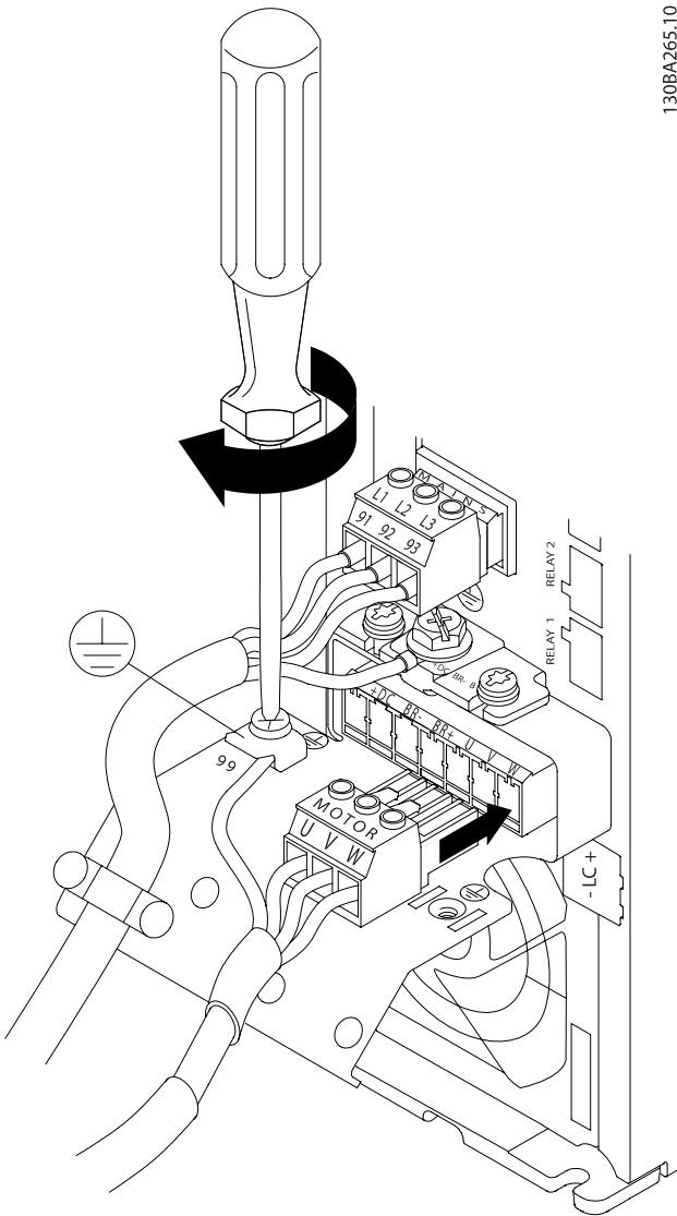
Εικόνα 4.17: Πρώτα συνδέστε τη γείωση, στη συνέχεια τοποθετήστε τα καλώδια U, V και W του κινητήρα στο βύσμα και βιδώστε τα.
