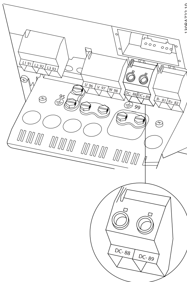
Εικόνα 4.21: Συνδέσεις διαύλου DC για περίβλημα B4.
