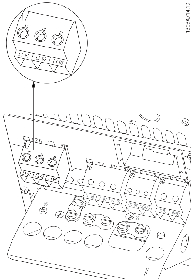
Εικόνα 4.12: Τρόπος σύνδεσης στο δίκτυο ρεύματος και στη γείωση για Β4.
