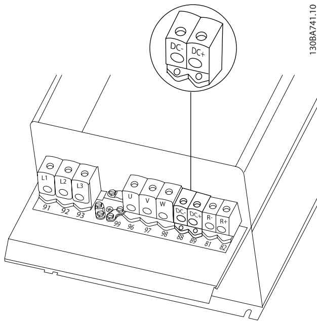
Εικόνα 4.23: Συνδέσεις διαύλου DC για περίβλημα C4.
