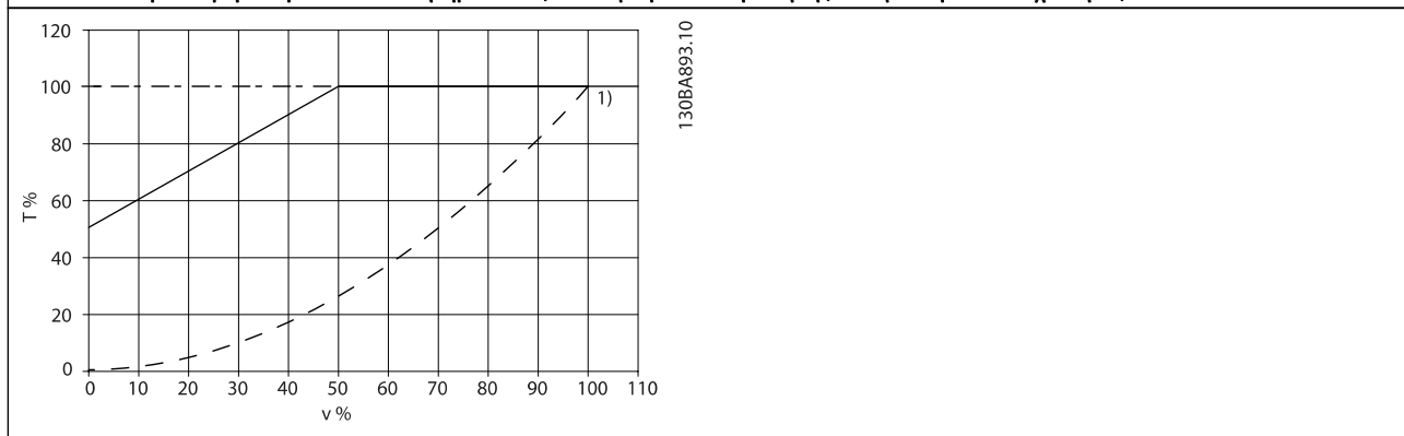
Μέγιστο φορτίο για τυπικό κινητήρα στους 40 °C με μετάδοση κίνησης από μετατροπέα συχνότητας τύπου VLT FCxxx
