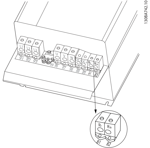
Çizim 4.27: C4 için fren bağlantı terminali.
