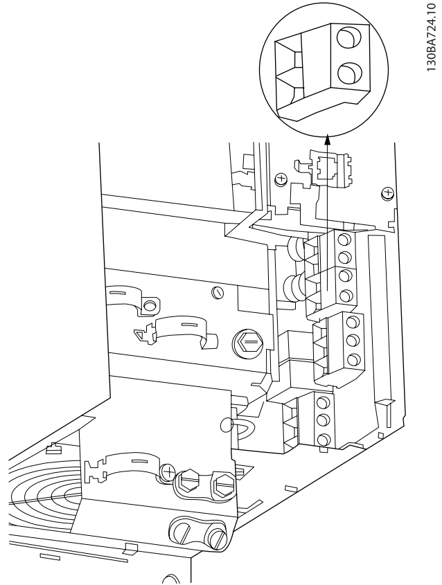
Çizim 4.24: B3için fren bağlantı terminali.
