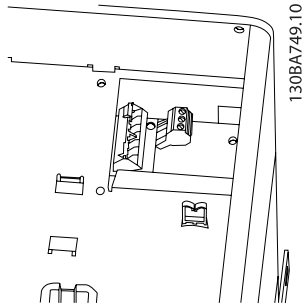
Çizim 4.31: C3 ve C4 için röle bağlantıları terminalleri. Frekans dönüştürücünün sağ üst köşesinde bulunur.
