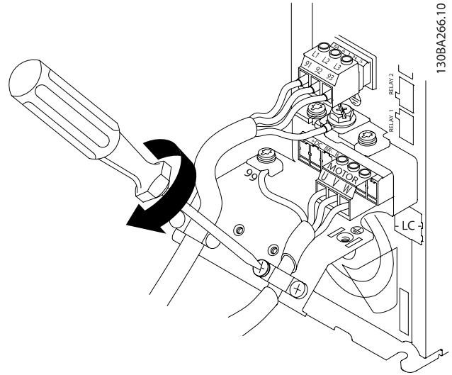
Çizim 4.18: Şasi ile ekran arasında 360 derecelik bağlantı sağlamak için kablo kelepçesini takın, motor kablosunun dış izolasyonunun kelepçenin altından çıkmasına dikkat edin.
