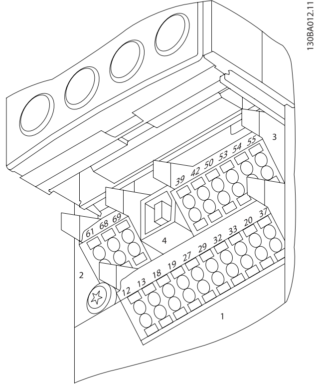
Çizim 4.34: Kontrol terminalleri (tüm muhafazalar)
