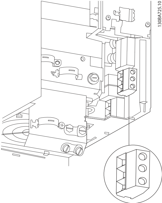
Çizim 4.10: RFI olmadan B3 için şebekeye ve topraklamaya bağlama.
