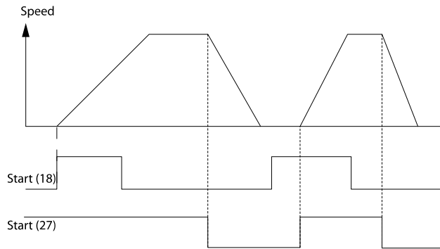
Çizim 5.5: Terminal 37 Yalnızca Güvenli Durdurma İşlevi'nde kullanılabilir!
