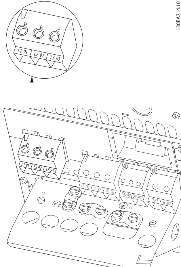
Çizim 4.12: B4 için şebekeye ve topraklamaya bağlama.
