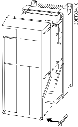
Çizim 4.33: A4, A5, B1, B2, C1 ve C2 muhafazalarının
