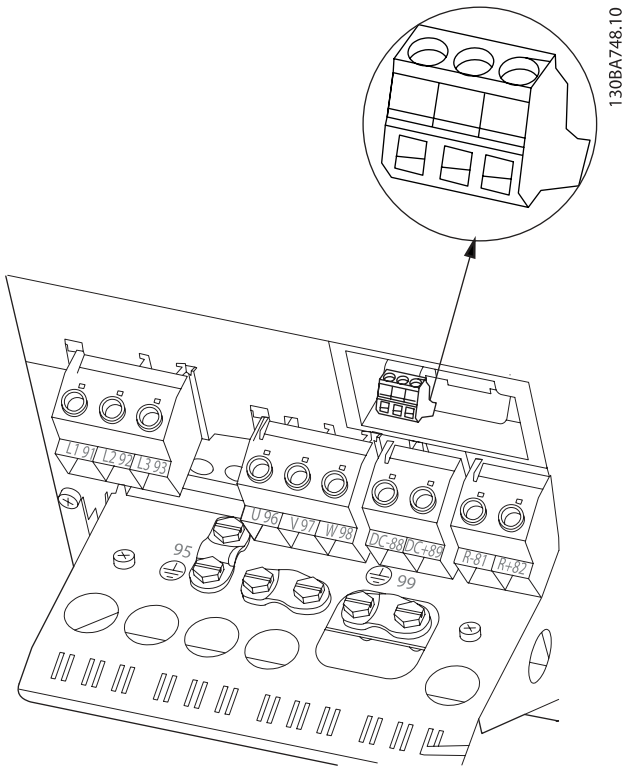
Çizim 4.30: B4 röle bağlantıları için terminaller.
