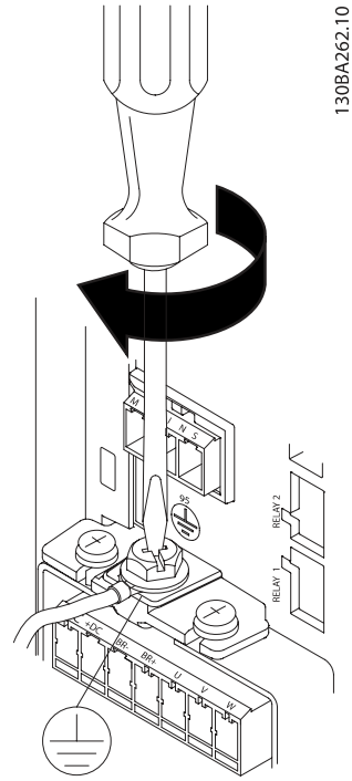
Çizim 4.4: Kabloları monte ederken, öncelikle toprak kablosunu takın ve sıkıştırın.
