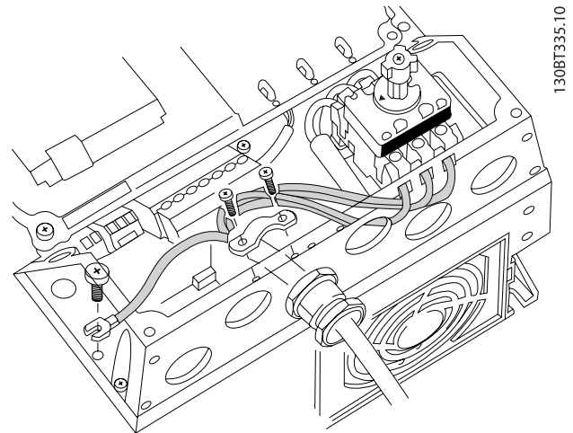
Çizim 4.8: Şebeke ayırma anahtarıyla şebekeyi ve topraklamayı bağlama.
