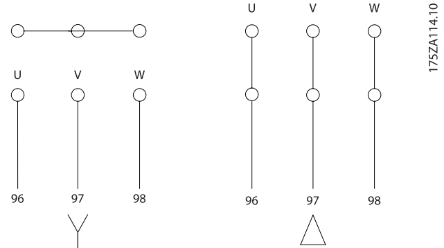
Çizim 4.16: Motor bağlantısı için terminaller
