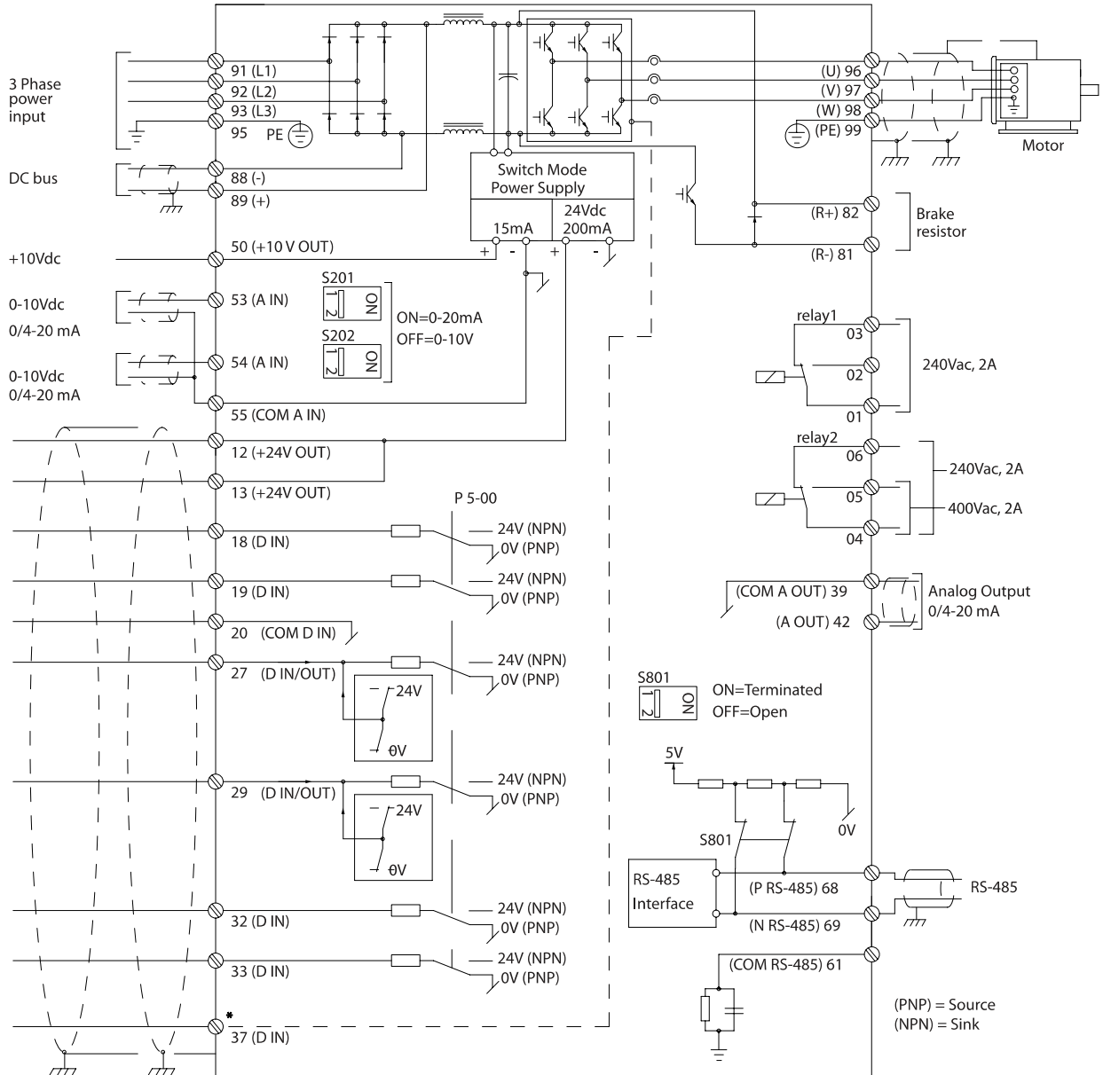
Çizim 4.1: Tüm elektrik terminallerini gösteren diyagram. (Terminal 37 yalnızca Güvenli Durdurma İşlevine sahip birimlerde mevcuttur.)
