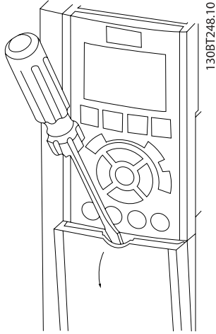
Çizim 4.32: A2, A3, B3, B4, C3 ve C4 muhafazalarının kontrol terminallerine erişim
