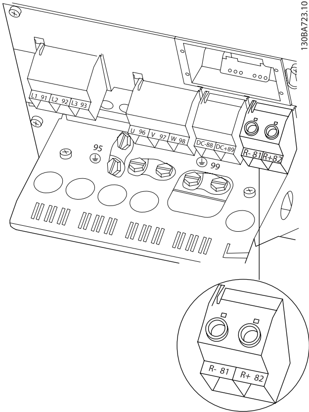
Çizim 4.25: B4 için fren bağlantı terminali.
