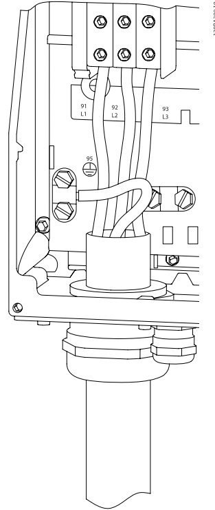
Çizim 4.13: C1 ve C2 için şebekeye ve topraklamaya bağlama.
