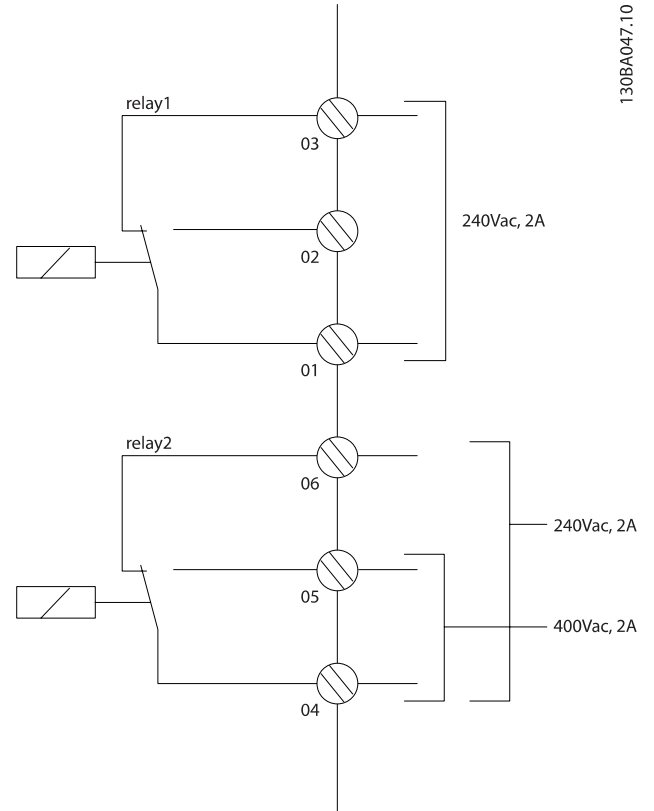
Çizim 4.31: C3 ve C4 için röle bağlantıları terminalleri. Frekans dönüştürücünün sağ üst köşesinde bulunur.
