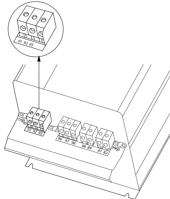
Çizim 4.14: C3'ü şebekeye ve toprağa bağlama.
