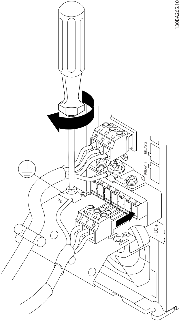
Çizim 4.17: Öncelikle motor topraklamasını uçlandırın, ardından motorun U, V ve W tellerini fişe takıp sıkıştırın.
