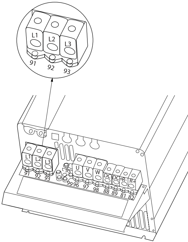
Çizim 4.15: C4'ü şebekeye ve toprağa bağlama.
