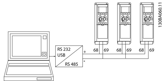
Çizim 5.2: Bağlantı örneği.
