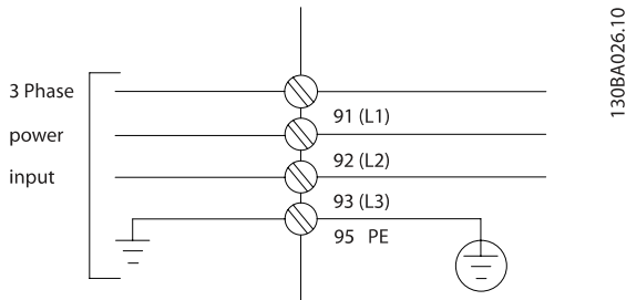
Çizim 4.2: Şebeke ve topraklama terminaleri.
