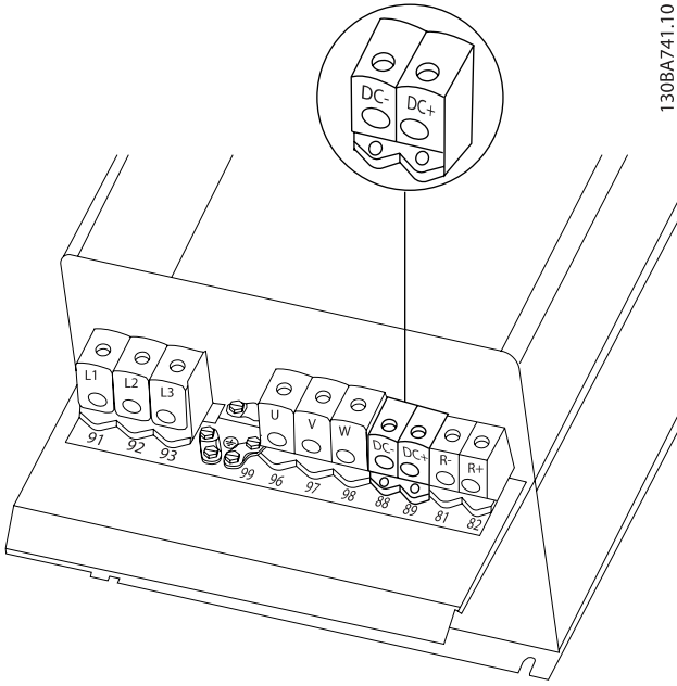
Çizim 4.23: C4 muhafazası.
