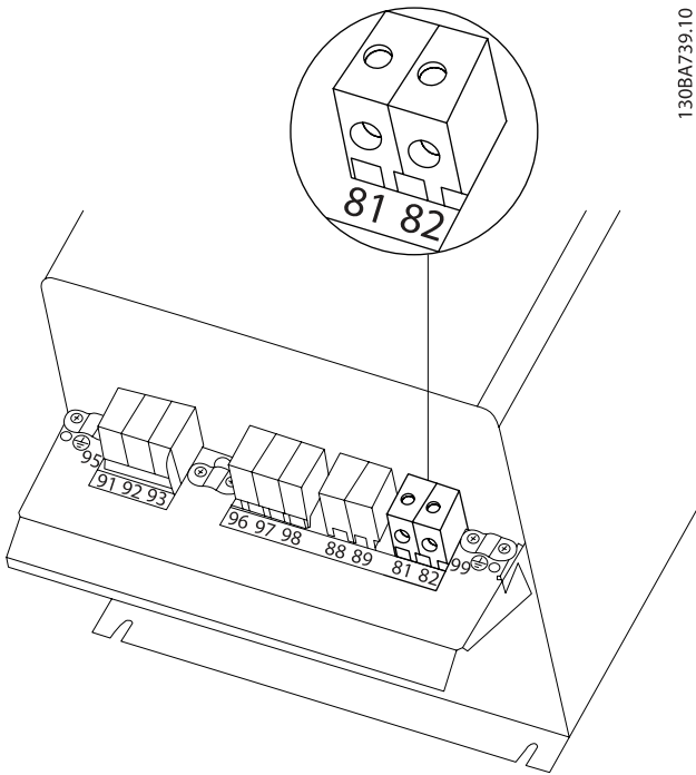
Çizim 4.26: C3 için fren bağlantı terminali.
