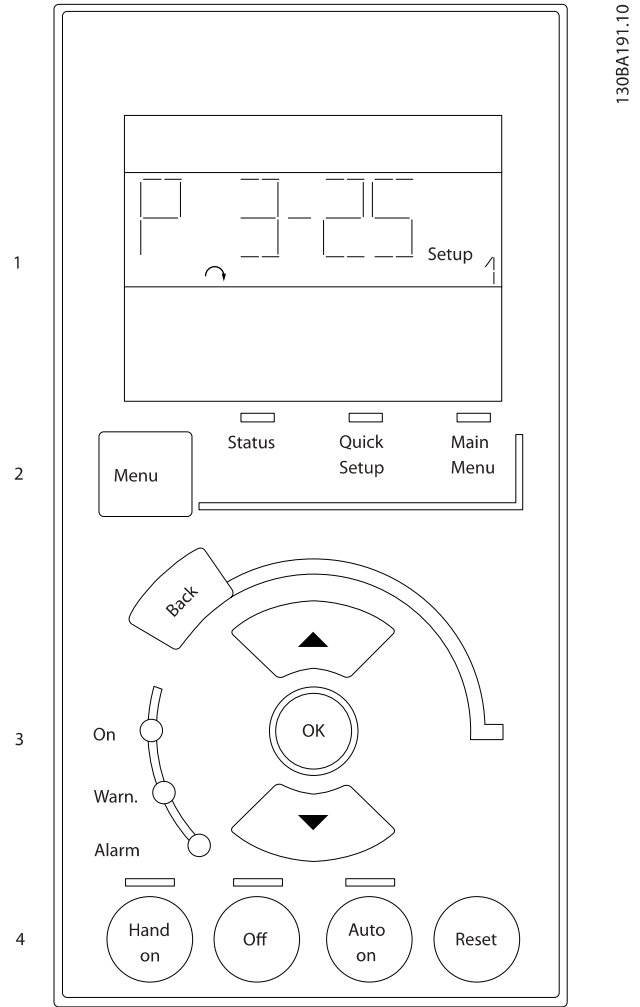
Çizim 6.1: Sayısal LCP (NLCP)
