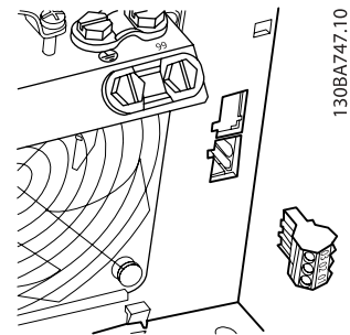
Çizim 4.29: B3 röle bağlantıları için terminaller. Fabrikada yalnızca tek bir röle girişi takılır. İkinci röle gerekirse, takma kapağını çıkarın.
