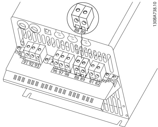
Çizim 4.22: C3 muhafazası için DC bus bağlantıları.
