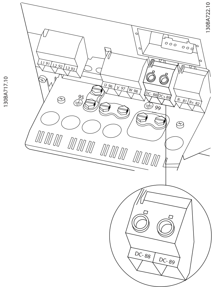
Çizim 4.21: B4 muhafazası için DC bus bağlantıları.
