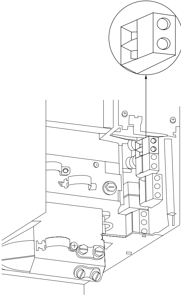
Çizim 4.20: B3 muhafazası için DC bus bağlantıları.
