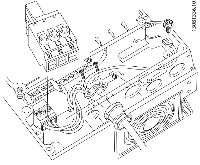
Çizim 4.7: Şebeke ayırma anahtarı olmaksızın şebekeyi ve topraklamayı bağlama. Kablo kelepçesinin kullanıldığını unutmayın.
