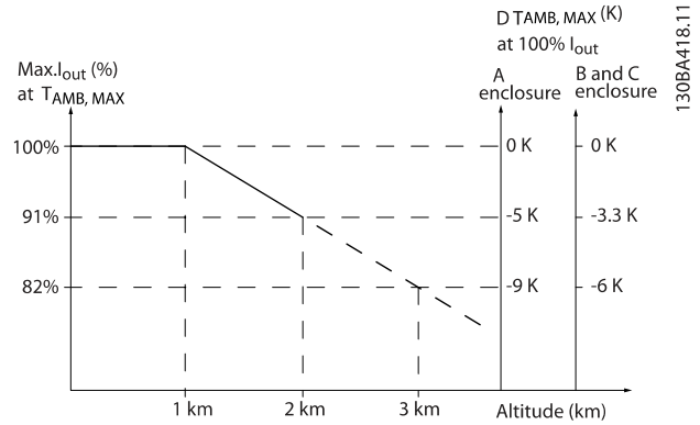
Çizim 9.1: A, B ve C çerçeve boyutu 1x, 2x ve 3x . Denizden 2 km'den daha yüksek yerlerde, DanfossPELV ile ilgili lütfen ile iribat kurun.
