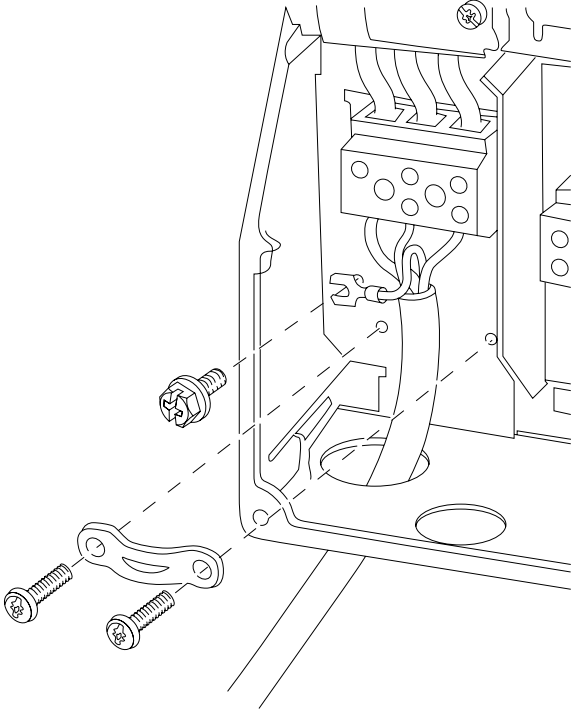
Çizim 4.9: B1 ve B2 için şebekeye ve topraklamaya bağlama
