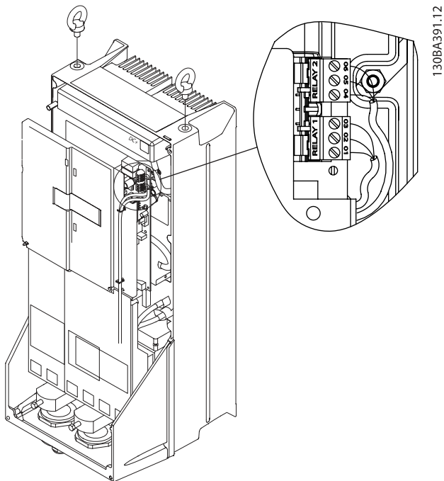
Çizim 4.28: Röle bağlantısı için terminaller (C1 ve C2 muhafazaları).
