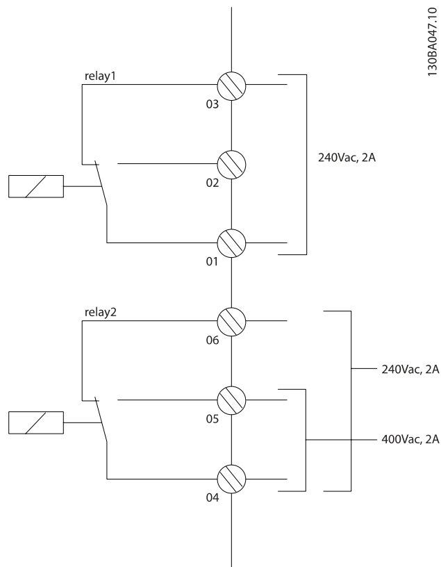
圖 4.31: C3 與 C4 的繼電器連接端子。位於變頻器的右上角。
