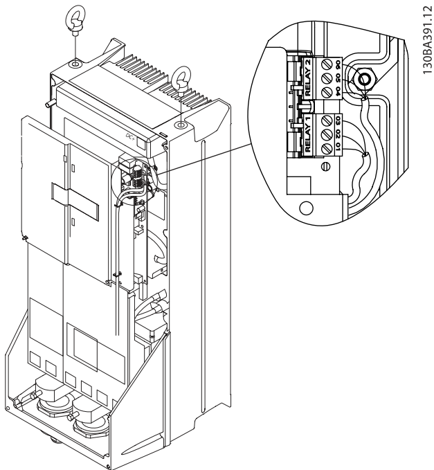
圖 4.28: 繼電器連接端子 (C1 與 C2 外殼)。 繼電器連接係顯示於已裝上繼電器插頭 (從配件包取出的) 的放大圖。
