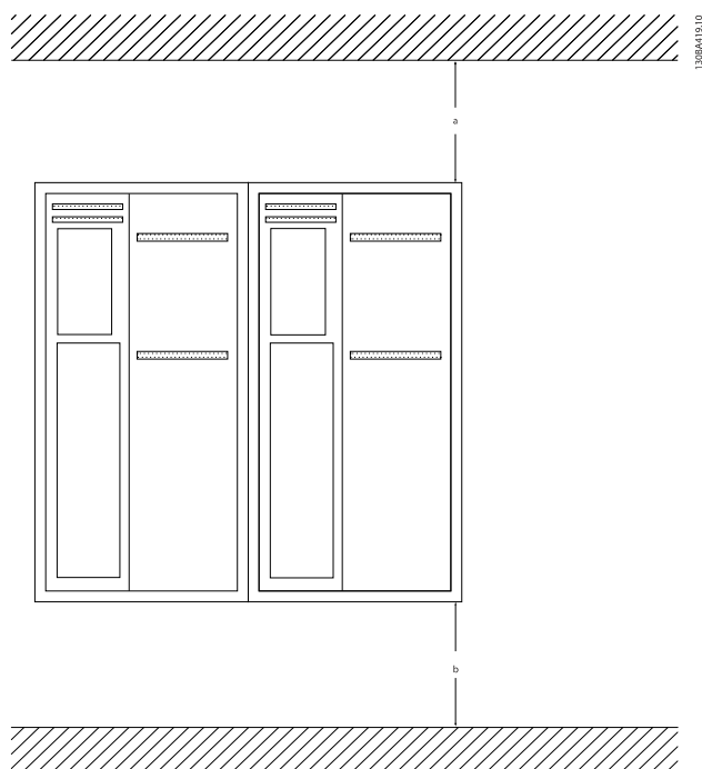
不同外殼的通風空間
