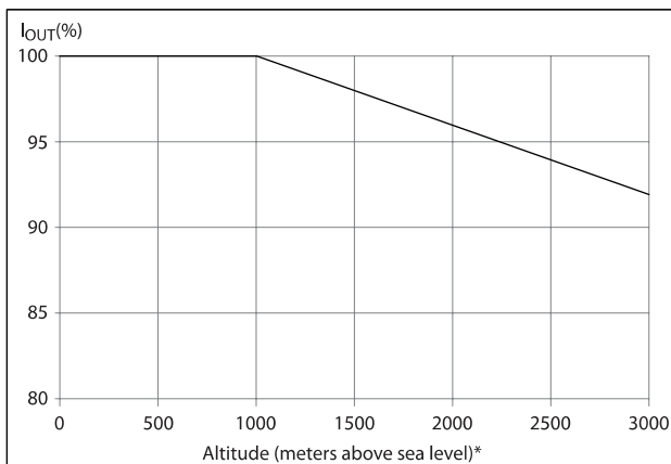
機架大小 D、E 和 F 在 T_{AMB, MAX} 時，輸出電流額定值的降低與海拔高度的關係。
