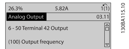
圖 7.6: 步驟 6: 選擇參數 6-50。按下 [OK]。
