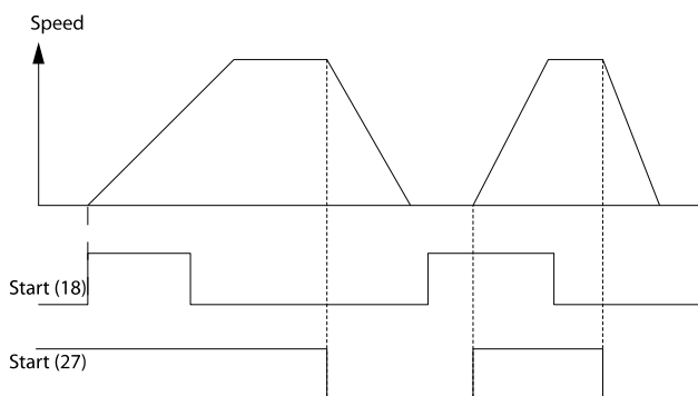
圖 5.5: 端子 37: 僅在具有安全停機功能時提供!
