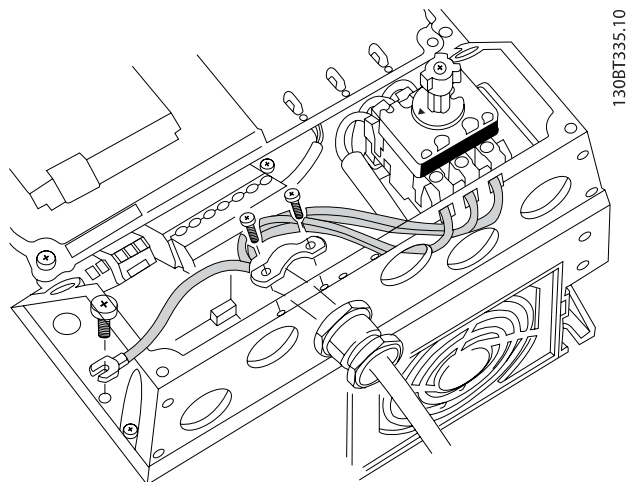
圖 4.8: 如何使用主電源斷開連接開關連接至主電源與接地。
