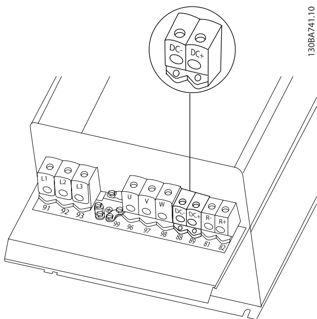
圖 4.23: 外殼 C4 DC 總線的連接。
