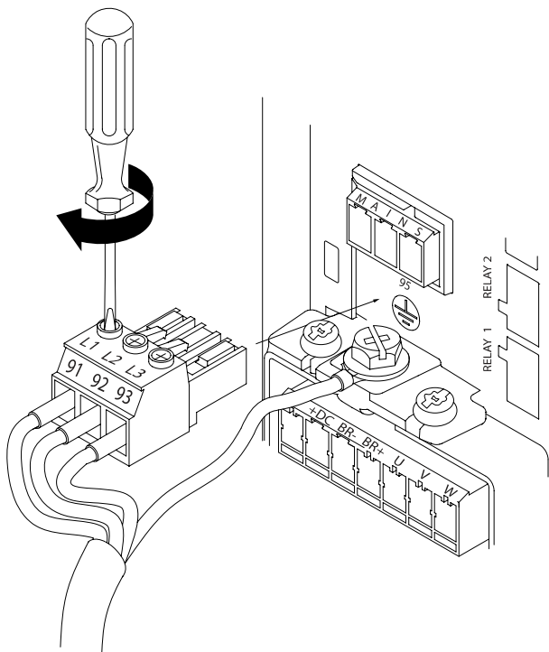
圖 4.5: 然後安裝主電源插頭並鎖緊電線。
