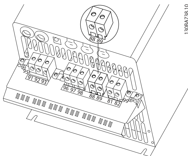
圖 4.22: 外殼 C3 DC 總線的連接。
