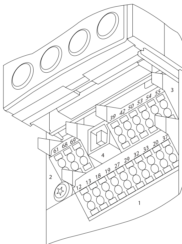
圖 4.34: 控制端子 (所有外殼)
