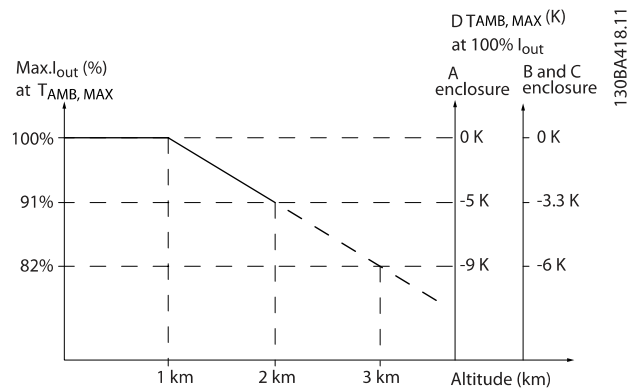
圖 9.1: 機架大小 A、B 和 C 在 T_{AMB, MAX} 時，輸出電流額定值的降低與海拔高度的關係。海拔高度超過 2 km 時，請洽詢 Danfoss 瞭解有關 PELV 的資訊。
