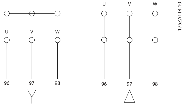
圖 4.16: 馬達連接的端子。
