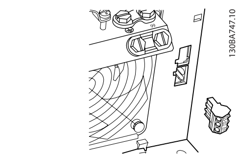
圖 4.29: B3 的繼電器連接端子。出廠時僅安裝一個繼電器輸入。在需要使用第二繼電器時移除擋板。
