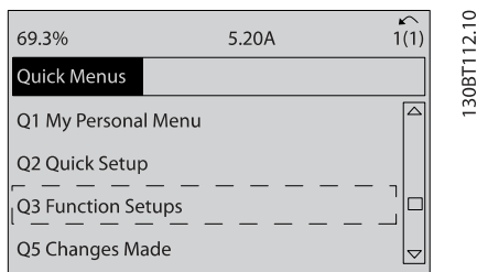
圖 7.3: 步驟 3: 使用向上/向下導航鍵下拉至功能設定表單。按下 [OK]。
