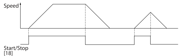
圖 5.4: 端子 37: 僅在具有安全停機功能時提供!
