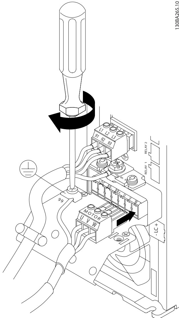
圖 4.17: 首先將馬達地線終接，然後將馬達 U、V 與 W 電線放進插頭並鎖緊。
