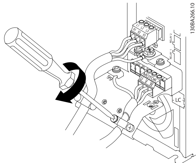
圖 4.18: 請安裝電纜線夾鉗以確保在底架與遮罩之間具有 360 度的連接，請注意，馬達電纜線的外部絕緣已從夾鉗下移除。
