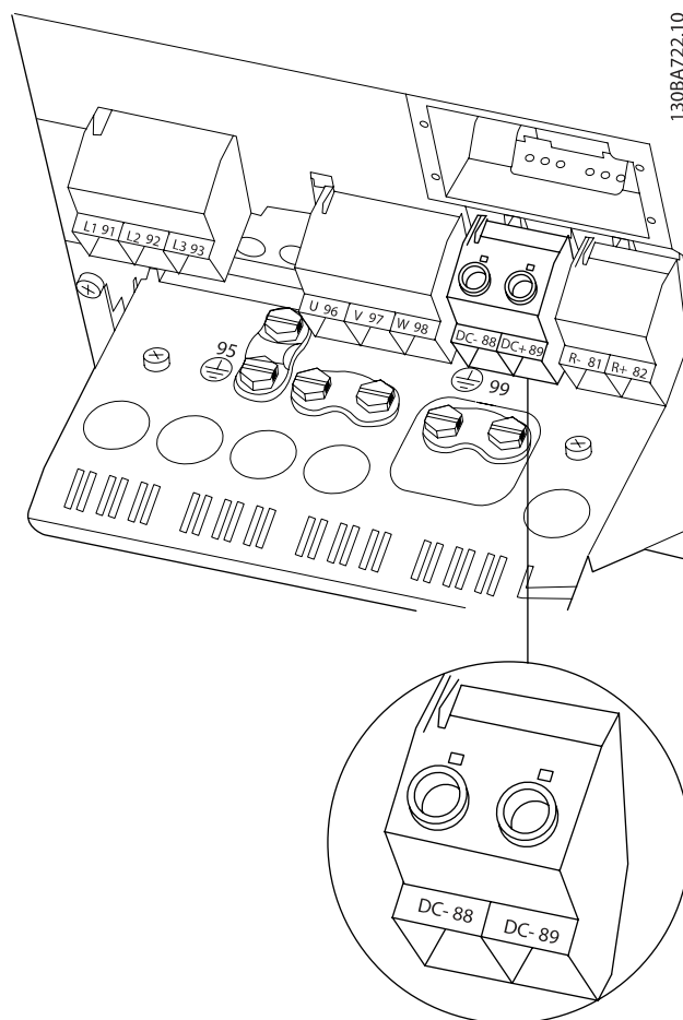
圖 4.21: 外殼 B4 DC 總線的連接。
