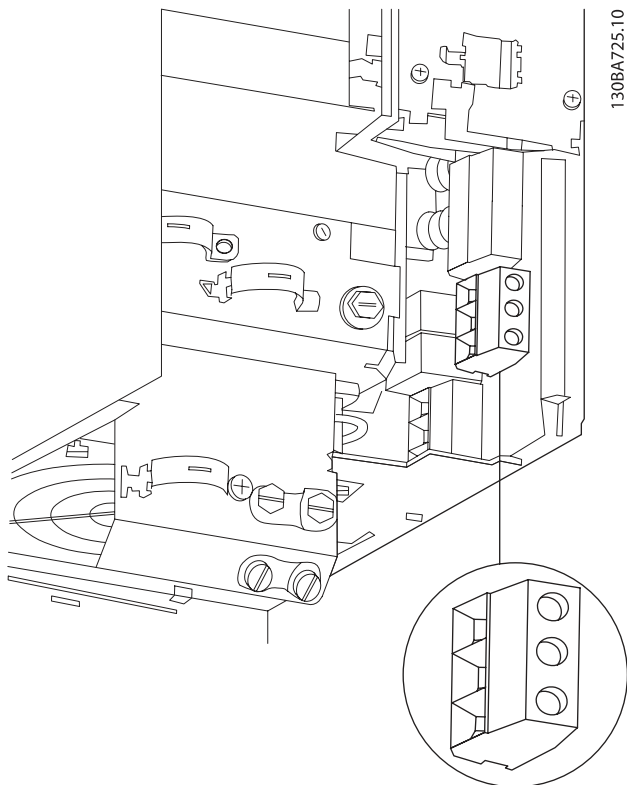
圖 4.10: 如何連接到主電源以及不含 RFI 的 B3 的接地。
