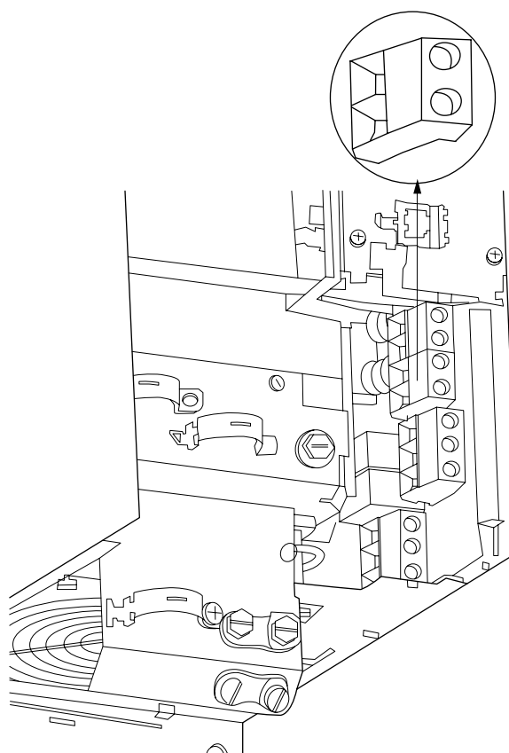
圖 4.24: B3 的煞車連接端子。
