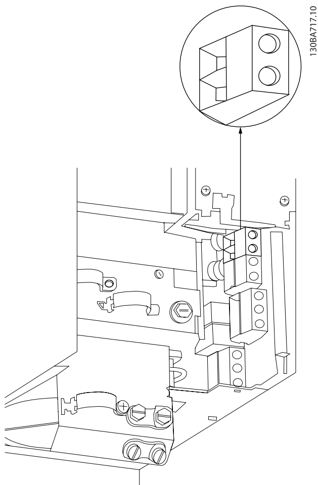
圖 4.20: 外殼 B3 DC 總線的連接。
