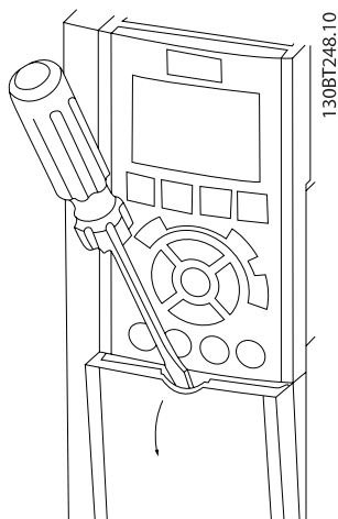
圖 4.32: 操作 A2、A3、B3、B4、C3 與 C4 外殼的控制端子
