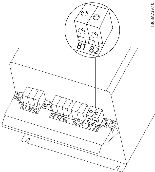
圖 4.26: C3 的煞車連接端子。
