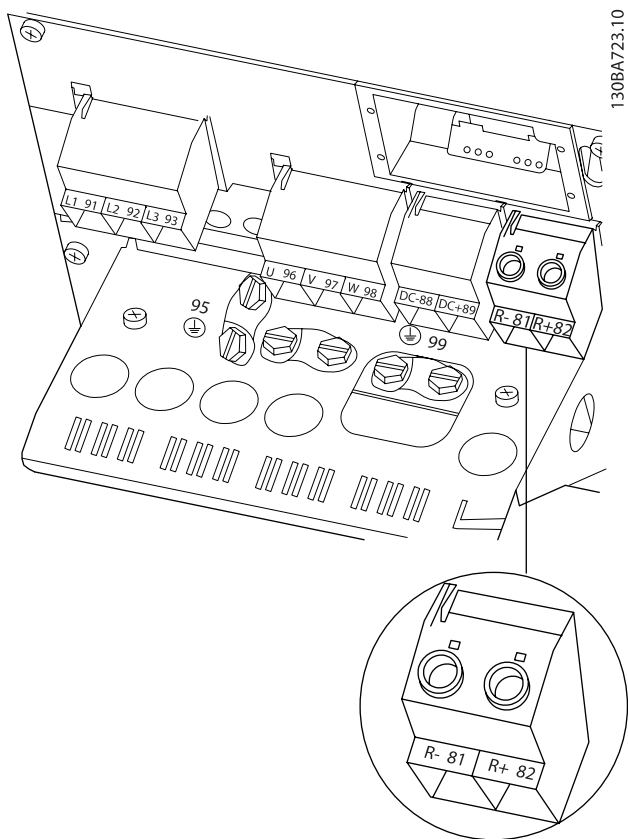
圖 4.25: B4 的煞車連接端子。
