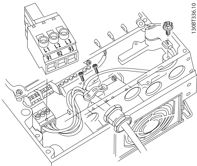
圖 4.7: 如何在不使用主電源斷開連接開關的情況下連接至主電源與接地。請注意此處使用了電纜線夾鉗。
