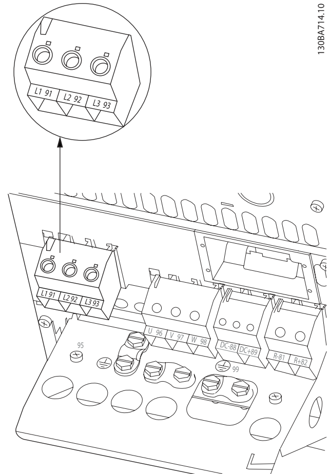
圖 4.12: 如何將 B4 連接至主電源與接地。
