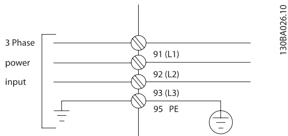
圖 4.2: 主電源和接地的端子。
