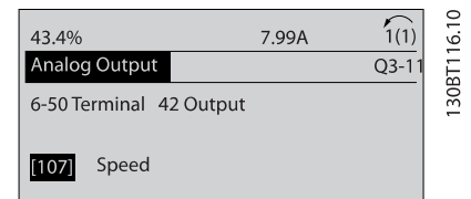
圖 7.7: 步驟 7: 使用向上/向下導航鍵在不同的選項之間進行選擇。按 [OK] 鍵。
