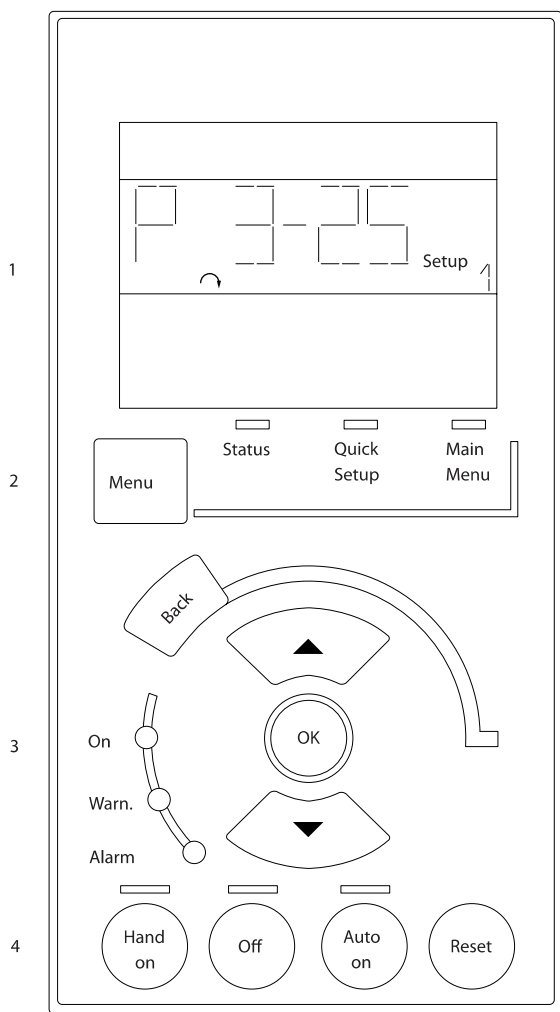
圖 6.1: 數字型 LCP (NLCP)
