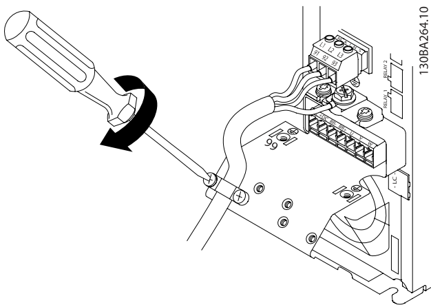
圖 4.6: 最後將支撐架鎖至主電源電線上。
