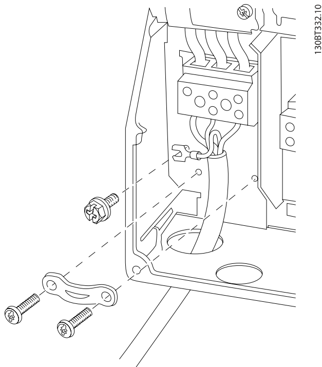
圖 4.9: 如何連接到主電源及接地 (B1 與 B2 )。
