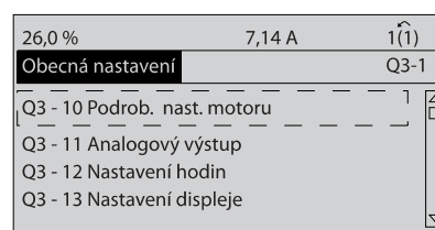
Obrázek 7.5: Krok 5: Pomocí navigačních tlačítek nahoru a dolů přejděte dolů např. na možnost Q3-11 Analogové výstupy. Stiskněte tlačítko [OK].
