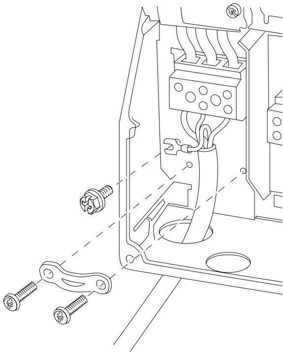
Obrázek 4.9: Připojení k síti a uzemnění pro B1 a B2
