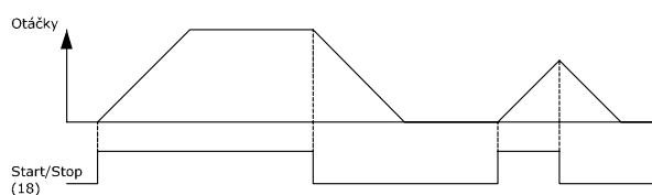
Obrázek 5.4: Svorka 37: K dispozici pouze s funkcí bezpečného zastavení!
