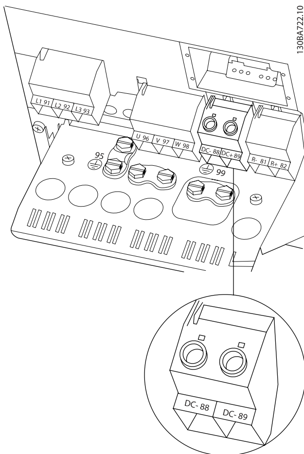
Obrázek 4.21: Připojení sběrnice DC pro krytí B4.
