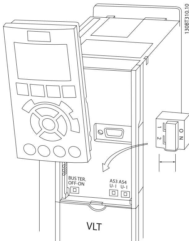
Obrázek 4.44: Umístění přepínačů.
