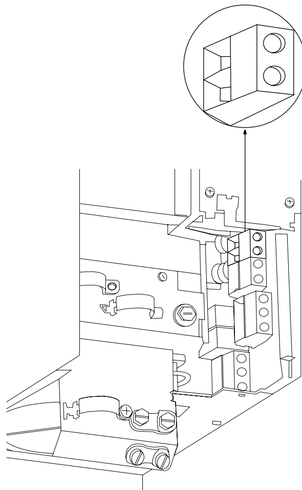
Obrázek 4.20: Připojení sběrnice DC pro krytí B3.
