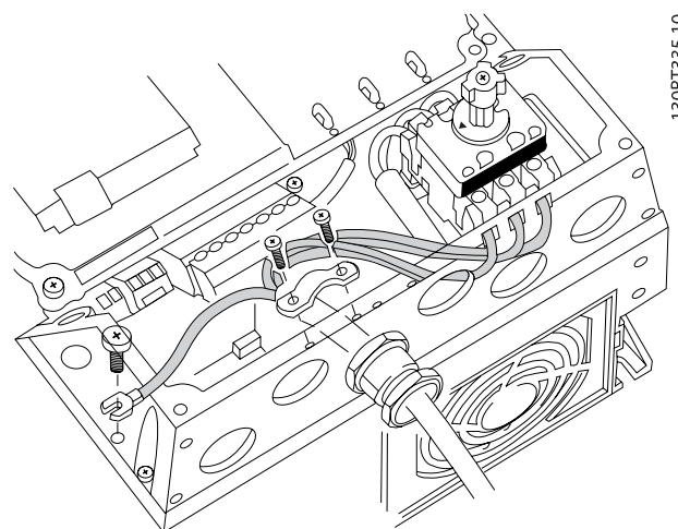
Obrázek 4.8: Připojení k síti a uzemnění s odpojovačem.
