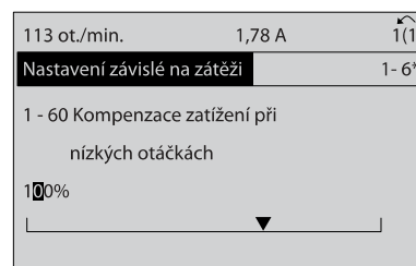
Obrázek 7.10: Příklad zobrazení na displeji.
