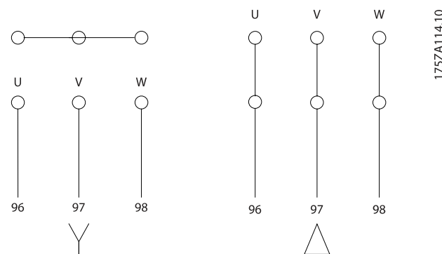
Obrázek 4.16: Svorky pro připojení motoru
