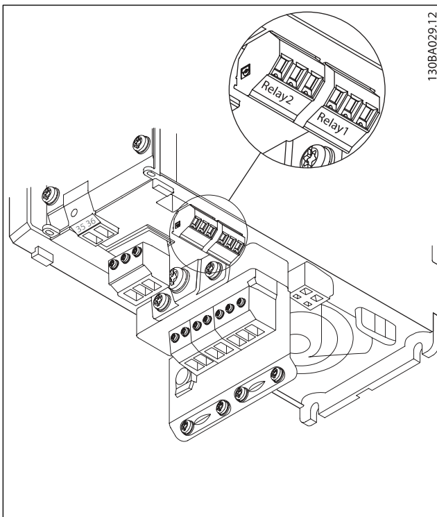
Svorky pro připojení relé (krytí A2 a A3).
