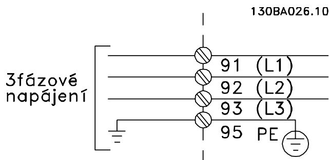
Obrázek 4.2: Svorky síťového napájení a uzemnění.
