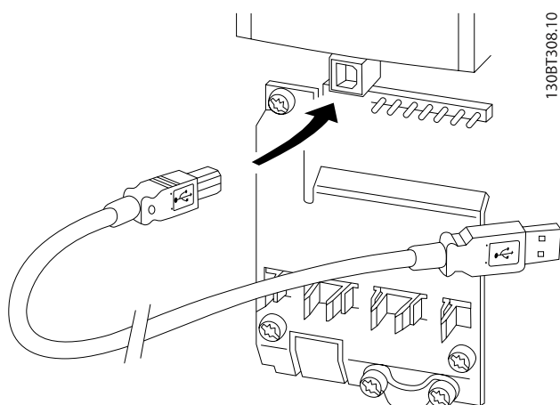
Obrázek 5.3: Další informace o připojení řídicích kabelů najdete v části Řídicí svorky.
