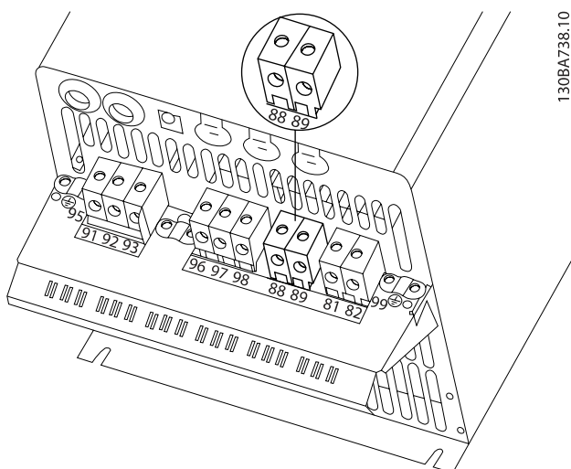
Obrázek 4.22: Připojení sběrnice DC pro krytí C3.
