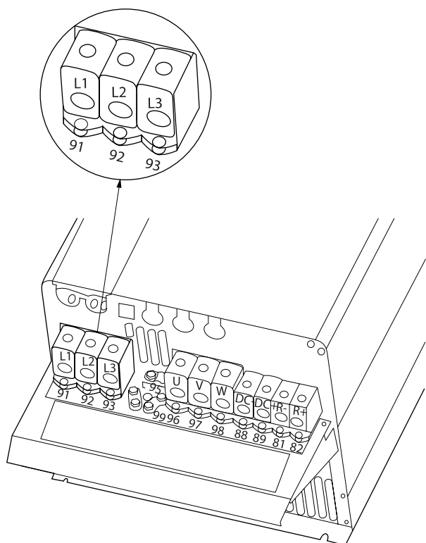
Obrázek 4.15: Připojení C4 k síti a uzemnění.
