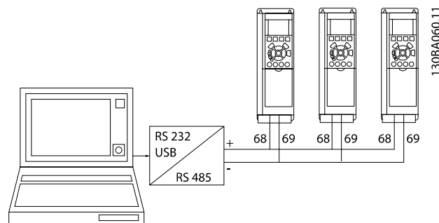
Obrázek 5.2: Příklad připojení.
