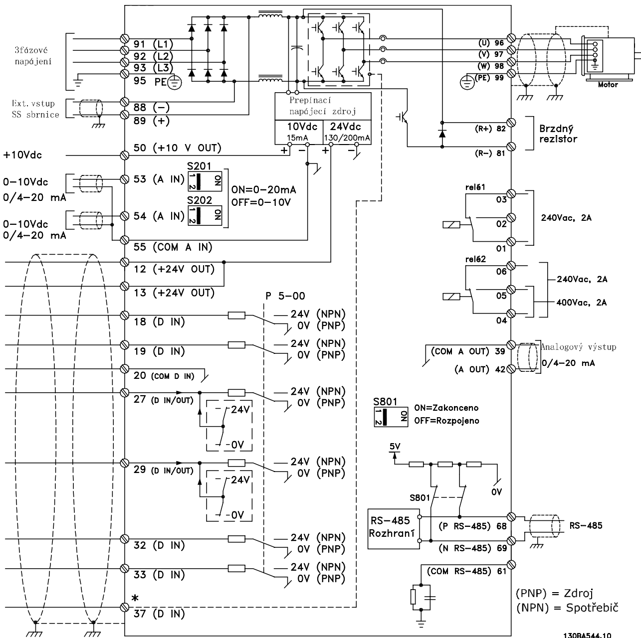
Obrázek 4.1: Na schématu jsou zobrazeny všechny elektrické svorky. (Svorka 37 je obsažena pouze v jednotkách s funkcí Bezpečného zastavení.)
