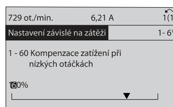
Obrázek 7.11: Příklad zobrazení na displeji.
