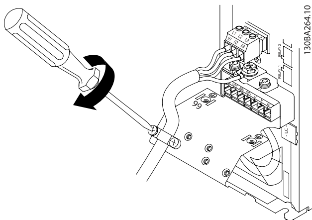
Obrázek 4.6: Nakonec dotáhněte držák síťových vodičů.
