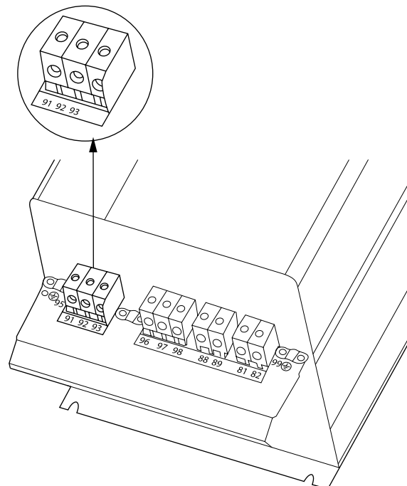
Obrázek 4.14: Připojení C3 k síti a uzemnění.
