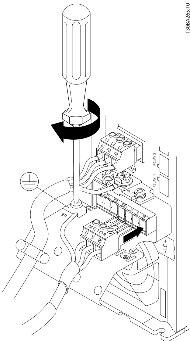
Obrázek 4.17: Nejprve upevněte zemnicí vodič motoru a potom zapojte vodiče U, V a W do konektoru a dotáhněte je.
