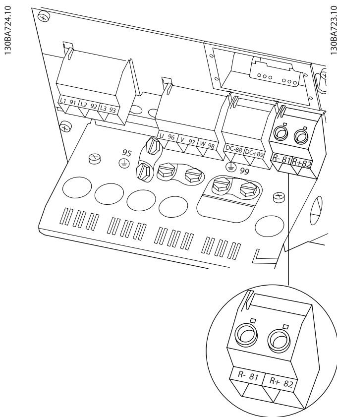
Obrázek 4.25: Svorka pro připevnění brzdy pro krytí B4.
