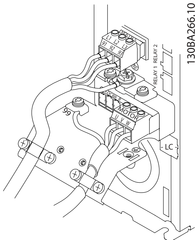
Obrázek 4.18: Namontujte kabelovou svorku, abyste zajistili 360stupňové připojení šasi a stínění. Pod svorkou je třeba odstranit vnější izolaci kabelu motoru.
