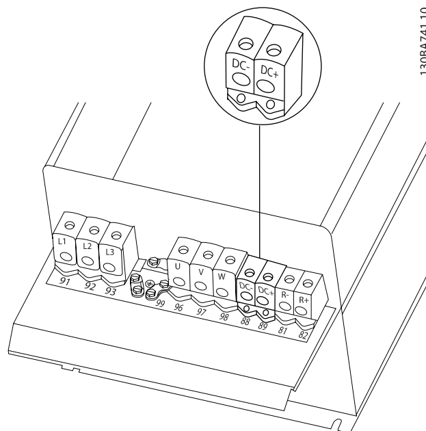
Obrázek 4.23: Připojení sběrnice DC pro krytí C4.
