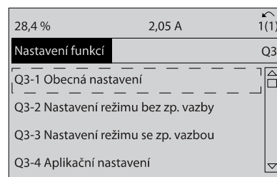
Obrázek 7.4: Krok 4: Zobrazí se možnosti menu Nastavení funkcí. Zvolte položku Q3-1 Obecná nastavení. Stiskněte tlačítko [OK].
