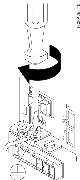
Obrázek 4.4: Při montáži kabelů nejprve namontujte a dotáhněte zemnicí kabel.
