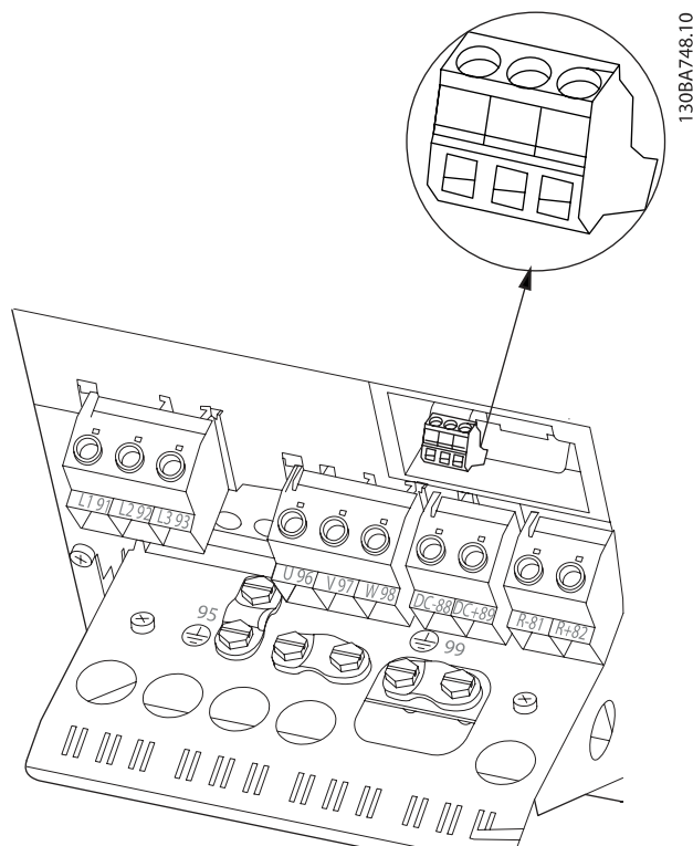
Obrázek 4.30: Svorčky pro připojení relé pro B4.
