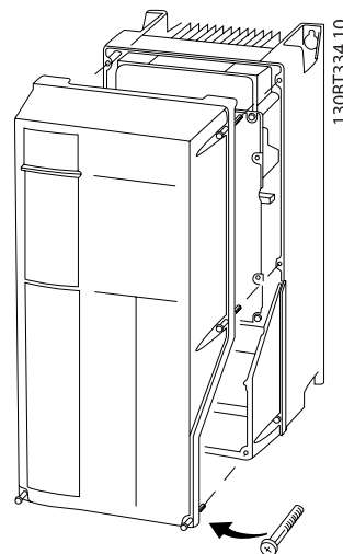
Obrázek 4.33: Přístup k řídicím svorkám pro krytí A4, A5, B1, B2, C1 a C2
