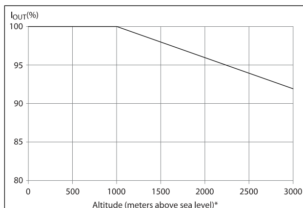
Snížení výstupního proudu v závislosti na výšce při T_{AMB, MAX} pro velikosti rámečků D, E a F.
