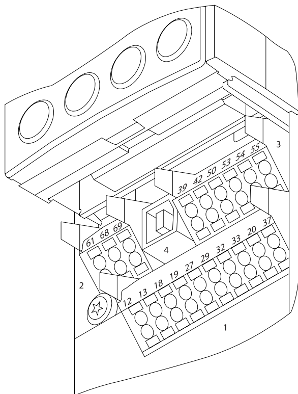
Obrázek 4.34: Řídicí svorky (všechna krytí)
