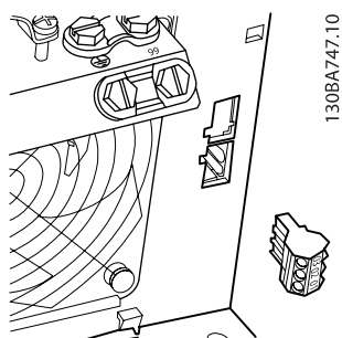
Obrázek 4.29: Svorčky pro připojení relé pro B3. Z továrny je osazen pouze jeden reléový vstup. Pokud je zapotřebí druhé relé, odstraňte vlis.
