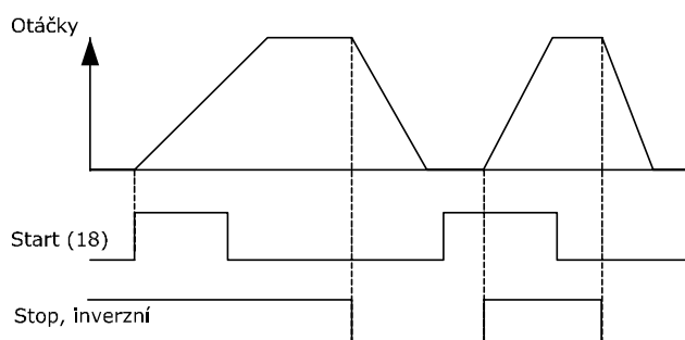
Obrázek 5.5: Svorka 37: K dispozici pouze s funkcí bezpečného zastavení!
