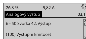
Obrázek 7.6: Krok 6: Zvolte par. 6-50. Stiskněte tlačítko [OK].
