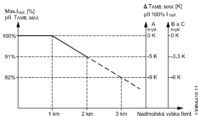
Obrazek 9.1: Snížení výstupního proudu v závislosti na výšce při T_{AMB, MAX} pro velikosti rámečků A, B a C. V případě nadmořských výšek nad 2 km se ohledně PELV obraťte na společnost Danfoss.
