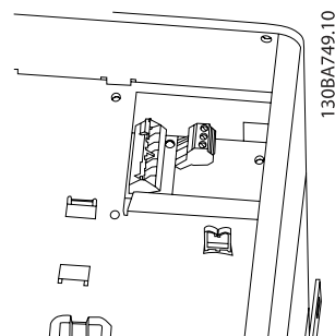
Obrázek 4.31: Svorčky pro připojení relé pro C3 a C4. Umístěny v pravém horním rohu měniče kmitočtu.
