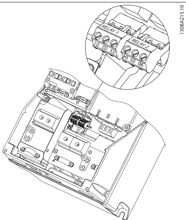
Svorky pro připojení relé (krytí A4, A5, B1 a B2).
