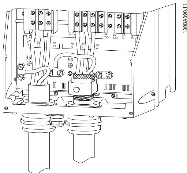
图 2.11 B 以及之上机架规格的电动机接线、主电源接线以及接地 (使用屏蔽电缆)
