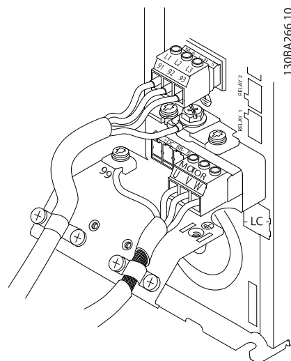
图 2.8 使用屏蔽电缆接地
