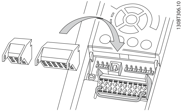
图 2.17 拔下控制端子
