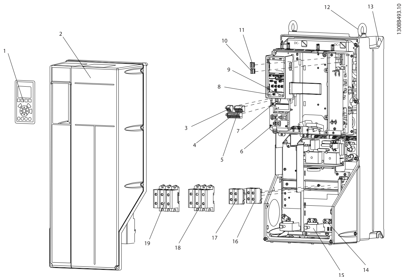
图 1.2 分解图 (规格 B 和 C)
