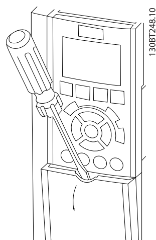
图 2.14 访问 A2、A3、B3、B4、C3 和 C4 机架的控制线路
