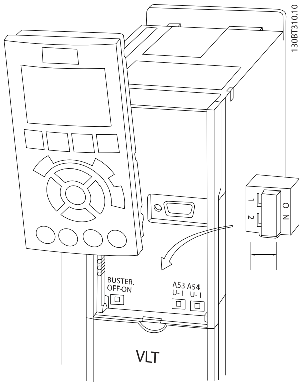
图 2.19 端子 53 和 54 的开关的位置
