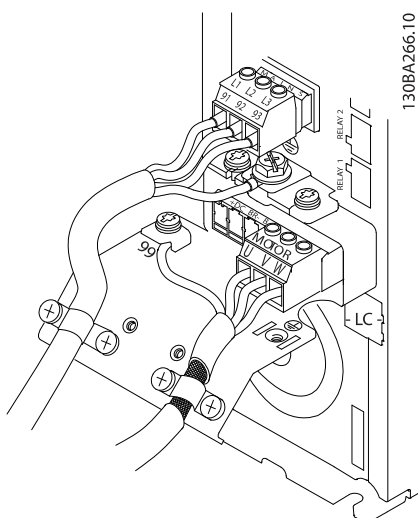
图 2.10 A 机架规格的电动机接线、主电源接线以及接地
