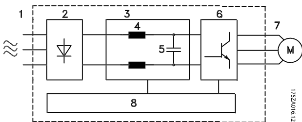
图 1.3 变频器框图
