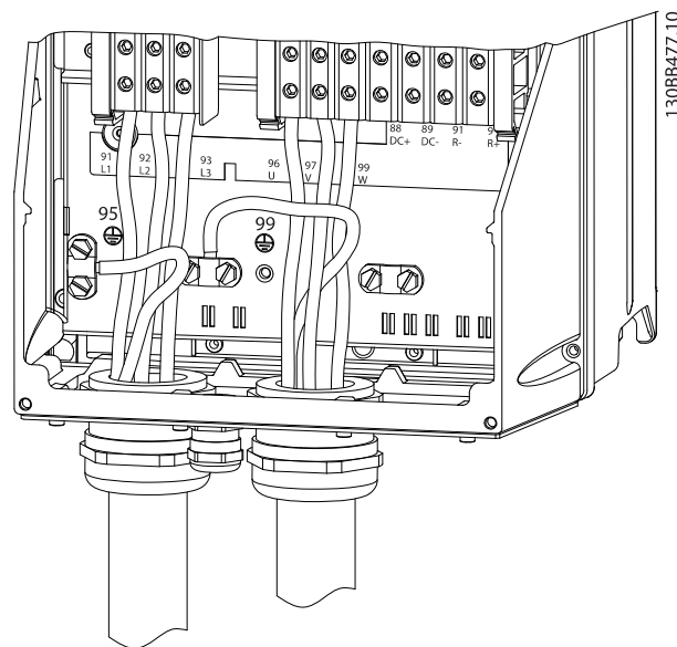
图 2.9 使用线管接地
