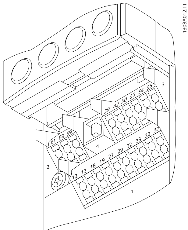
图 2.16 控制端子位置
