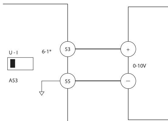
图 5.1 由外部设备提供 0-10V 控制信号的接线示例
