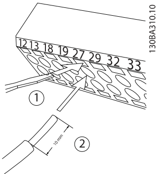
图 2.18 连接控制线缆
