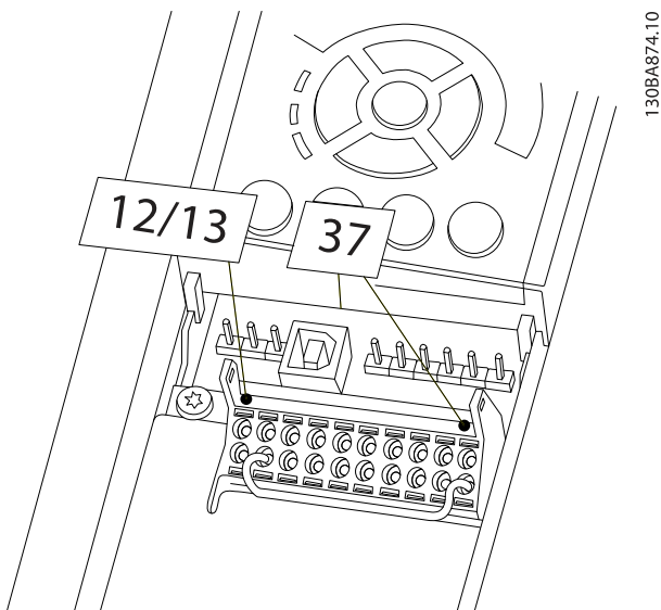
图 2.20 端子 12/13 (24 V) 与 37 之间的跳线
