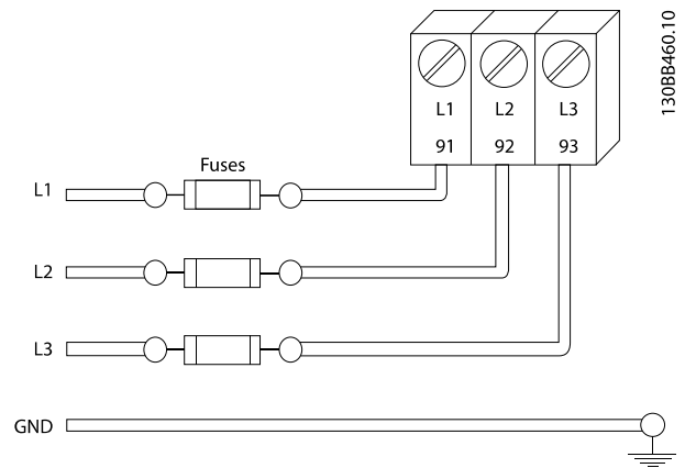
图 2.7 变频器熔断器
