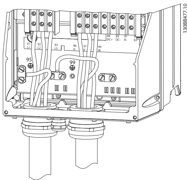
图 2.12 B 以及之上机架规格的电动机接线、主电源接线以及接地 (使用线管)
