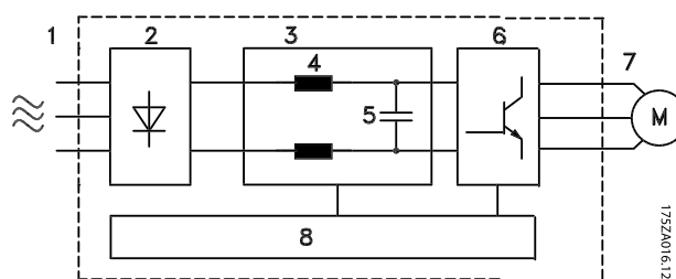
Slika 1.3 Blok dijagram frekventnog pretvarača Frekventni pretvarač
