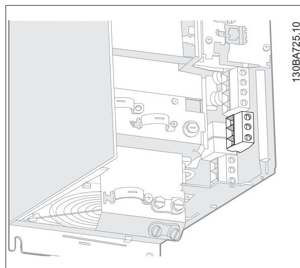
Disegno 5.15: Collegamento alla rete e messa a terra per B3 senza RFI.
