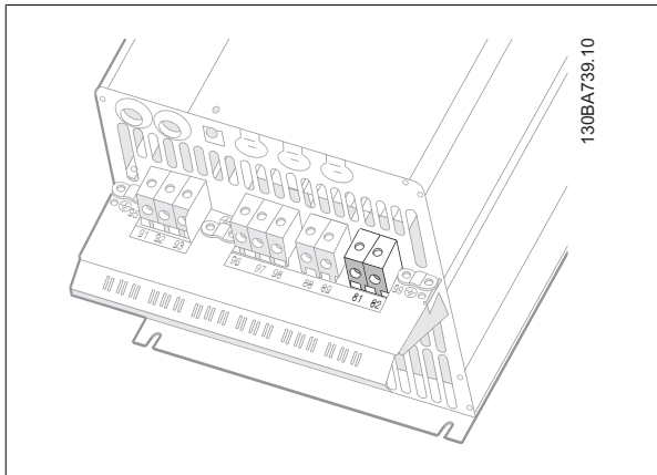
Disegno 5.41: Morsetto di collegamento freno per C3.
