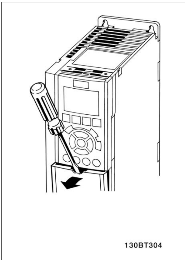
Disegno 5.29: Custodie A1, A2, A3,B3, B4, C3 e C4
