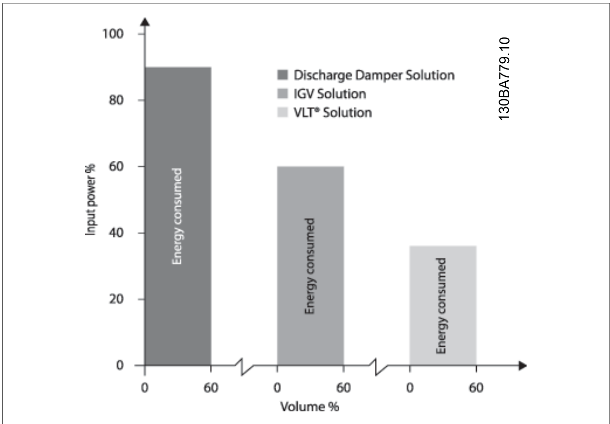
Disegno 2.4: Le valvole di scarico riducono un po' il consumo di corrente. Le palette regolabili in aspirazione offrono una riduzione del 40% ma la loro installazione è costosa. La soluzione Danfoss VLT® riduce il consumo energetico di oltre il 50% ed è facile da installare.
