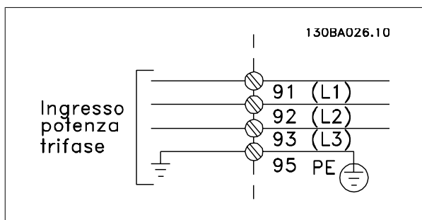
Disegno 5.5: Morsetti per la rete e la messa a terra.
