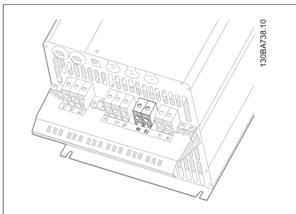
Disegno 5.37: Collegamenti bus CC per custodia C3.
