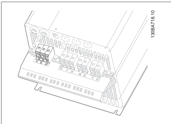
Disegno 5.18: Procedura di collegamento di C3 alla rete e messa a terra.
