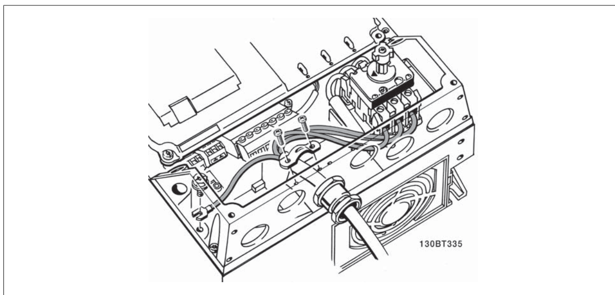
Disegno 5.12: Collegamento alla rete e messa a terra con sezionatore di rete.
