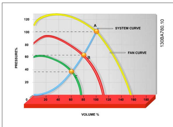
Disegno 2.1: Il grafico mostra le curve della ventola (A, B e C) per portate ridotte della ventola.
