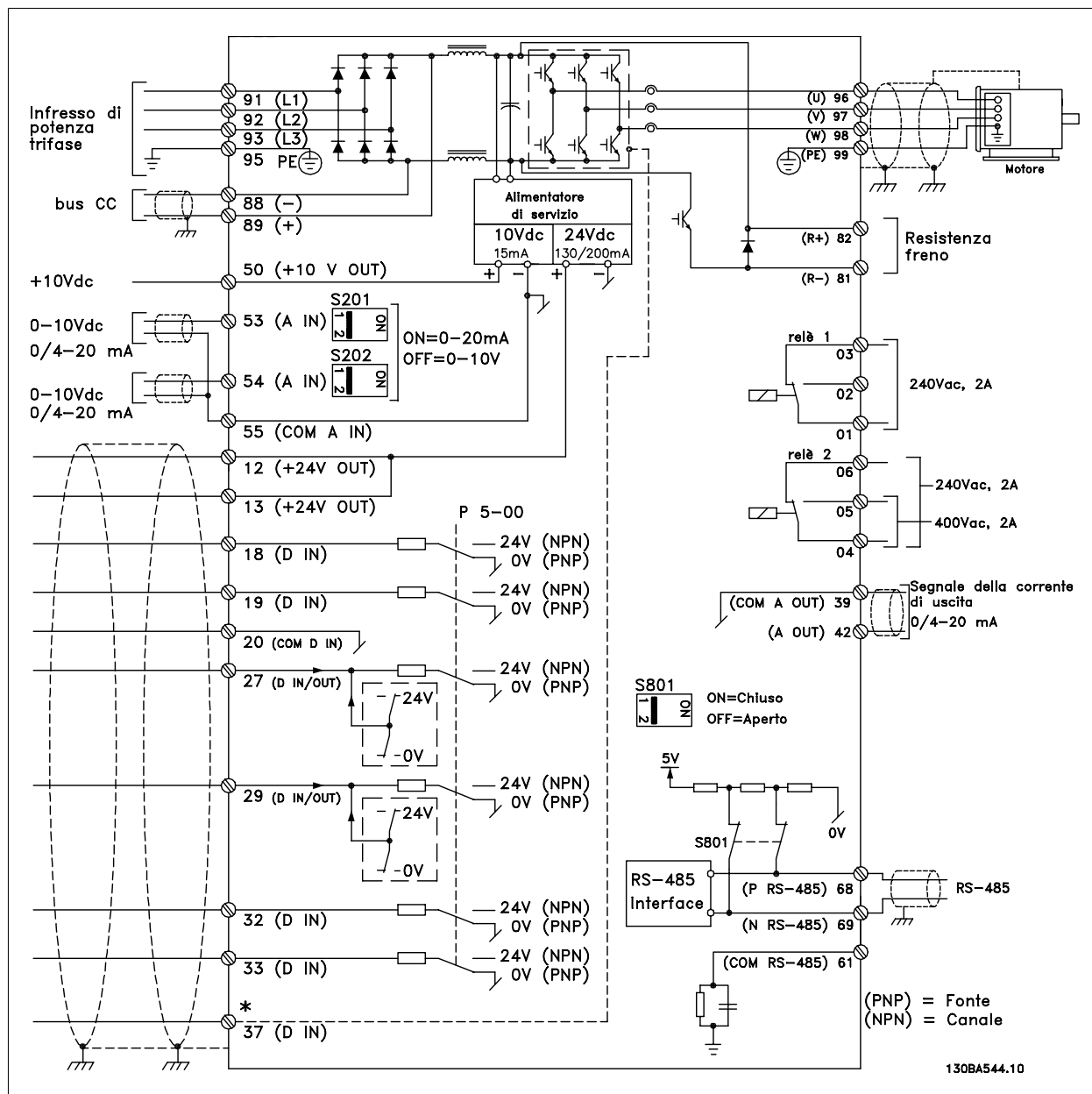
Disegno 5.34: Il diagramma mostra tutti i morsetti elettrici. (Il morsetto 37 è solo presente per unità con funzione di arresto di sicurezza).
