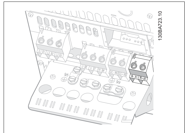
Disegno 5.40: Morsetto di collegamento freno per B4.
