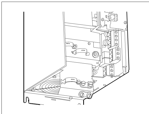
Disegno 5.35: Collegamenti bus CC per custodia B3.
