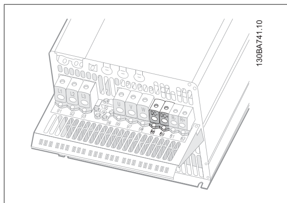
Disegno 5.38: Collegamenti bus CC per custodia C4.
