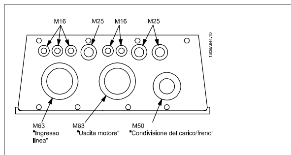
Disegno 5.4: Fori di ingresso dei cavi per la custodia C2. La soluzione proposta per l'uso dei fori di ingresso è solo a titolo di esempio; sono possibili anche altre soluzioni.
