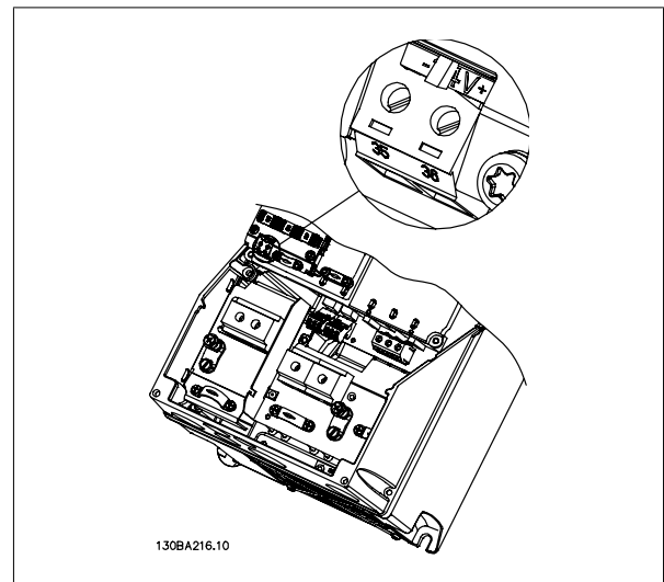
Disegno 3.3: Collegamento all'alimentazione di back-up 24 V (A5-C2).
