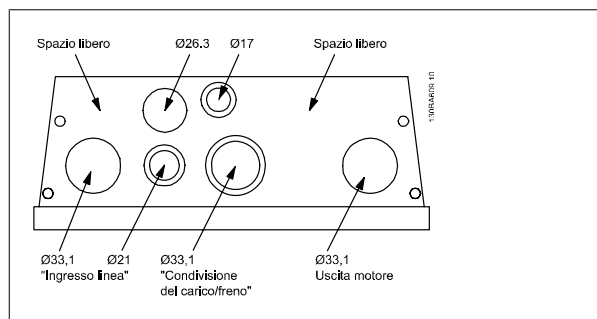
Disegno 5.1: Fori di ingresso dei cavi per la custodia B1. La soluzione proposta per l'uso dei fori di ingresso è solo a titolo di esempio; sono possibile anche altre soluzioni.
