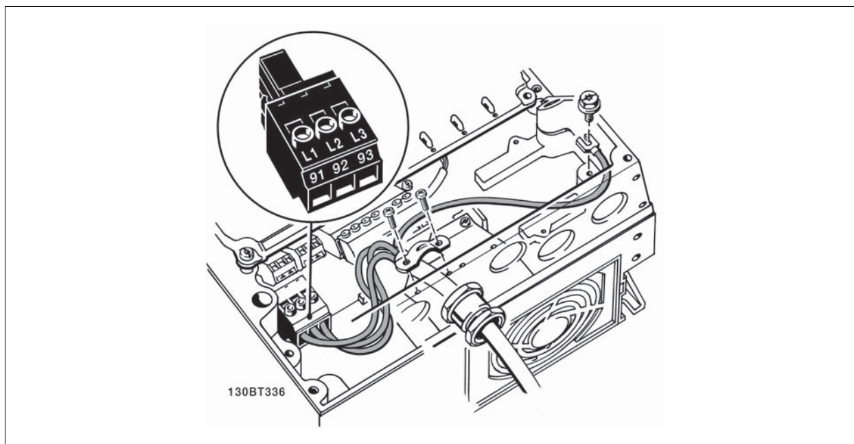
Disegno 5.11: Collegamento alla rete e messa a terra senza sezionatore di rete. Tenere presente che viene utilizzato un pressacavo.
