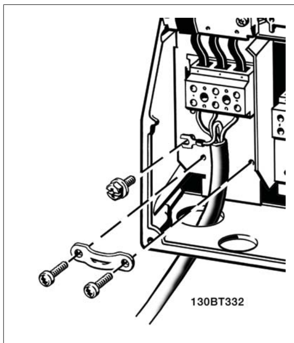
Disegno 5.13: Collegamento alla rete e messa a terra per B1 e B2.
