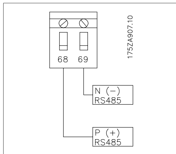
Disegno 7.1: Collegamento ai morsetti di rete
