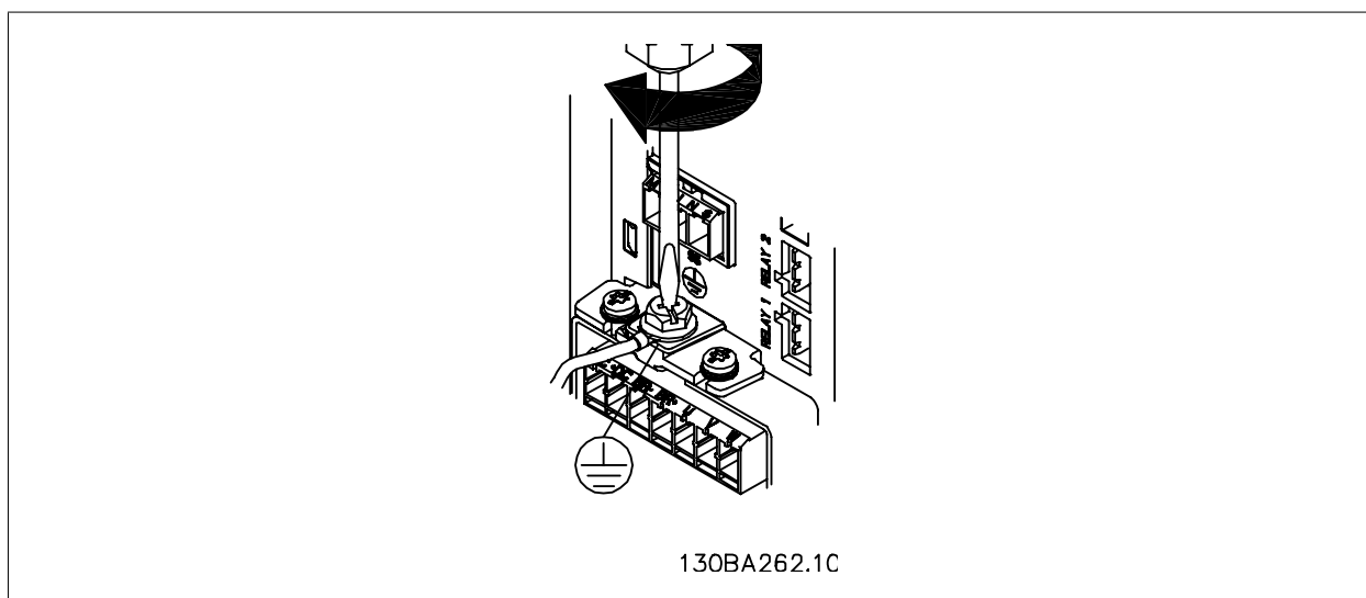
Disegno 5.8: Quando si montano i cavi, prima deve essere montato e serrato il cavo di terra.
