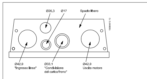
Disegno 5.2: Fori di ingresso dei cavi per la custodia B2. La soluzione proposta per l'uso dei fori di ingresso è solo a titolo di esempio; sono possibile anche altre soluzioni.
