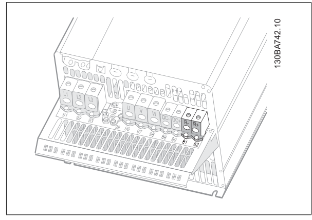
Disegno 5.42: Morsetto di collegamento freno per C4.
