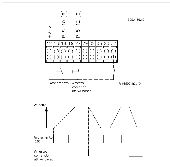
Disegno 5.33: Morsetto 37 solo disponibile con funzione di arresto di sicurezza!
