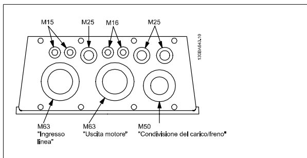
Disegno 5.3: Fori di ingresso dei cavi per la custodia C1. La soluzione proposta per l'uso dei fori di ingresso è solo a titolo di esempio; sono possibili anche altre soluzioni.
