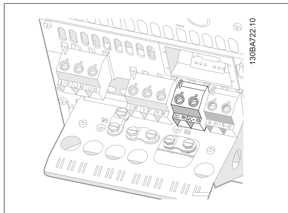
Disegno 5.36: Collegamenti bus CC per custodia B4.
