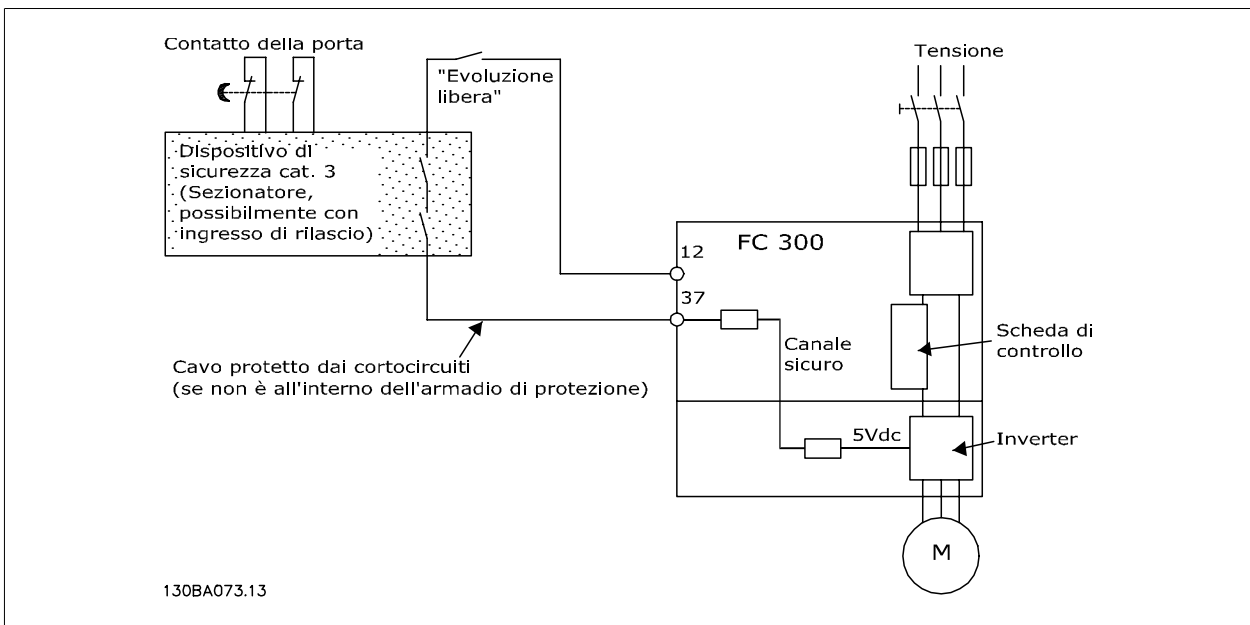
Disegno 2.9: Illustrazione degli aspetti essenziali di un'installazione al fine di ottenere Categoria d'arresto 0 (EN 60204-1) con Categoria di sicurezza 3 (EN 954-1).
