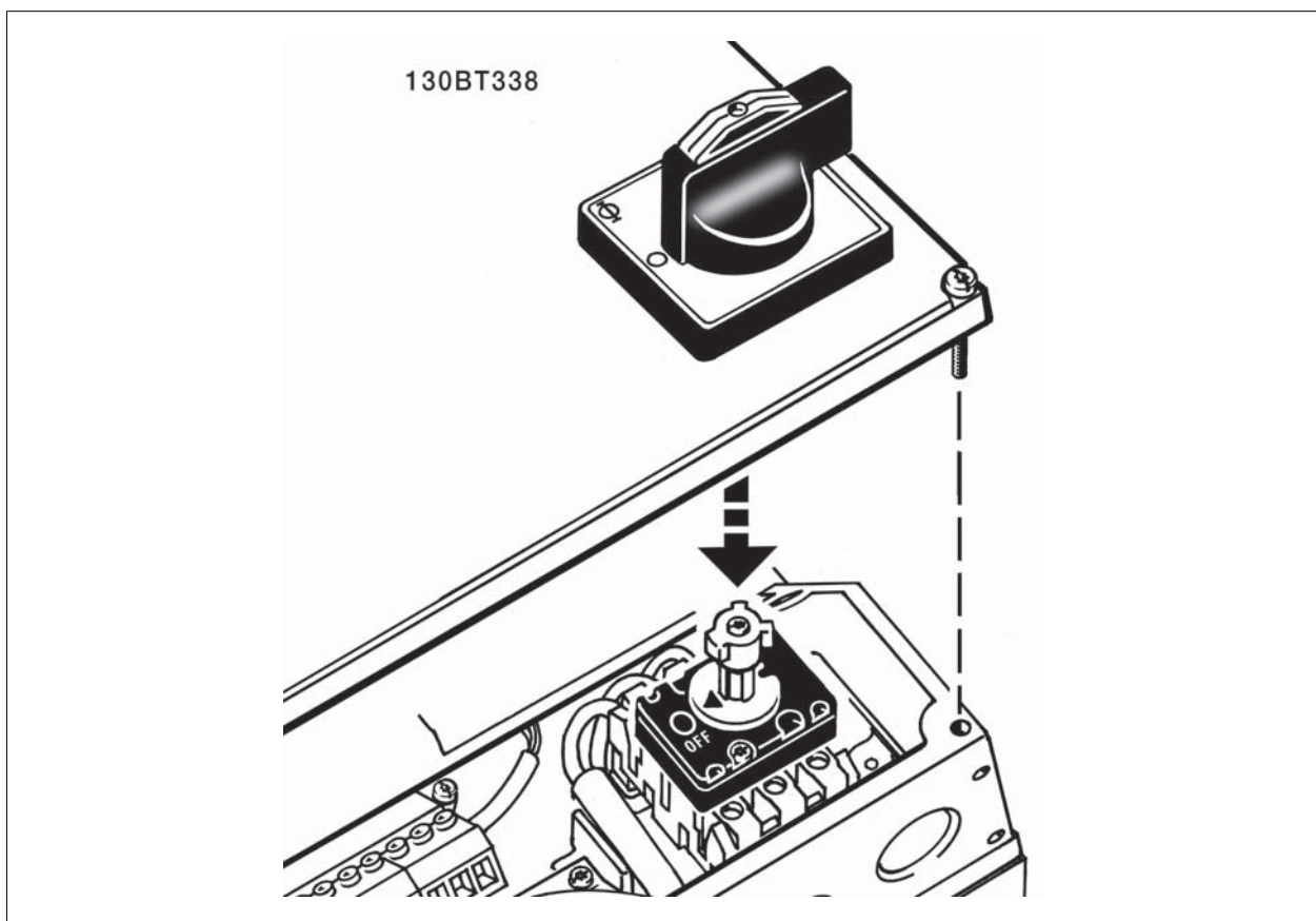
Disegno 5.32: Installazione della custodia IP21 / IP55 / NEMA TIPO 12 con sezionatore di rete.
