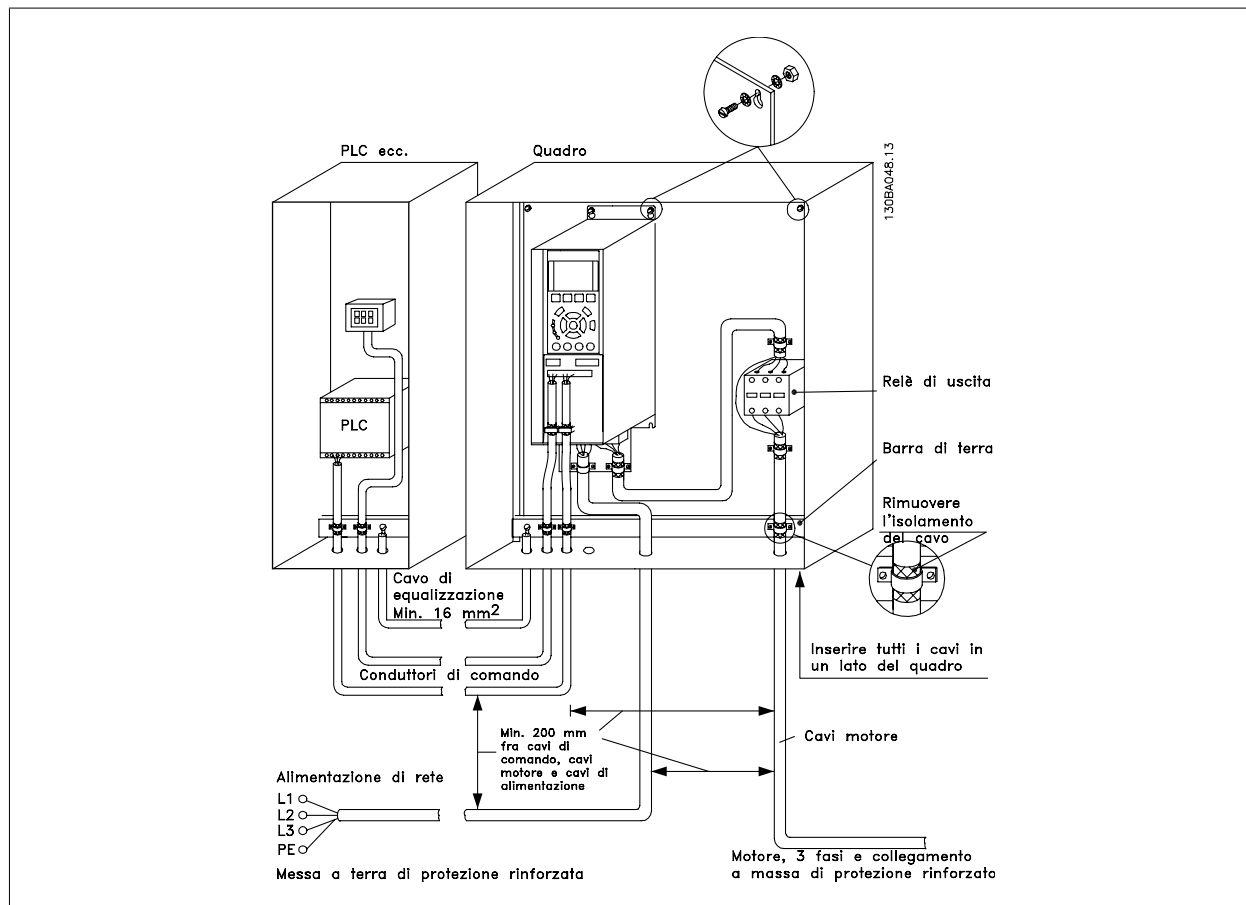
Disegno 5.48: Installazione elettrica conforme ai requisiti EMC di un convertitore di frequenza.
