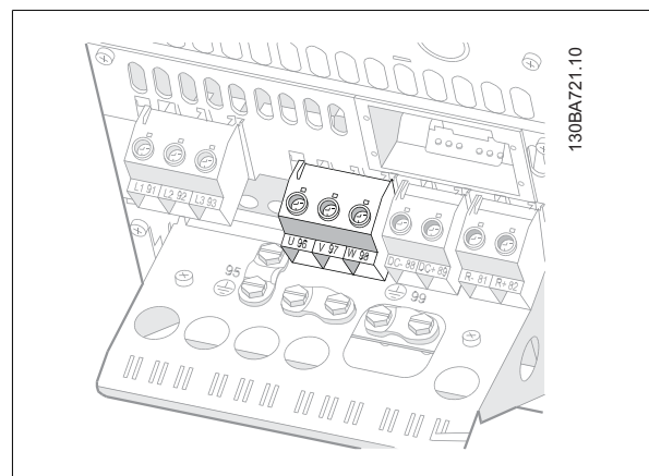
Disegno 5.26: Prima fissare il conduttore di terra del motore, quindi inserire i fili U, V e W del motore nel morsetto e serrarli. Assicurare che l'isolamento esterno del cavo motore viene rimosso sotto il pressacavo EMC.
