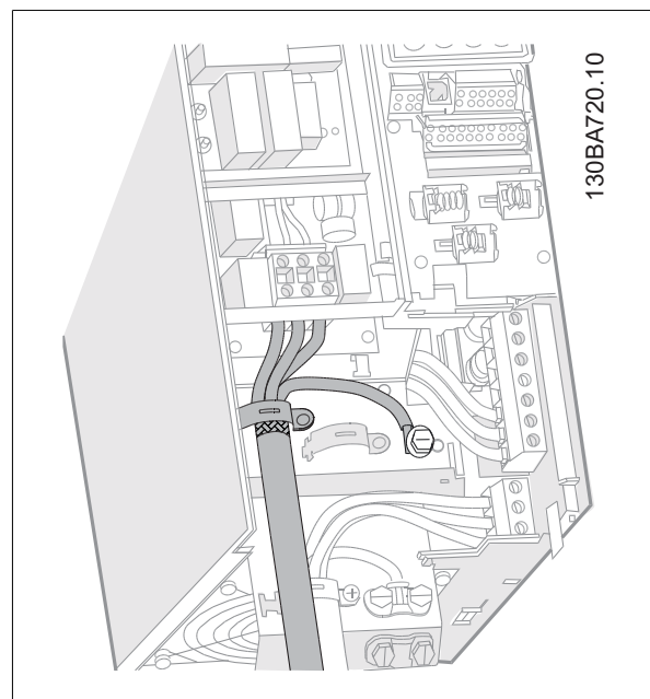
Disegno 5.14: Procedura di collegamento alla rete e messa a terra per B3 con RFI.
