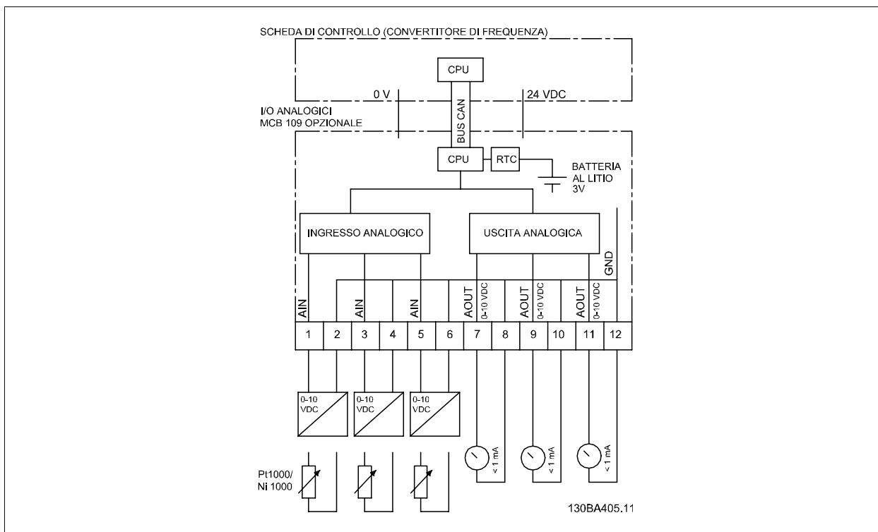
Disegno 3.4: Diagramma di principio per I/O analogici montati nel convertitore di frequenza.
