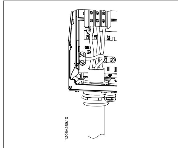
Disegno 5.17: Procedura di collegamento alla rete e messa a terra per C1 e C2.
