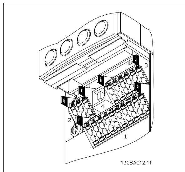
Disegno 5.31: Morsetti di controllo (tutte le custodie)
