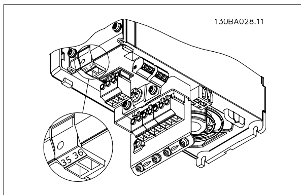
Disegno 3.2: Collegamento all'alimentazione di back-up 24 V (A2-A3).
