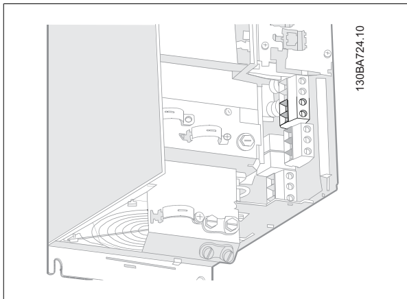
Disegno 5.39: Morsetto di collegamento freno per B3.
