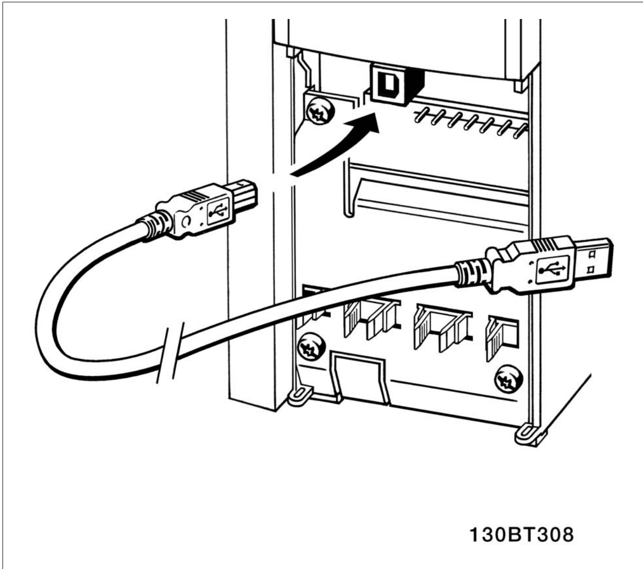
Disegno 5.47: Per collegamenti con cavo di controllo, vedere la sezione Morsetti di controllo .
