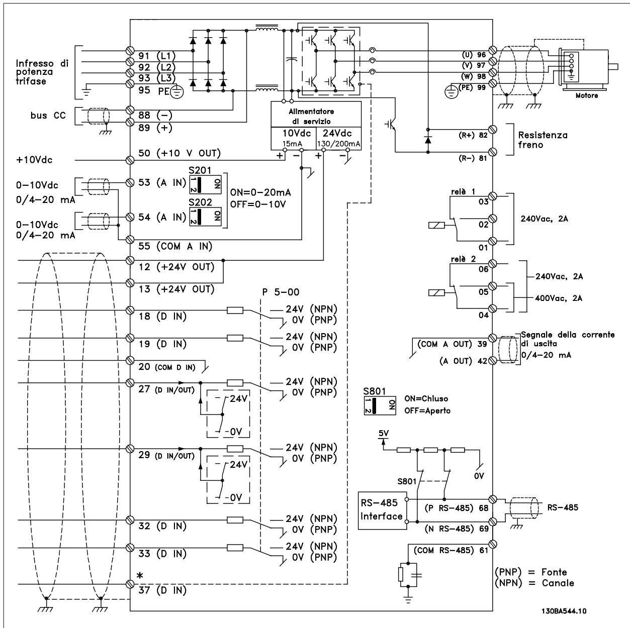
Disegno 2.7: Il diagramma mostra tutti i morsetti elettrici. (Il morsetto 37 è solo presente per unità con funzione di arresto di sicurezza).
