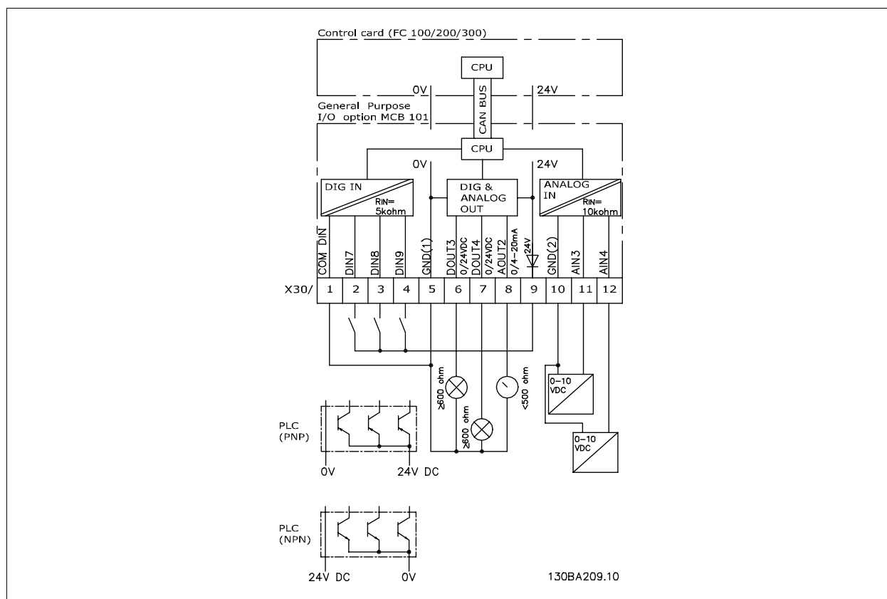
Disegno 3.1: Diagramma di principio
