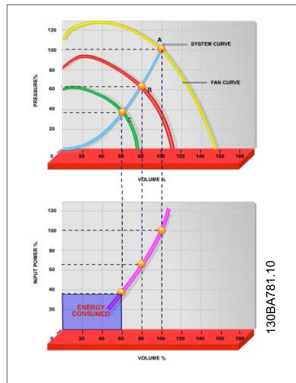
Disegno 2.2: Quando si utilizza un convertitore di frequenza per ridurre la capacità della ventola al 60%, in applicazioni tipiche possono essere ottenuti oltre il 50% di risparmi energetici.
