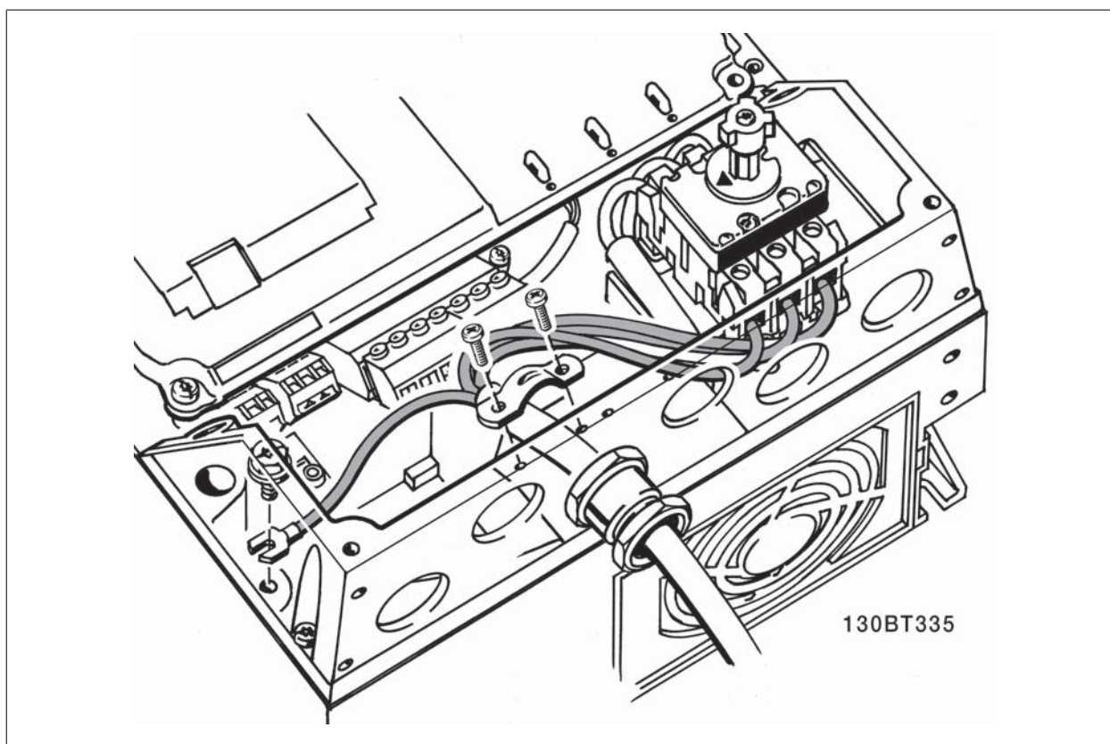
Disegno 5.6: Procedura di collegamento alla rete e messa a terra con sezionatore (custodia A5).
