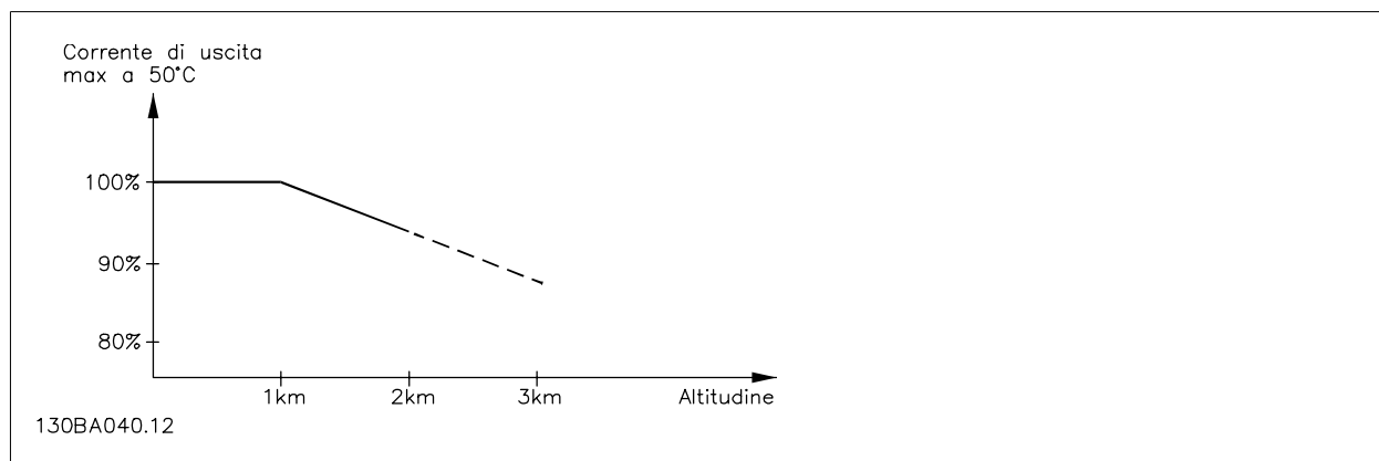
Disegno 8.1: Declassamento della corrente di uscita rispetto all'altitudine, con T_{AMB, MAX} . Per altitudini superiori ai 2000 m, contattare Danfoss per informazioni sulle caratteristiche PELV.
