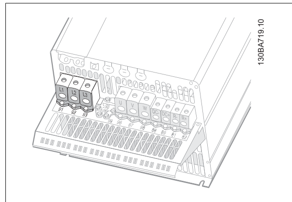
Disegno 5.19: Procedura di collegamento di C4 alla rete e messa a terra.
