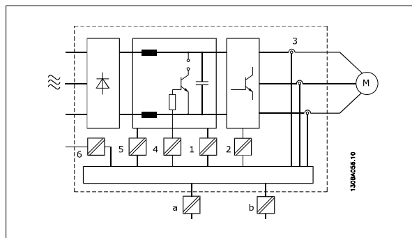
Disegno 2.6: Isolamento galvanico
