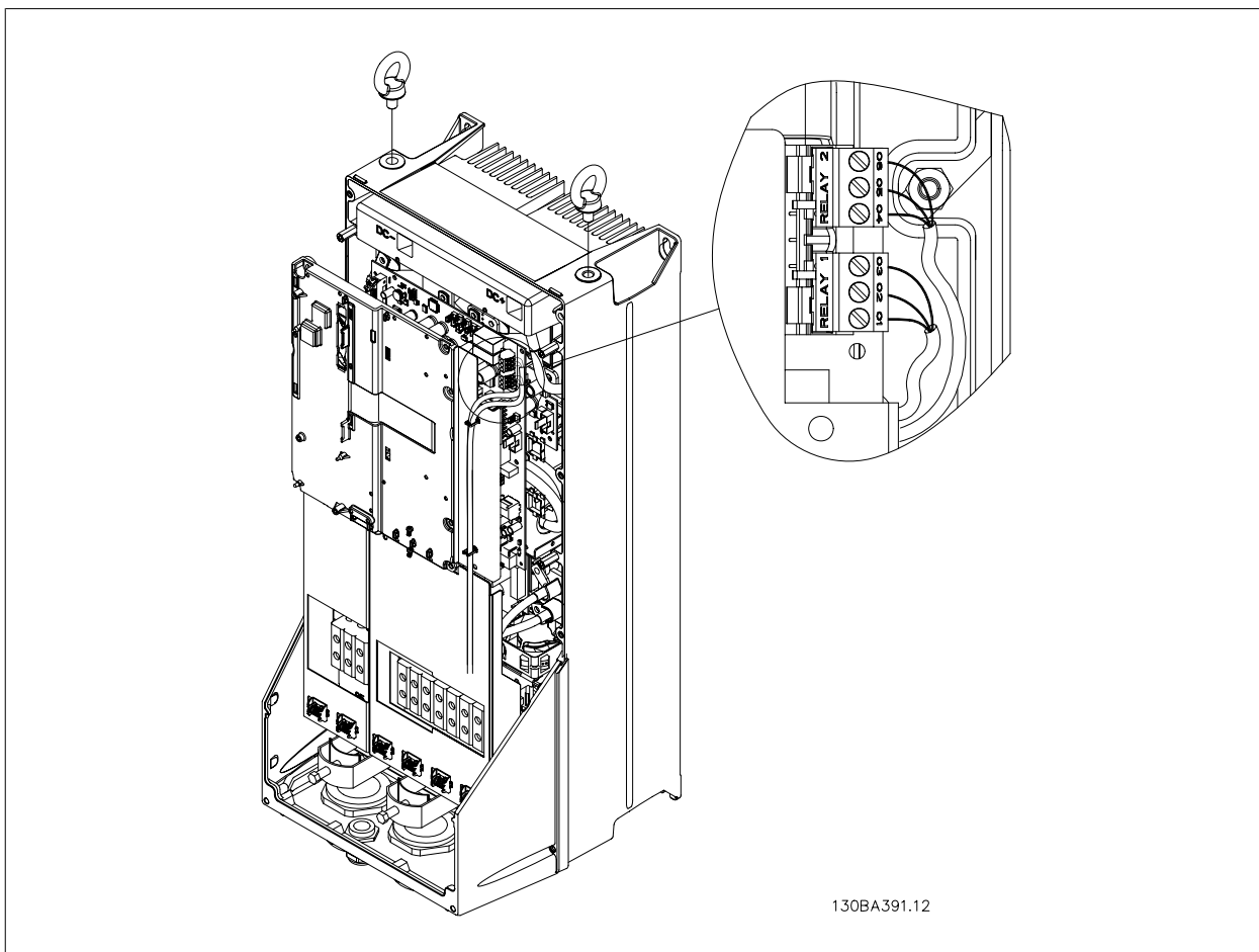
Disegno 5.43: Morsetti per il collegamento relè (custodie C1 e C2).
