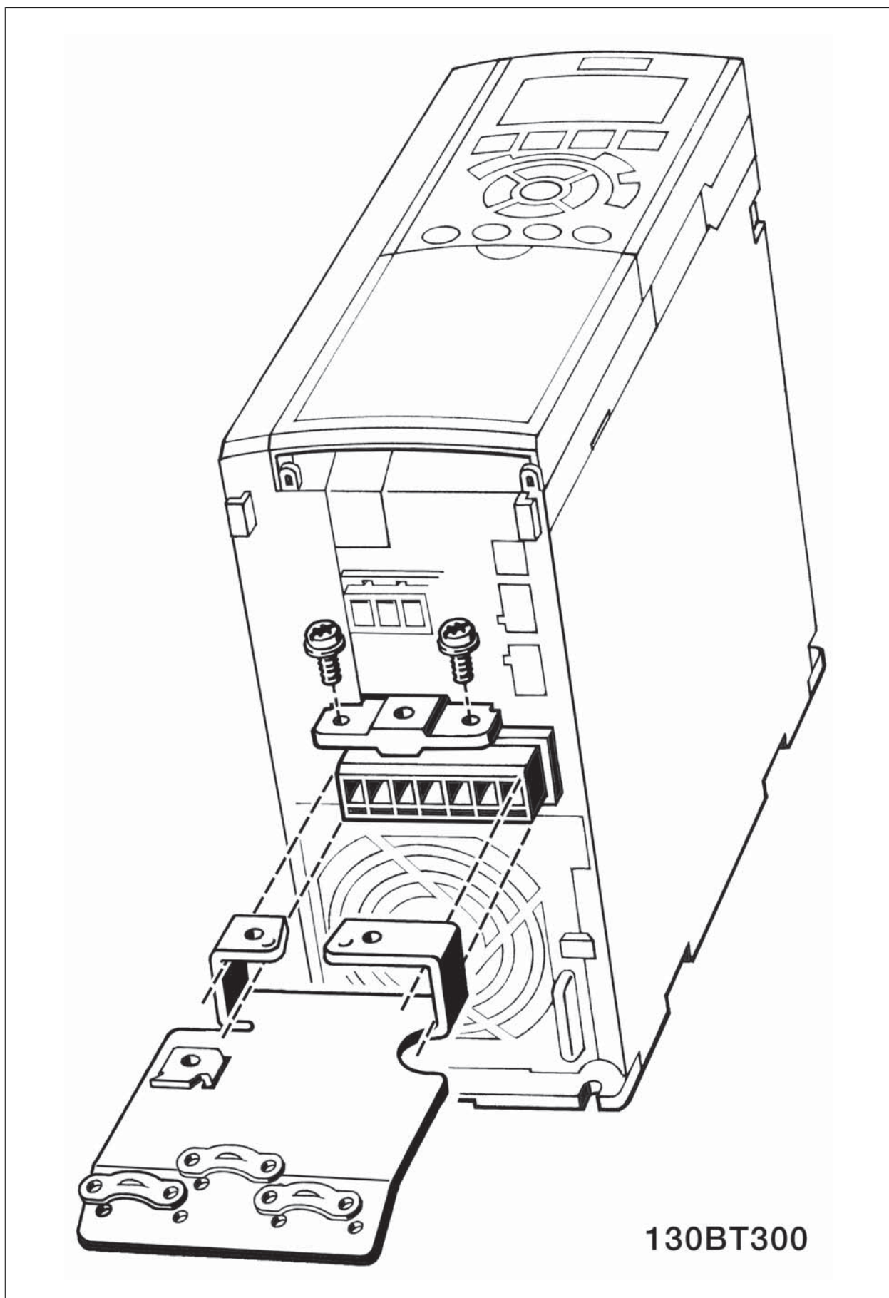
Disegno 5.20: Montaggio della piastra di disaccoppiamento.
