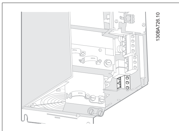
Disegno 5.25: Prima fissare il conduttore di terra del motore, quindi inserire i fili U, V e W del motore nel morsetto e serrarli. Assicurare che l'isolamento esterno del cavo motore viene rimosso sotto il pressacavo EMC.
