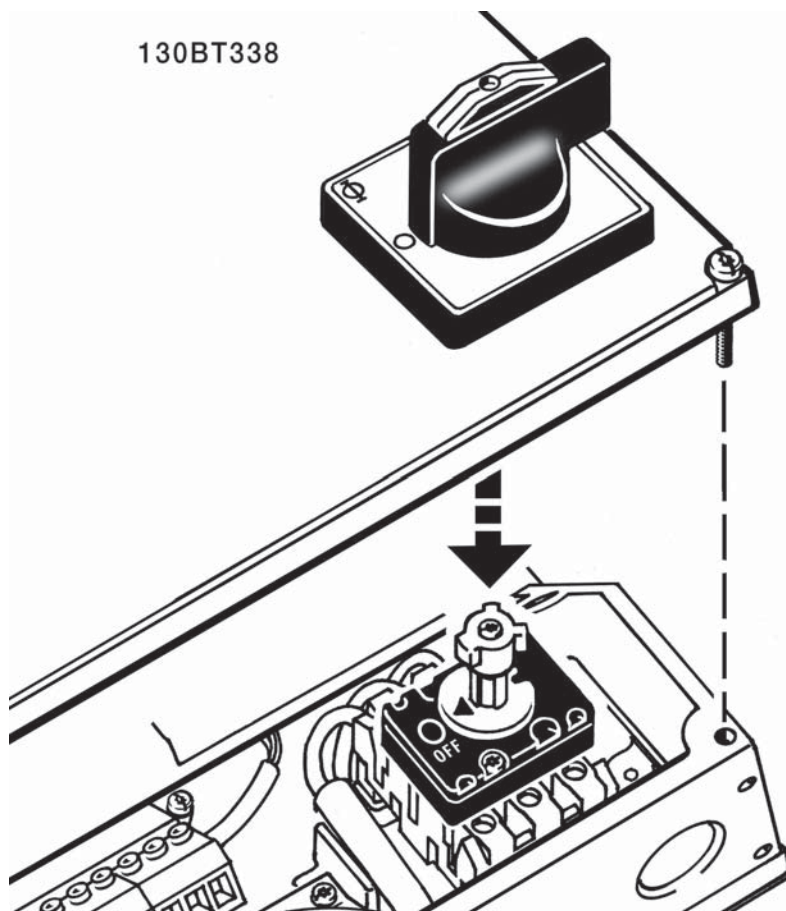
Ilustração 5.35: Montagem do compartimento do IP21 / IP55 / NEMA TIPO 12 com o disjuntor de rede elétrica.
