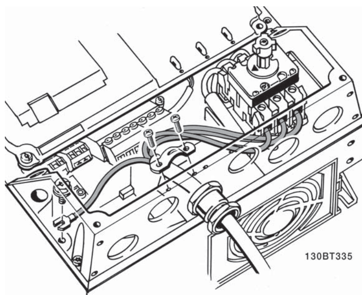
Ilustração 5.8: Como fazer a conexão à rede elétrica e ao ponto de aterramento (gabinete metálico A5).
