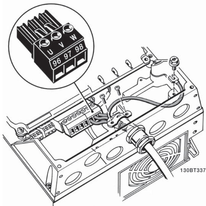
Ilustração 5.25: Primeiro, faça a terminação do terra do motor, em seguida, instale os fios U,V e W no terminal e aperte. Garanta que a isolação externa do cabo do sob a braçadeira de EMC seja removida.
