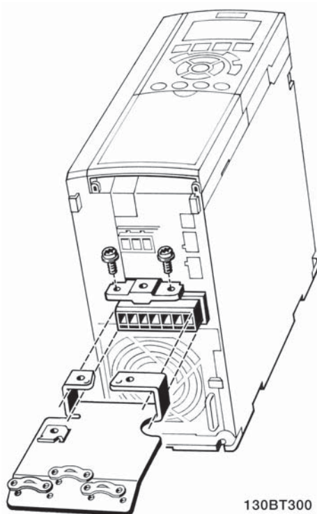
Ilustração 5.22: Montagem da placa de desacoplamento.
