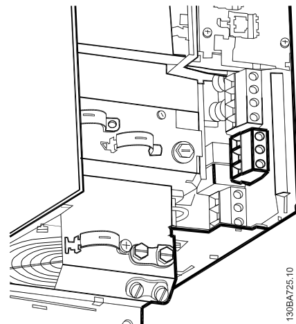
Ilustração 5.16: Como fazer a conexão na rede e aterramento do B3 sem o RFI.
