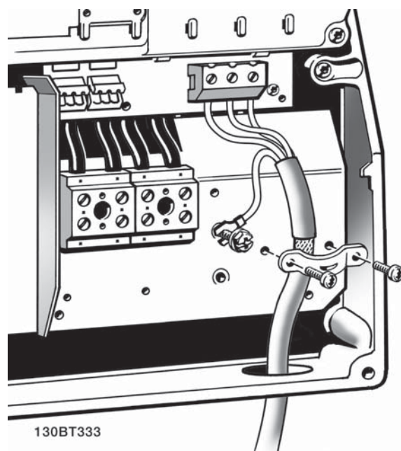
Ilustração 5.26: Primeiro, faça a terminação do terra do motor, em seguida, instale os fios U, V e W no terminal e aperte. Garanta que a isolação externa do cabo do sob a braçadeira de EMC seja removida.
