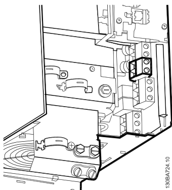
Ilustração 5.42: Terminal de conexão do freio para o B3.
