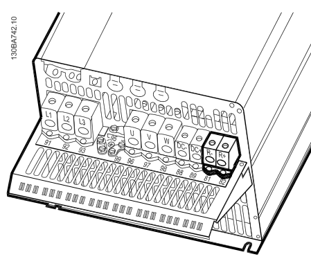
Ilustração 5.45: Terminal de conexão do freio para o C4.
