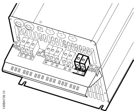
Ilustração 5.44: Terminal de conexão do freio para o C3.
