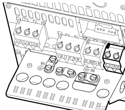
Ilustração 5.43: Terminal de conexão do freio para o B4.
