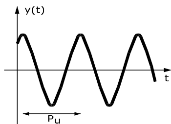
Ilustração 2.5: Sistema marginalmente estável
