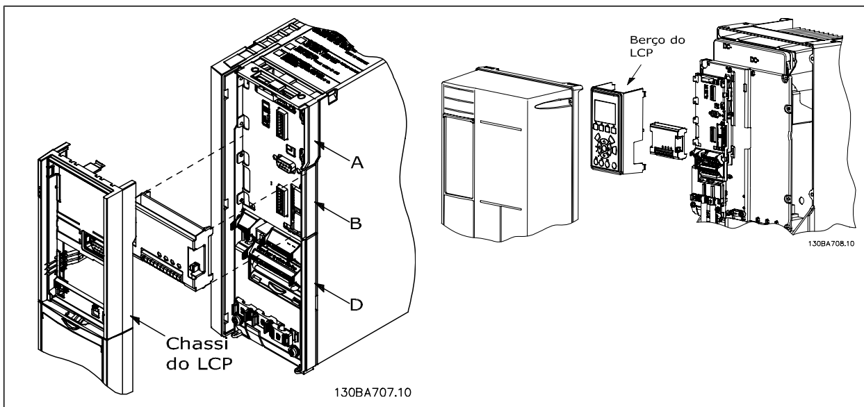
Gabinetes metálicos A2, A3 e B3
