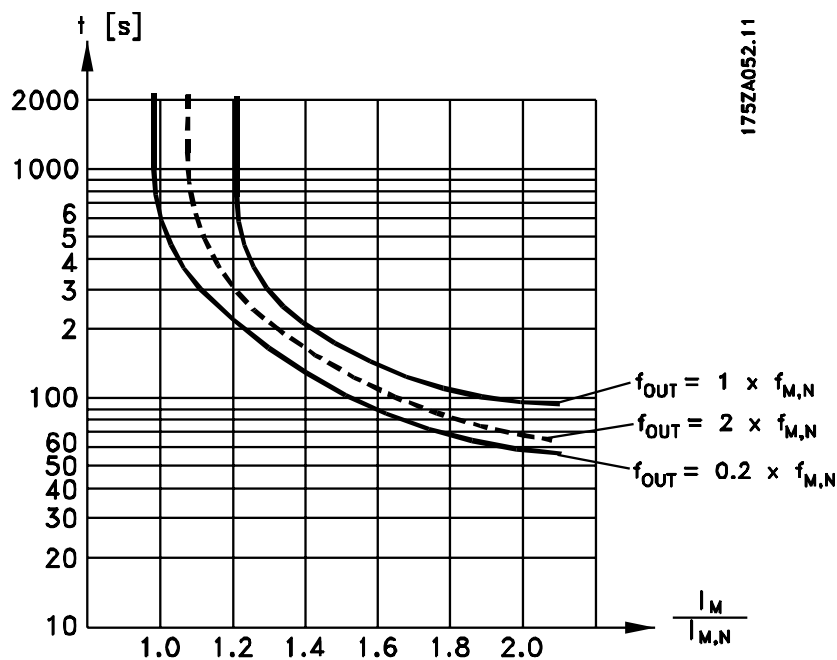
Ilustração 2.7: O eixo X mostra a relação entre a I_{motor} e a I_{motor} nominal. O eixo Y exibe o tempo, em segundos, antes do ETR cortar e desarmar o drive. As curvas mostram a velocidade nominal característica no dobro da velocidade nominal e em 0,2x a velocidade nominal.
