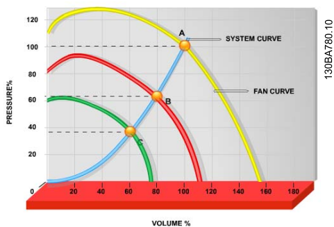
图 2.1: 下图显示了降低风扇容量时的风扇曲线（A、B 和 C）。
