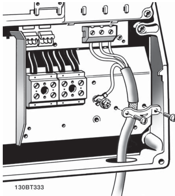
图 5.26: 首先, 断开电动机接地, 然后, 将电动机 U、V 和 W 电线接入端子并拧紧。请确保去除 EMC 电缆夹下面电动机电缆的外部绝缘层。
