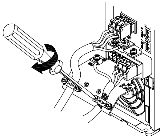
图 5.24: 安装电缆夹, 以确保机架和屏蔽丝网达到 360 度连接。注意, 请去除电缆夹下面电动机电缆的外部绝缘层。
