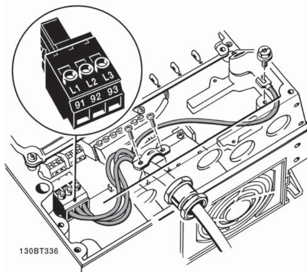
图 5.13: 如何在不使用主电源断路器连接主电源和接地。注意, 需要使用电缆夹。
