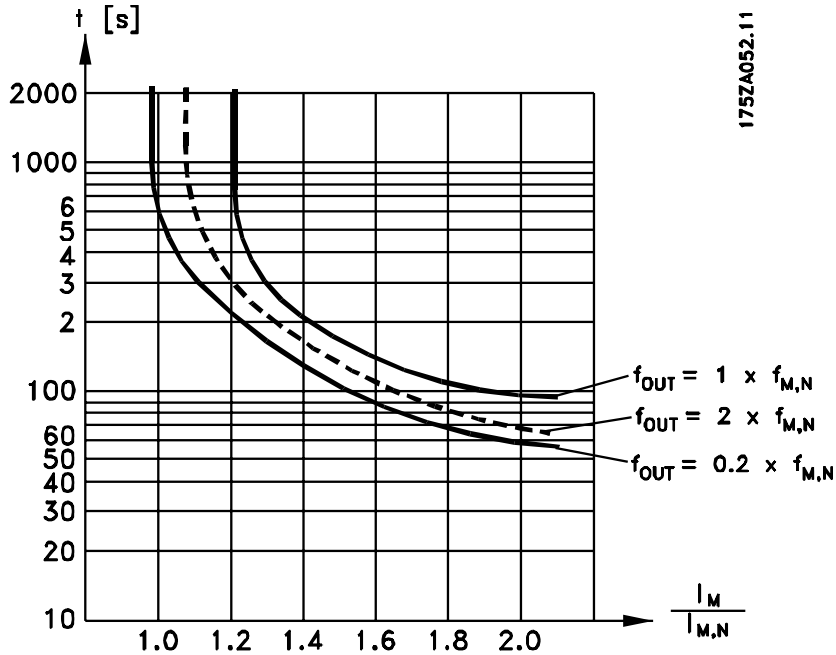
图 2.7: X 轴显示了 I_{motor} 和额定 I_{motor} 的比。Y 轴显示了 ETR 断开并使变频器跳闸之前的时间 (秒)。曲线显示了额定速度下、2 倍额定速度下以及 0.2 被额定速度下的特性。
