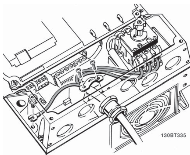
图 5.14: 如何使用主电源断路器连接主电源和接地。
