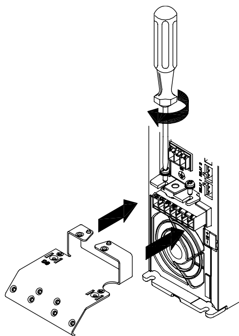
图 5.9: 首先, 将两个螺钉安装到固定板上, 然后将其滑动入位并完全拧紧。
