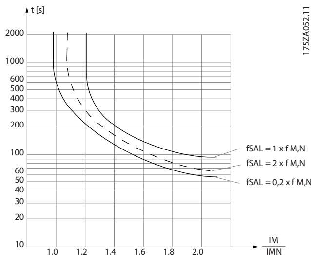
Ilustración 2.19 El eje X muestra la relación entre los valores I_{motor} e I_{motor} nominales. El eje Y muestra el intervalo en segundos antes de que el ETR se corte y desconecte el convertidor de frecuencia. Las curvas muestran la velocidad nominal característica al doble de la velocidad nominal y al 0,2x de la velocidad nominal.
