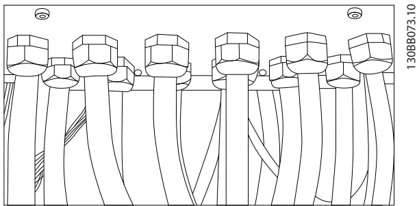
Ilustración 5.14 Ejemplo de instalación adecuada de la placa de prensacables.
