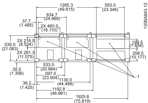
Ilustración 5.19 Tamaño del bastidor F3
