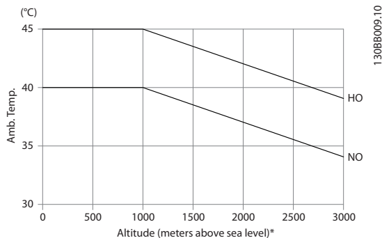
Reducción de intensidad de salida frente a la altitud a TAMB, MAX para tamaños de bastidor D, E y F.
