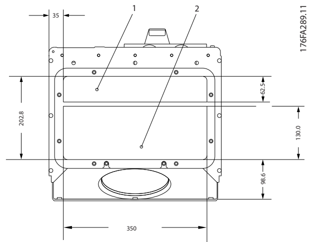
Ilustración 5.16 Tamaño del bastidor E1
