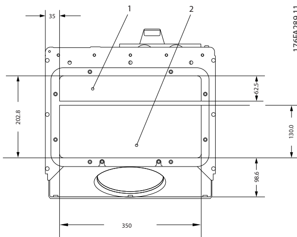
Ilustración 5.15 Tamaños del bastidor D1 + D2
