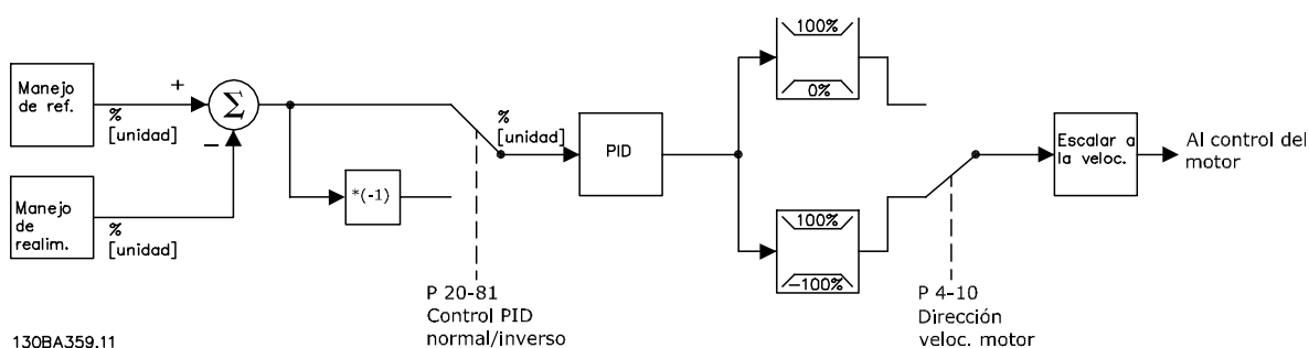
Ilustración 2.11 Diagrama de bloques de controlador de lazo cerrado
