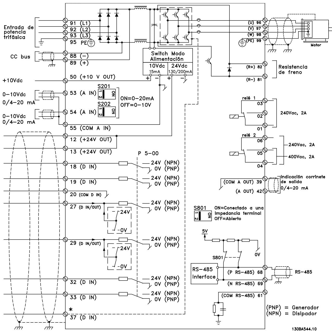
Ilustración 5.23 Diagrama que muestra todos los terminales eléctricos.
