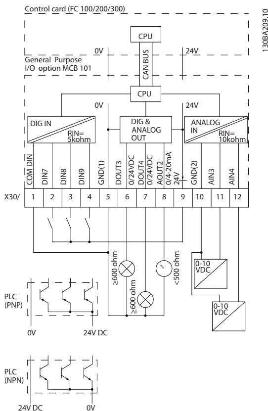
Ilustración 3.3 Diagrama básico
