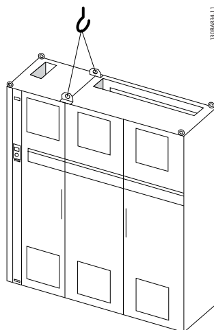
Ilustración 5.3 Método de elevación recomendado, tamaño del bastidor F2 (460 V, 1000 a 1200 CV, 575/690 V, 1250 a 1350 CV).
