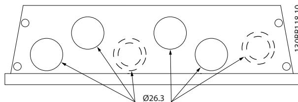
Ilustración 5.7 Orificios de entrada para cables en la protección A5. La utilización que se sugiere de los orificios es solo una recomendación. Son posibles otras soluciones.
