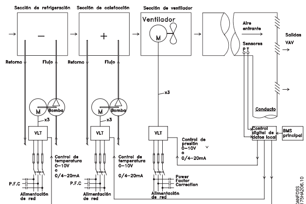
Ilustración 2.8 En la ilustración se muestra un sistema de ventiladores controlado por convertidores de frecuencia.
