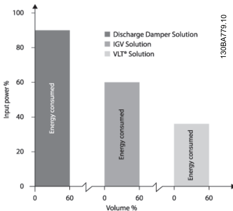
Ilustración 2.7 Los atenuadores de descarga reducen el consumo de energía en cierta medida. Las aletas guiadoras variables de entrada ofrecen un 40 % de reducción pero su instalación es costosa. El Danfoss convertidor de frecuencia reduce el consumo de energía en más de un 50 % y es fácil de instalar.
