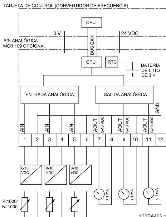
Ilustración 3.6 Esquema de principio para E/S analógicas montadas en convertidor de frecuencia.
