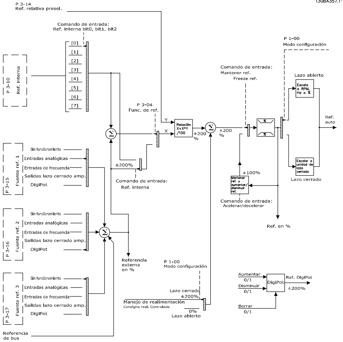
Ilustración 2.13 Diagrama de bloque que muestra la referencia remota
