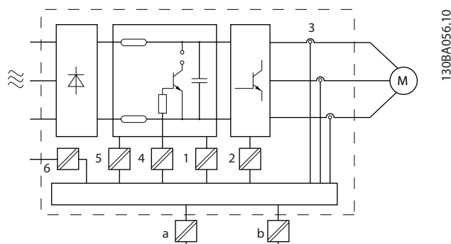
Ilustración 2.14 Aislamiento galvánico
