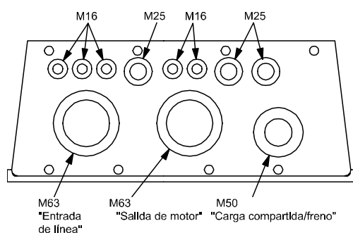
Ilustración 5.13 Orificios de entrada para cables en la protección C2. La utilización que se sugiere de los orificios es solo una recomendación. Son posibles otras soluciones.
