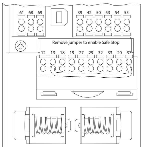
Ilustración 7.2 Terminales de la tarjeta de control
