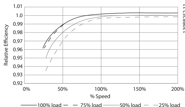
Ilustración 8.1 Curvas de rendimiento típico
