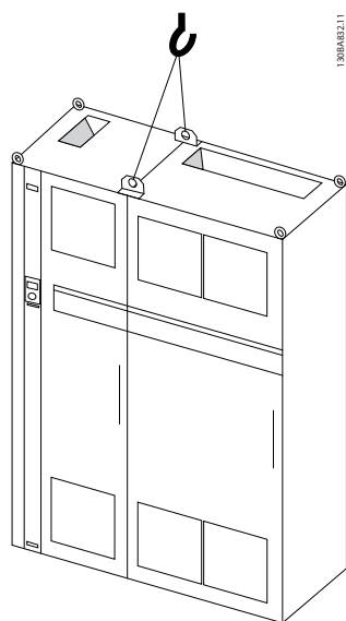
Ilustración 5.2 Método de elevación recomendado, tamaño del bastidor F1 (460 V, 600 a 900 CV, 575/690 V, 900 a 1150 CV).
