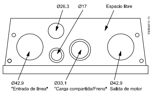
Ilustración 5.10 Orificios de entrada para cables en la protección B2. La utilización que se sugiere de los orificios es solo una recomendación. Son posibles otras soluciones.
