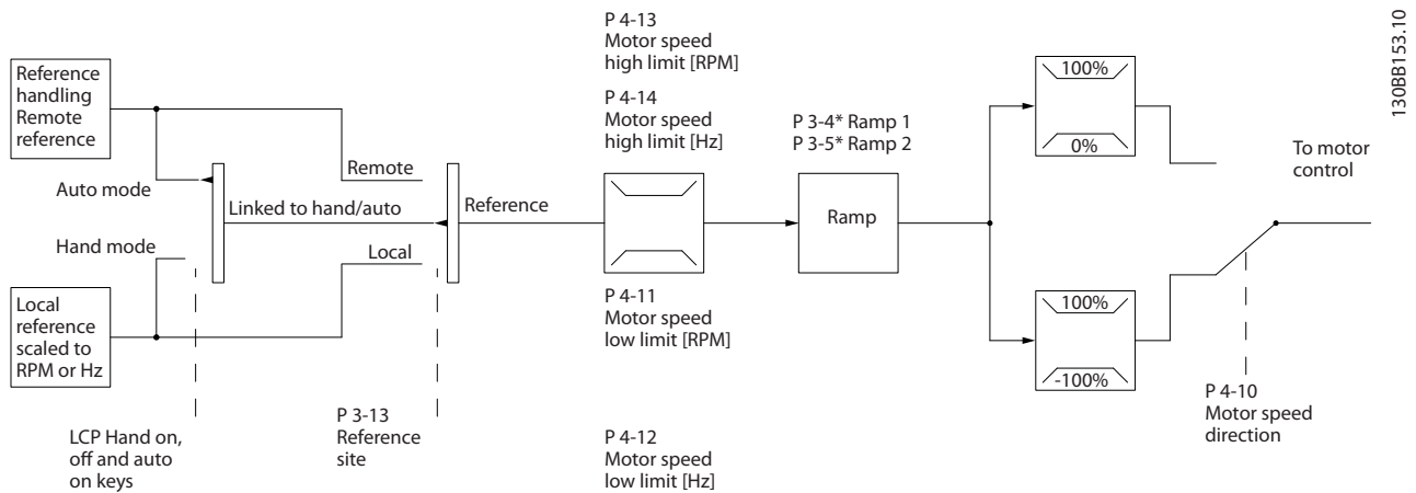
Ilustración 2.10 Estructura de lazo abierto
