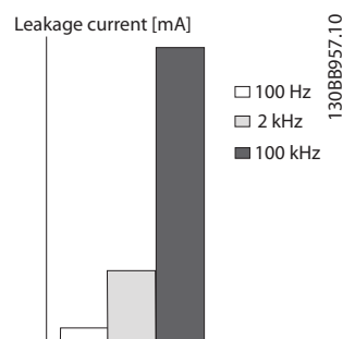
Ilustración 2.18 Esquema de principio que muestra cómo la frecuencia de corte del RCD influirá en la Respuesta/Medición.
