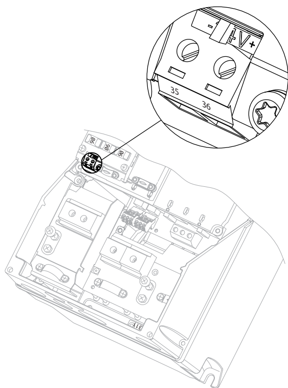
Ilustración 3.5 Conexión al suministro externo de 24 V (A5-C2).
