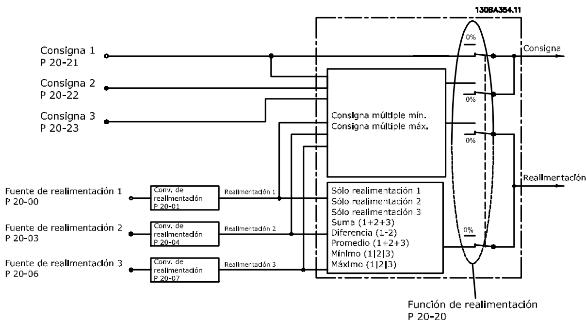
Ilustración 2.12 Diagrama de bloques de procesamiento de señal de realimentación
