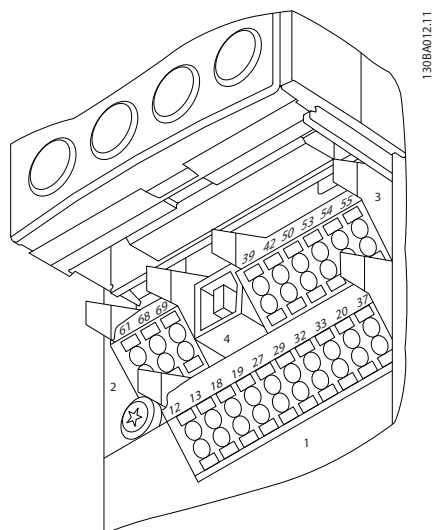
Ilustración 5.21 Terminales de control (todas las protecciones)
