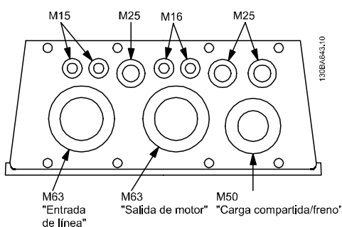
Ilustración 5.12 Orificios de entrada para cables en la protección C1. La utilización que se sugiere de los orificios es solo una recomendación. Son posibles otras soluciones.
