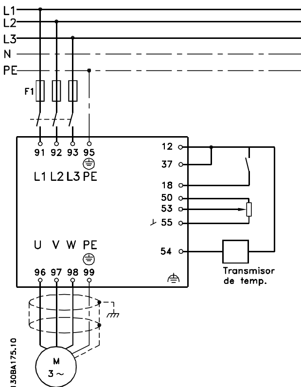
Ilustración 5.26 Diagrama de conexiones eléctricas.
