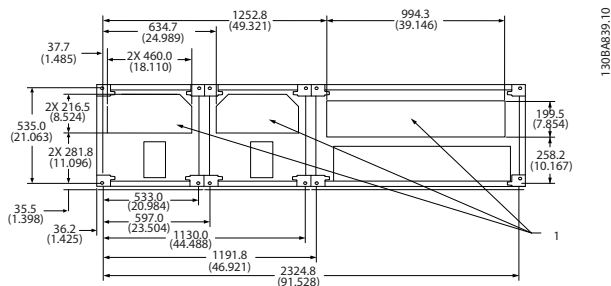
Ilustración 5.20 Tamaño del bastidor F4
