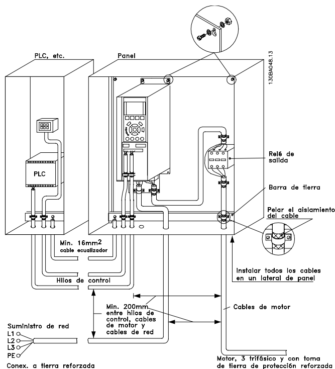
Ilustración 5.25 Instalación eléctrica correcta en cuanto a CEM de un Convertidor de frecuencia en el armario.
