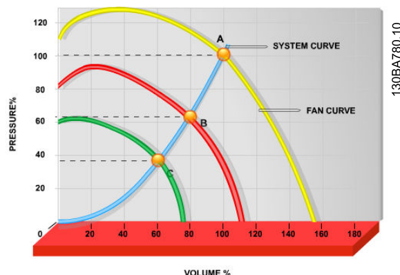
Ilustración 2.4 El gráfico muestra curvas de ventilador (A, B y C) para caudales bajos de ventilador.
