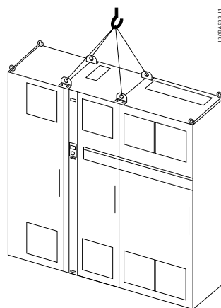
Ilustración 5.4 Método de elevación recomendado, tamaño del bastidor F3 (460 V, 600 a 900 CV, 575/690 V, 900 a 1150 CV).
