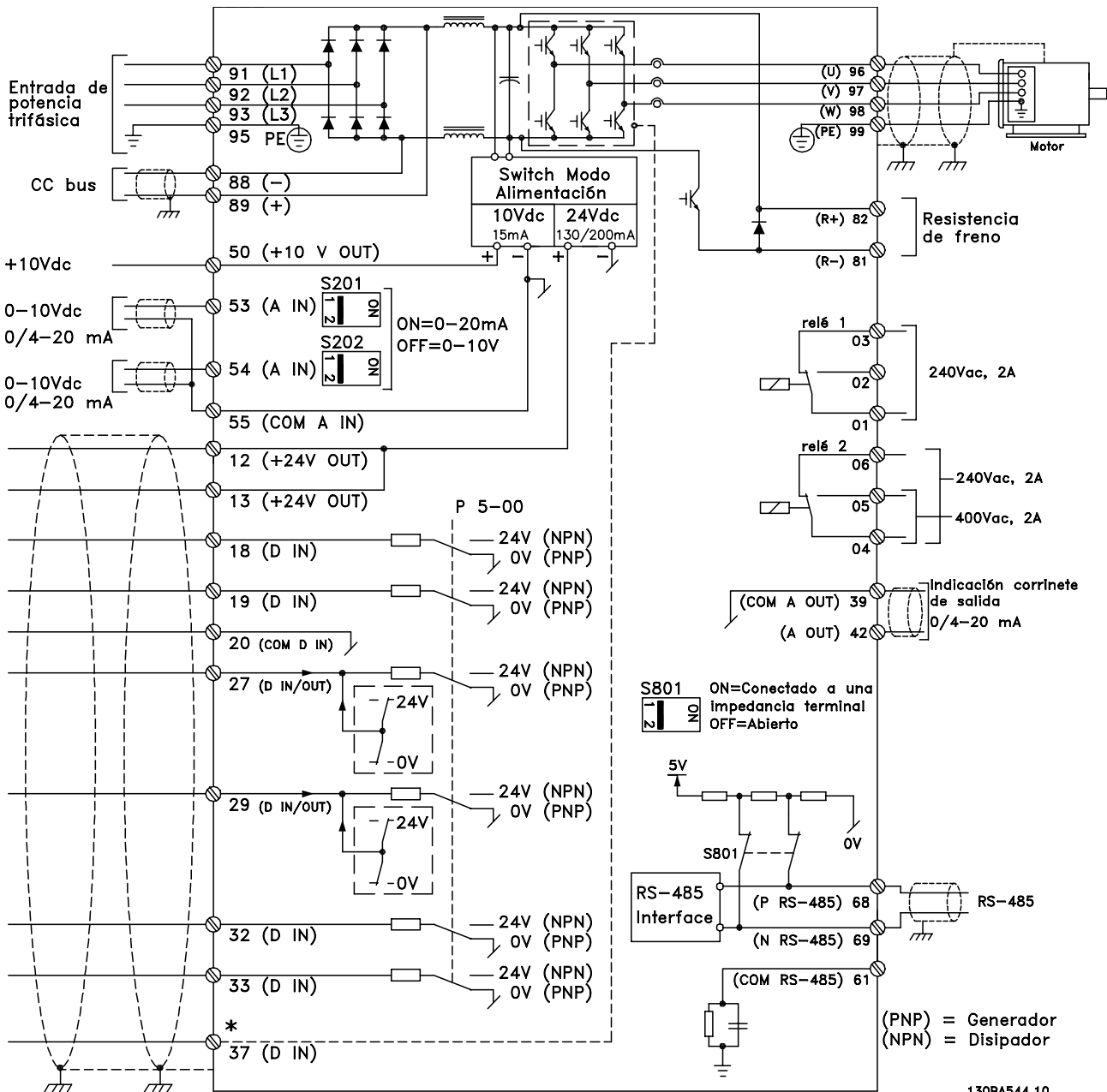
Ilustración 5.6 Diagrama que muestra todos los terminales eléctricos. (El terminal 37 solo está presente en unidades con función de parada de seguridad.)
