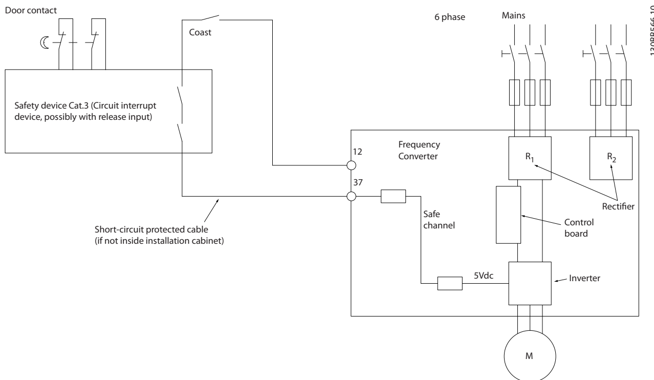
Ilustración 2.3 Ilustración de los aspectos esenciales de una instalación para lograr una parada de categoría 0 (EN 60204-1) con seguridad de categoría 3 (EN 954-1).
