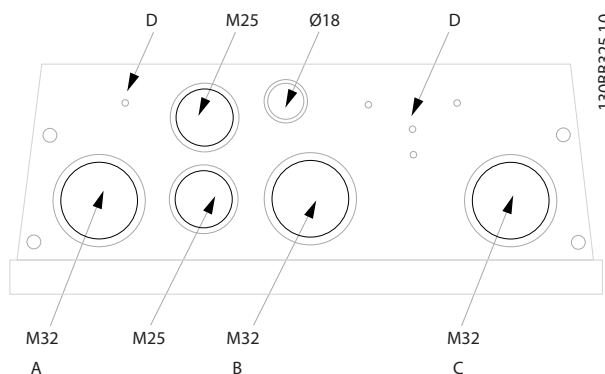
Ilustración 5.9 Orificios de entrada para cables en la protección B1. La utilización que se sugiere de los orificios es solo una recomendación. Son posibles otras soluciones.
