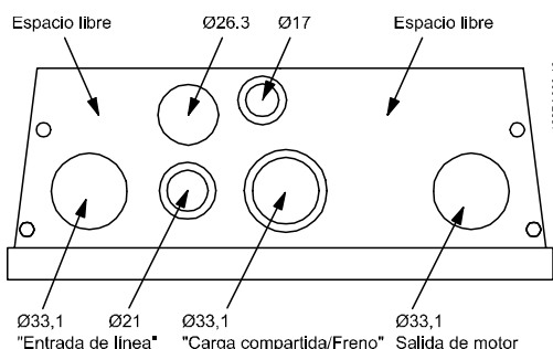
Ilustración 5.8 Orificios de entrada para cables en la protección B1. La utilización que se sugiere de los orificios es solo una recomendación. Son posibles otras soluciones.
