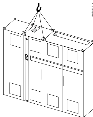
Ilustración 5.5 Método de elevación recomendado, tamaño del bastidor F4 (460 V, 1000 a 1200 CV, 575/690 V, 1250 a 1350 CV).
