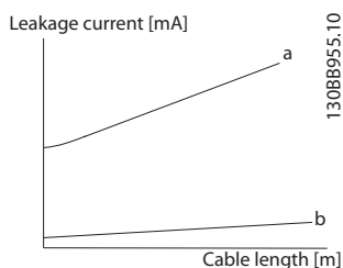
Ilustración 2.15 El esquema de principio muestra cómo la corriente de fuga depende de la longitud del cable y del tamaño de potencia. P_a > P_b .
