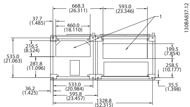
Ilustración 5.17 Tamaño del bastidor F1
