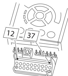
Ilustración 2.2 Puente de conexión entre el terminal 37 y 24 V CC.
