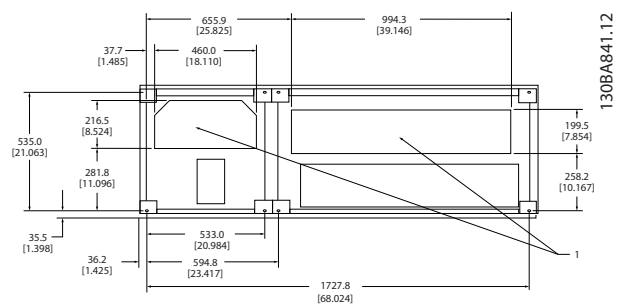
Ilustración 5.18 Tamaño del bastidor F2
