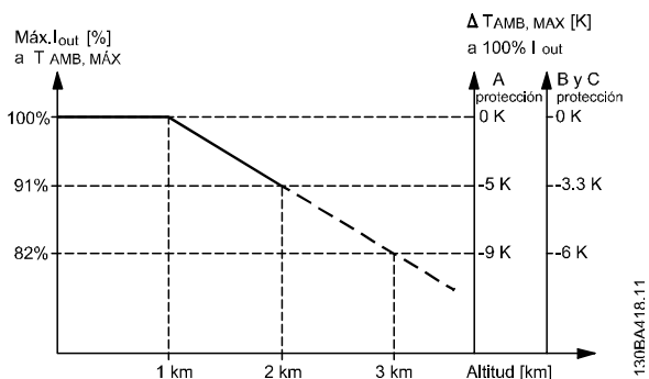
Ilustración 8.2 Reducción de intensidad de salida frente a la altitud a TAMB, MAX para tamaños de bastidor D, E y F. En altitudes superiores a 2 km, póngase en contacto con Danfoss en relación con PELV.
