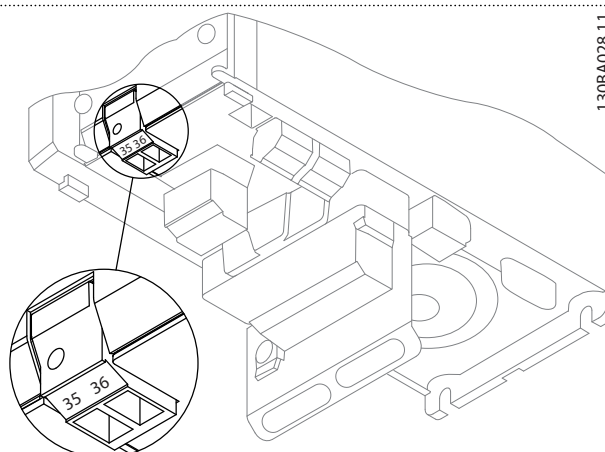
Ilustración 3.4 Conexión al suministro externo de 24 V (A2-A3).
