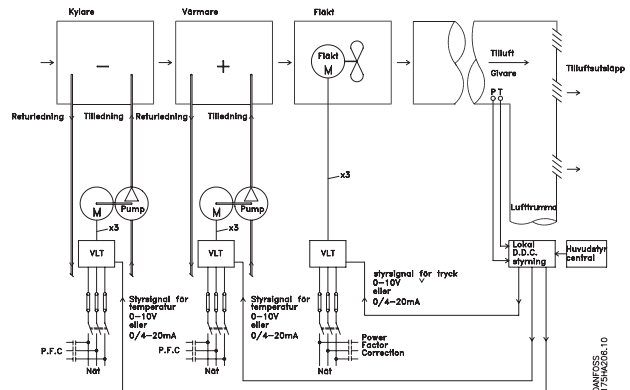
Bild 2.8 Bilden visar ett fläktsystem som styrs av frekvensomformare.
