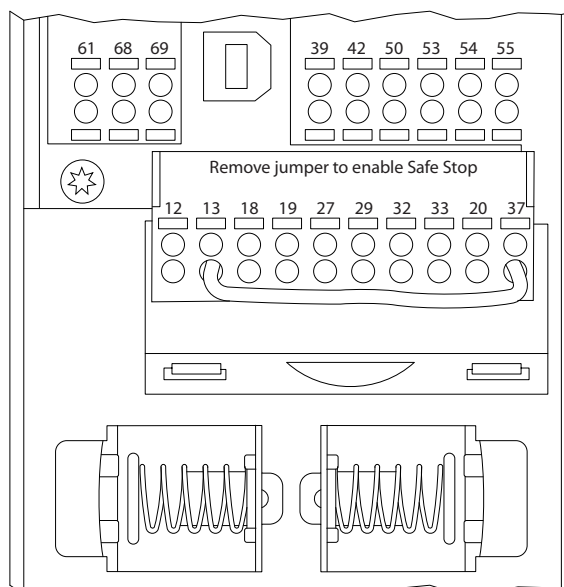
Bild 7.2 Plintar på styrkort
