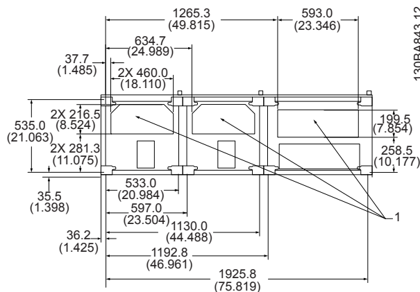
Bild 5.19 Ramstorlek F3
