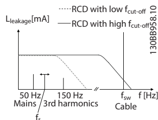
Bild 2.17 Skiss över de huvudsakliga bidragande faktorerna till läckström
