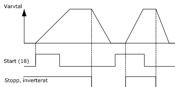
Bild 6.2 Plint 37: Endast tillgänglig med funktion för säkerhetsstopp
