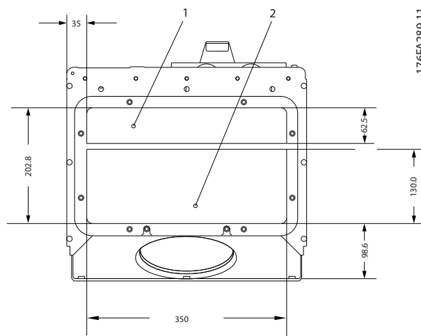
Bild 5.15 Ramstorlek D1 + D2
