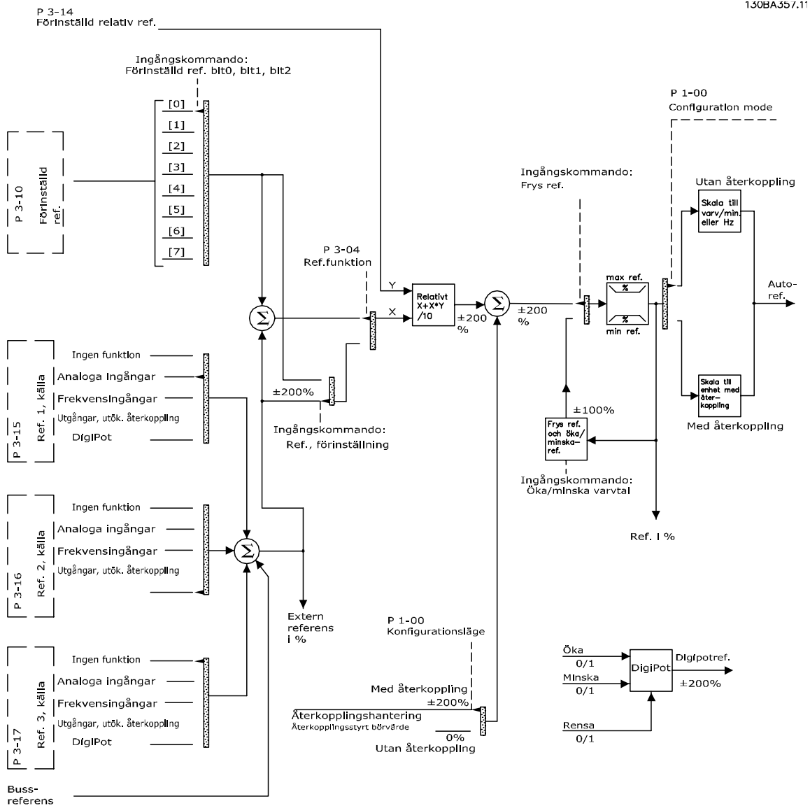
Bild 2.13 Blockdiagram som visar extern referens
