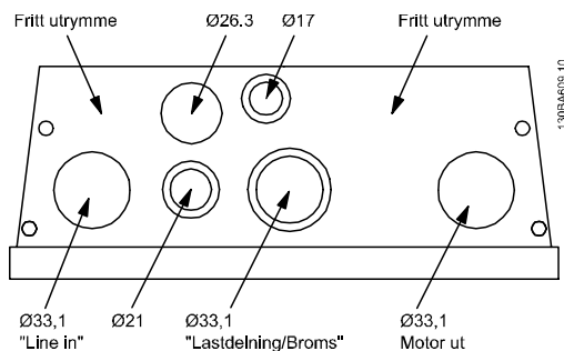
Bild 5.8 Kabelinföringshål för kapslingen B1. Den föreslagna användningen av hålen är enbart en rekommendation och andra lösningar kan vara möjliga.
