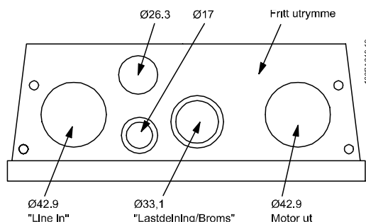
Bild 5.10 Kabelinföringshål för kapslingen B2. Den föreslagna användningen av hålen är enbart en rekommendation och andra lösningar kan vara möjliga.
