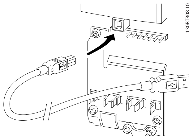
Bild 5.24 Mer information om styrkabelanslutningar finns i avsnittet Styrplintar .
