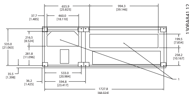
Bild 5.18 Ramstorlek F2
