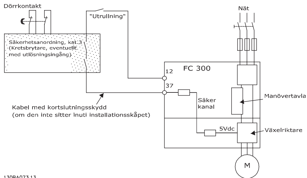
Bild 2.3 Bild av de viktigaste aspekterna av en installation för att uppnå en stoppkategori 0 (EN 60204-1) med säkerhetskategori 3 (EN 954-1).
