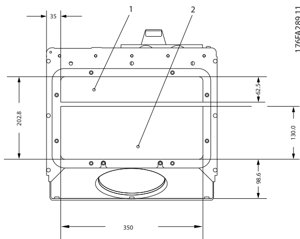
Bild 5.16 Ramstorlek E1
