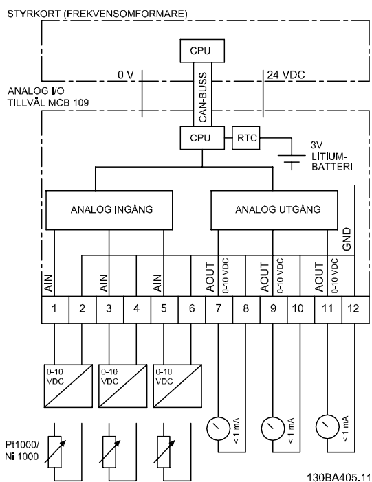
Bild 3.6 Principdiagram för analoga I/O som monterats i frekvensomformaren.
