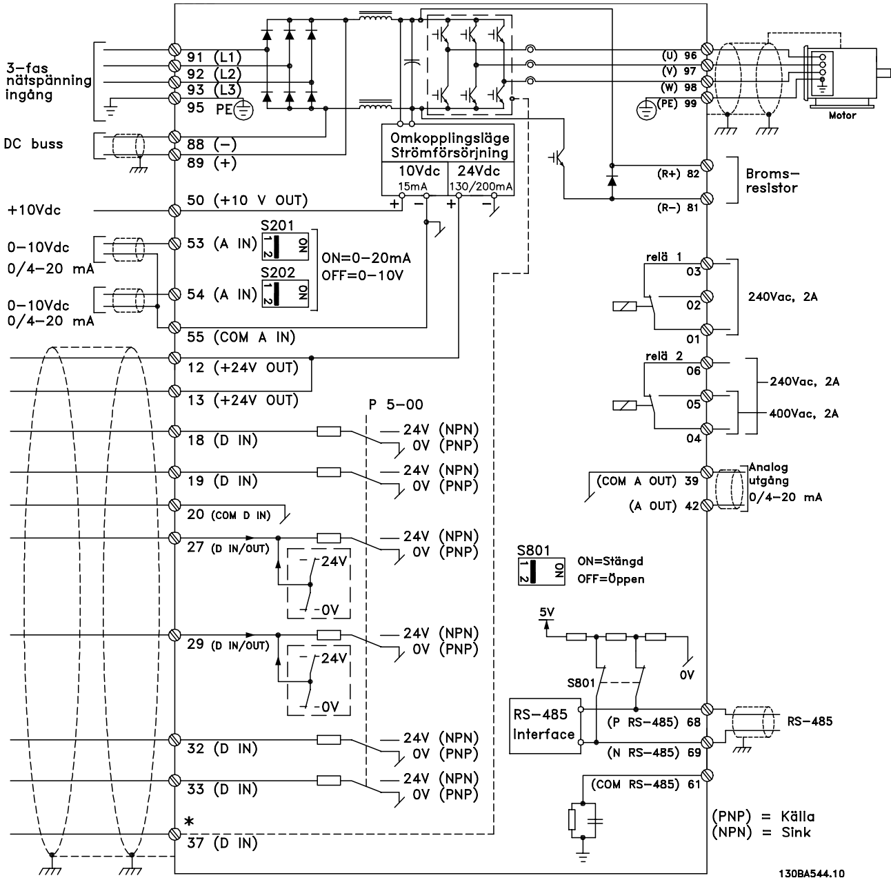
Bild 5.6 Diagram över alla elektriska plintar. (Plint 37 fungerar enbart med enheter som har funktionen säkerhetsstopp.)
