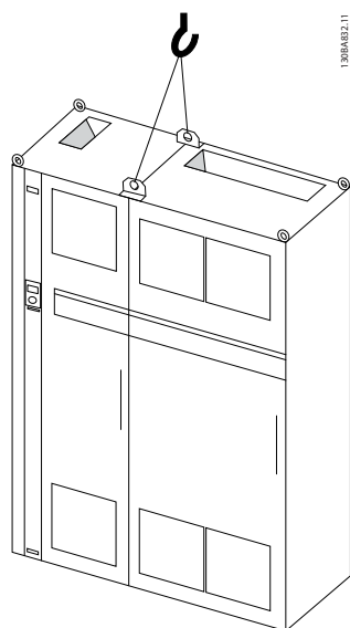
Bild 5.2 Rekommenderad lyftmetod, ramstorlek F1 (460 V, 600 till 900 HP, 575/690 V, 900 till 1 150 HP).
