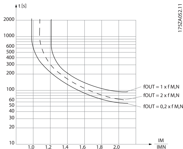
Bild 2.19 X-axeln visar förhållandet mellan I_{motor} och I_{motor} nominellt. Y-axeln visar tiden i sekunder innan ETR-reläet stängs av och trippar frekvensomformaren. Kurvorna visar det karakteristiska nominella varvtalet vid dubbla det nominella varvtalet och vid 0,2 x det nominella motorvarvtalet.
