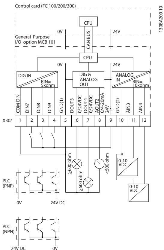
Bild 3.3 Kopplingschema
