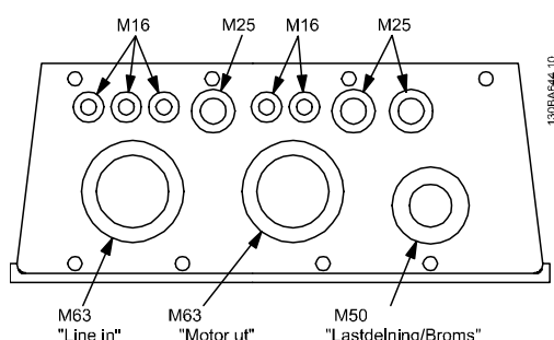
Bild 5.13 Kabelinföringshål för kapslingen C2. Den föreslagna användningen av hålen är enbart en rekommendation och andra lösningar kan vara möjliga.
