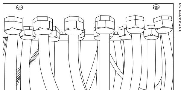
Bild 5.14 Exempel på korrekt installation av av boxplåten.
