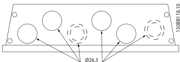
Bild 5.7 Kabelinföringshål för kapslingen A5. Den föreslagna användningen av hålen är enbart en rekommendation och andra lösningar kan vara möjliga.
