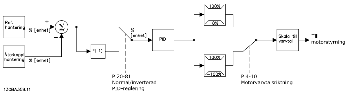
Bild 2.11 Blockdiagram över regulatorn med återkoppling
