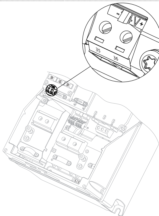
Bild 3.5 Anslutning till 24 V-reservförsörjningen (A5-C2).
