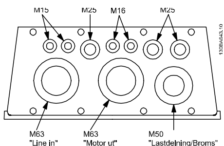
Bild 5.12 Kabelinföringshål för kapslingen C1. Den föreslagna användningen av hålen är enbart en rekommendation och andra lösningar kan vara möjliga.
