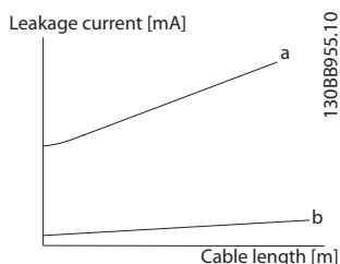
Bild 2.15 Principskiss som visar hur läckströmmen påverkas av kabellängden och storleken på strömmen. P_a > P_b .
