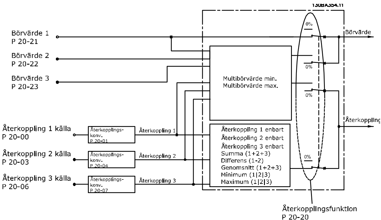
Bild 2.12 Blockdiagram över behandlingen av återkopplingssignalen
