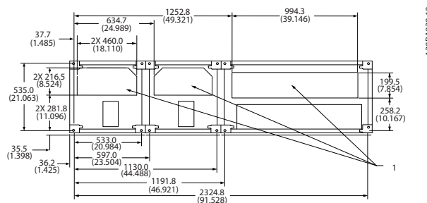
Bild 5.20 Ramstorlek F4
