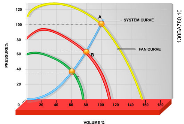
Bild 2.4 Diagrammet visar fläktkurvor (A, B och C) för reducerade fläktvolymmer.
