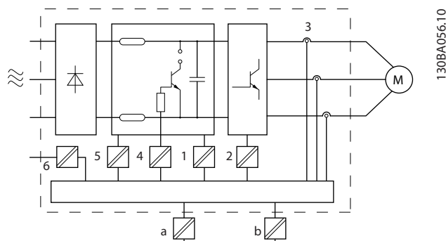
Bild 2.14 Galvanisk isolering
