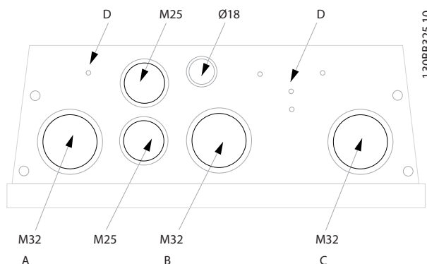
Bild 5.9 Kabelinföringshål för kapslingen B1. Den föreslagna användningen av hålen är enbart en rekommendation och andra lösningar kan vara möjliga.
