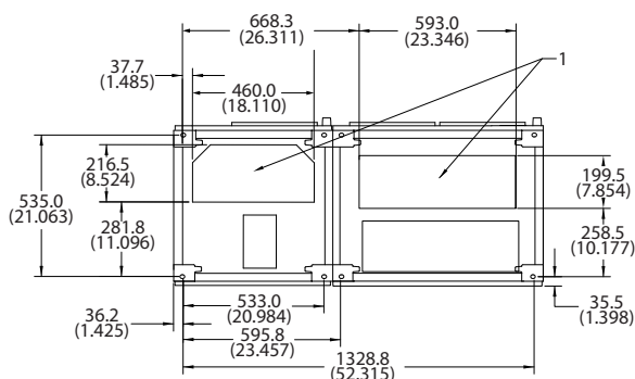
Bild 5.17 Ramstorlek F1
