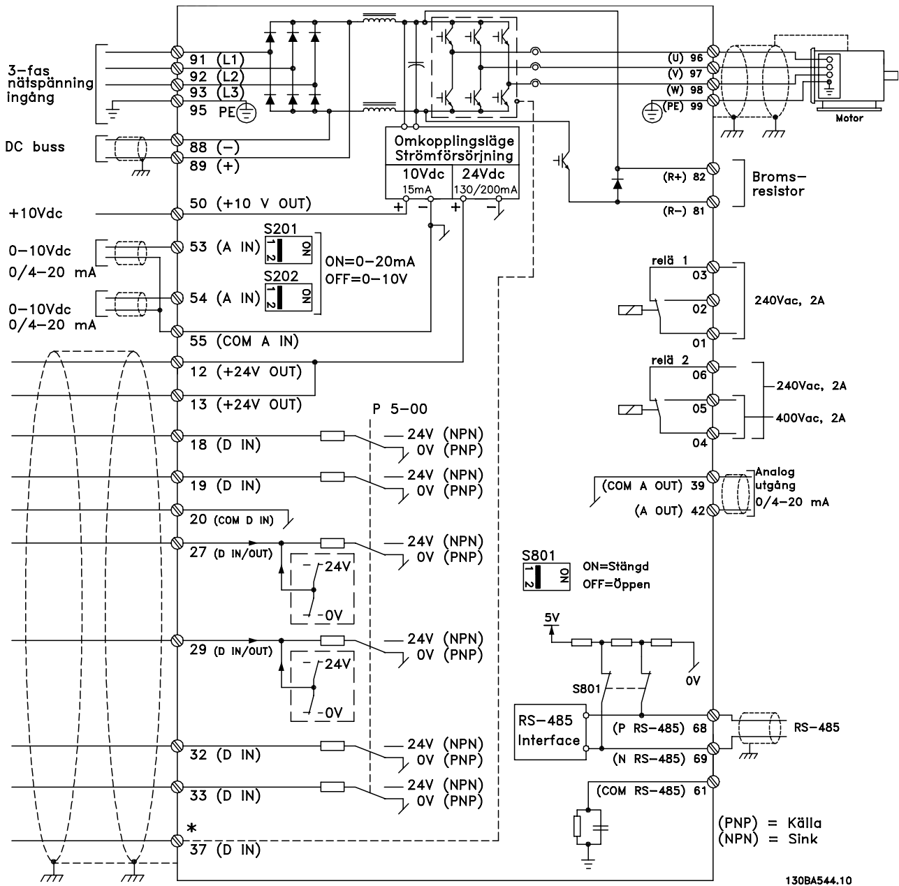
Bild 5.23 Diagram över alla elektriska plintar.
