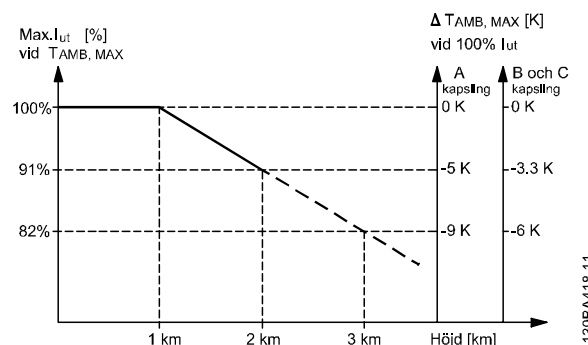
Bild 8.2 Nedstämpling av utström visavi höjd vid T_{AMB, MAX} för ramstorlekarna A, B och C. Kontakta Danfoss om PELV vid höjder över 2 km.
