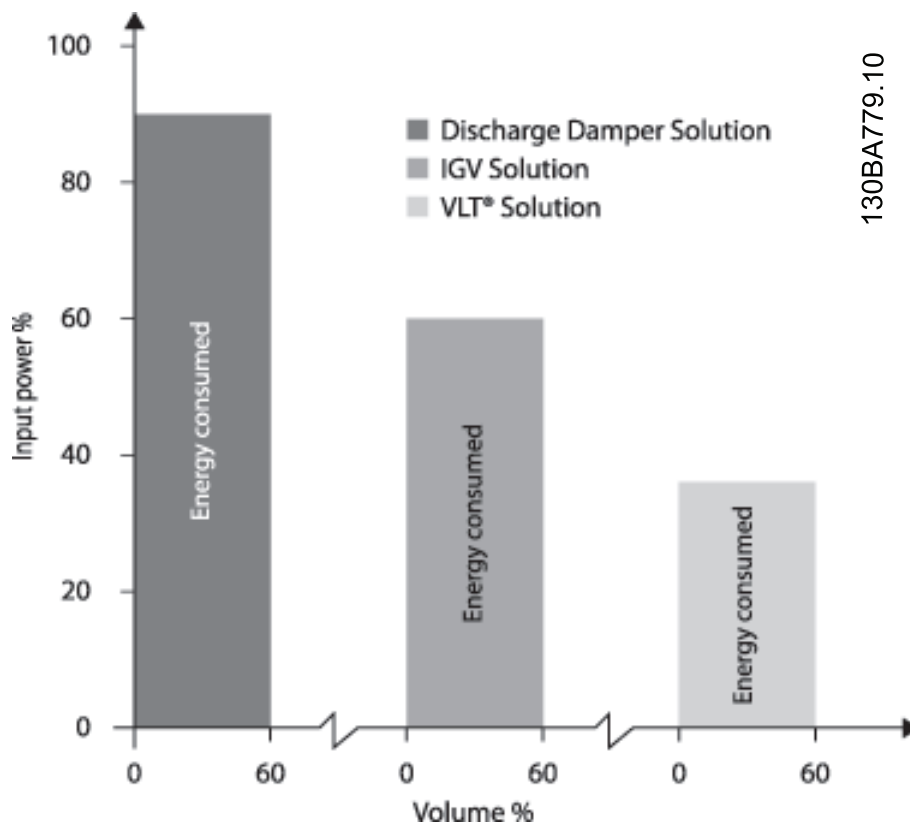
Bild 2.7 Utblåsdämpare reducerar strömförbrukningen något. Inlet Guide Vans ger en reduktion på 40 % men är dyra att installera. Lösningen med frekvensomformare från Danfoss minskar energiförbrukningen med mer än 50 % och är lätt att installera.
