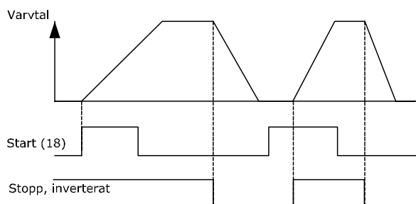
Bild 5.22 Plint 37 är endast tillgänglig med funktionen säkerhetsstopp!
