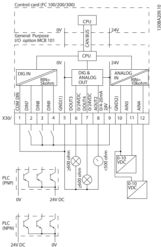
图 3.3 原理图
