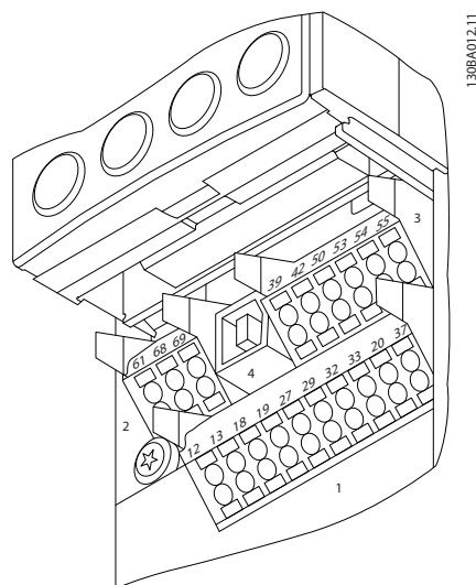
图 5.21 控制端子 (所有机箱)
