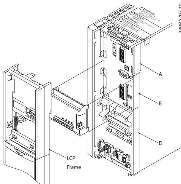
图 3.1 A2、A3 和 B3 机箱
