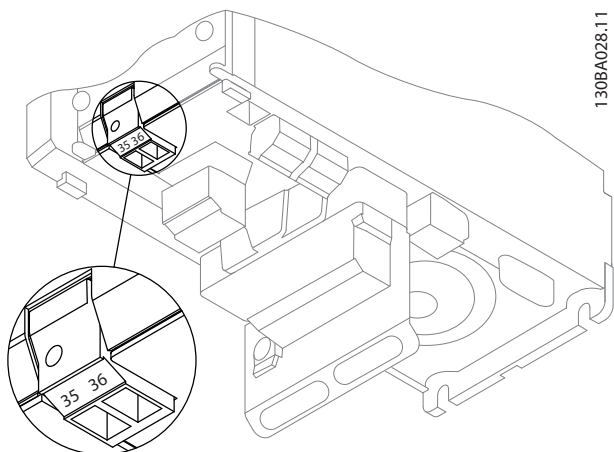
图 3.4 24V 备用电源的连接 (A2-A3)。
