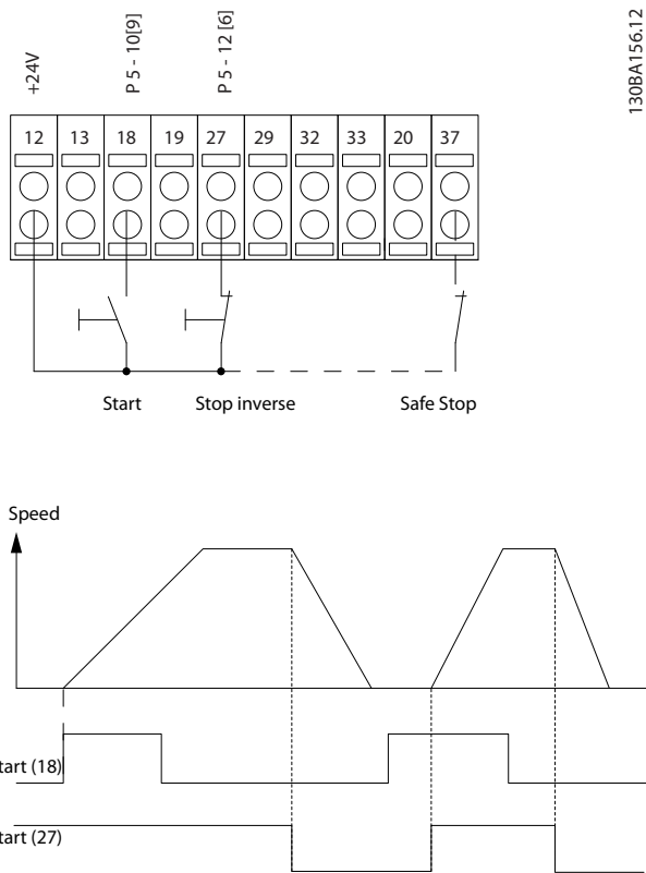
图 5.22 端子 37 仅随安全停止功能一起提供!
