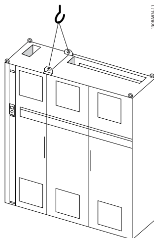
图 5.3 建议的起吊方法, 机架规格 F2 (460V, 1000 到 1200 HP; 575/690V, 1250 到 1350 HP)。
