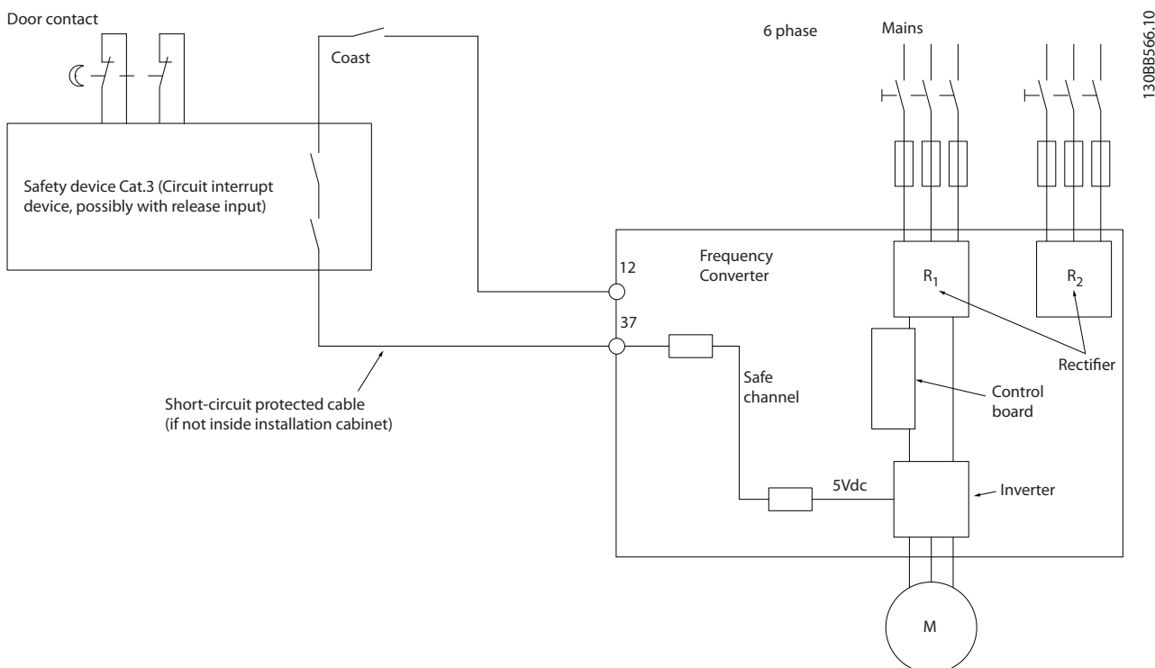
图 2.3 符合安全类别 3 (EN 954-1) 停止类别 0 (EN 60204-1) 的安装基本配置的简图。
