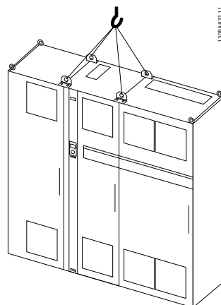
图 5.4 建议的起吊方法, 机架规格 F3 (460V, 600 到 900 HP; 575/690V, 900 到 1150 HP)。
