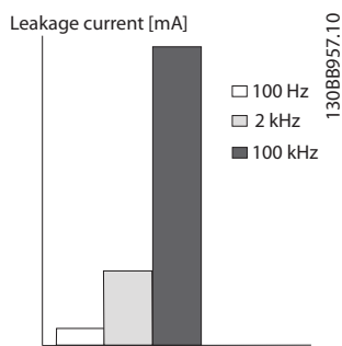
图 2.18 原理图显示了 RCD 的截止频率将会如何影响需要对何对象作出响应/测量。
