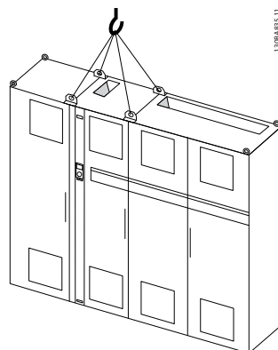
图 5.5 建议的起吊方法, 机架规格 F4 (460V, 1000 到 1200 HP; 575/690V, 1250 到 1350 HP)。
