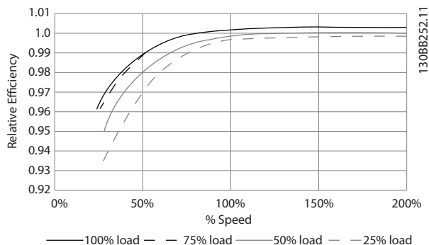
图 8.1 典型效率曲线
