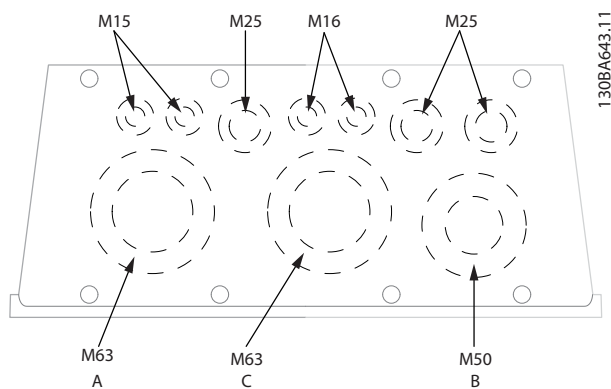
图 5.12 机箱 C1 的电缆入口。入口的用途仅为建议，您也可以采用其它方案。
