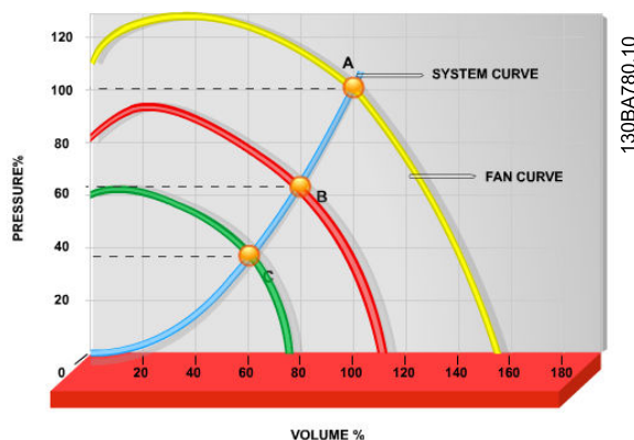
图 2.4 下图显示了降低风扇容量时的风扇曲线 (A、B 和 C)。
