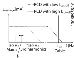
图 2.17 漏电电流主要成分示意图
