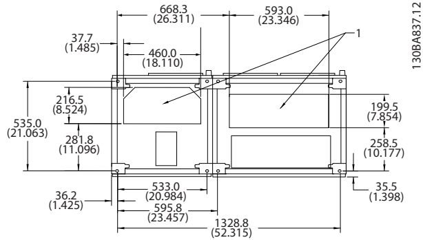
图 5.17 机架规格 F1
