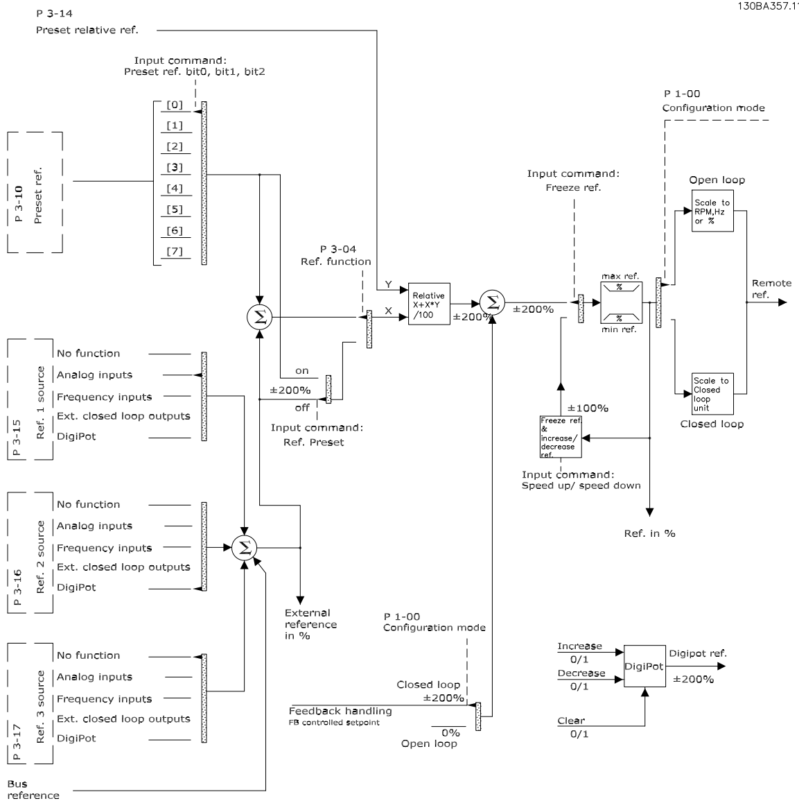
图 2.13 框图显示了远程参考值
