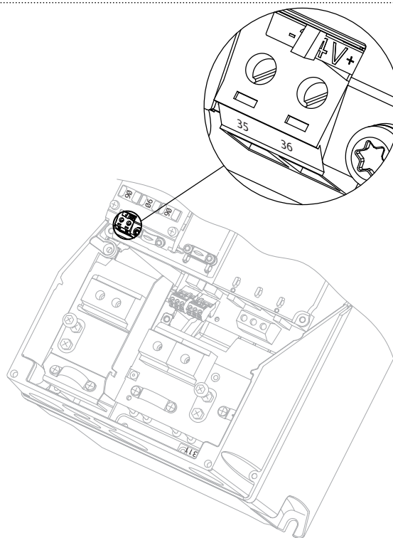
图 3.5 24V 备用电源的连接 (A5-C2)。
