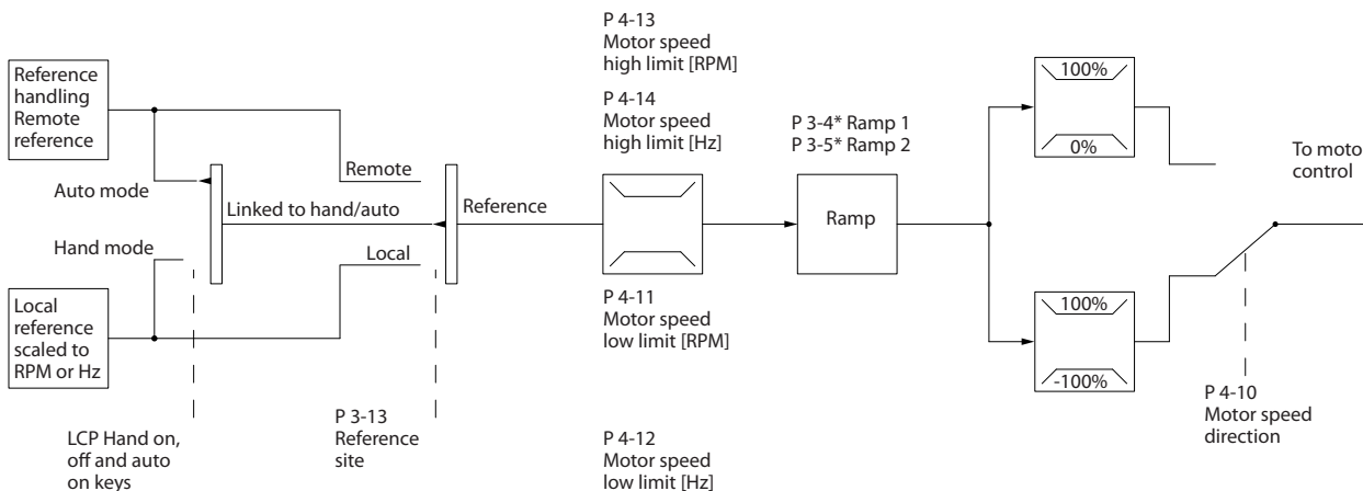
图 2.10 开环结构。
