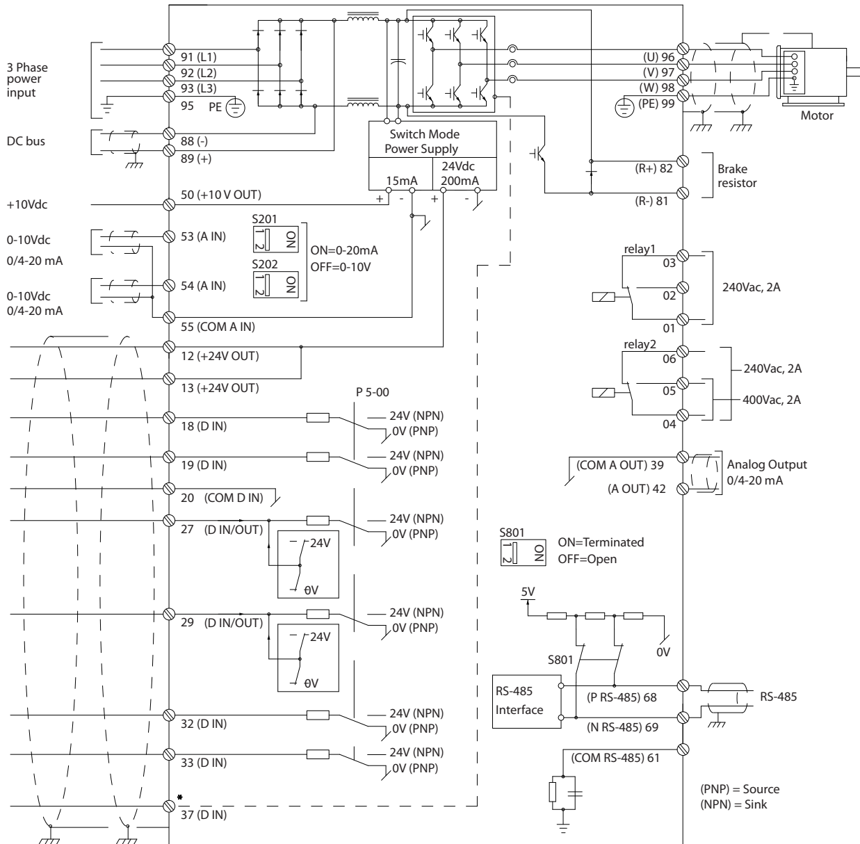
图 5.23 图中显示了所有电气端子。
