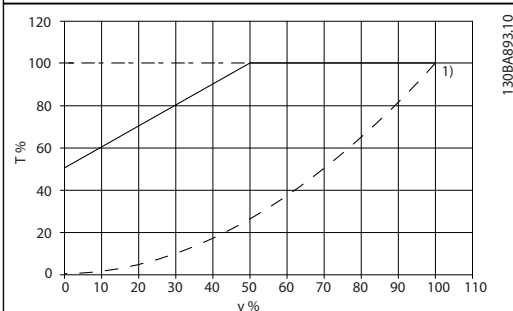
图例 ---VT 负载下的典型转矩 - - - - - 带强制冷却时的最大转矩 ——最大转矩
