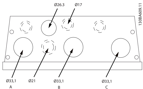
图 5.8 机箱 B1 的电缆入口。入口的用途仅为建议，您也可以采用其它方案。
