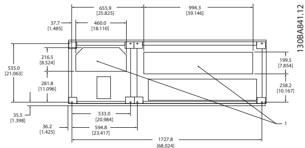
图 5.18 机架规格 F2
