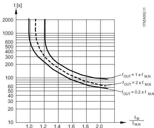
图 2.19 X 轴显示了 I_{motor} 和额定 I_{motor} 的比。Y 轴显示了 ETR 在使变频器断开并跳闸之前的时间 (秒)。曲线显示了额定速度下、2 倍额定速度下以及 0.2 倍额定速度下的特性。
