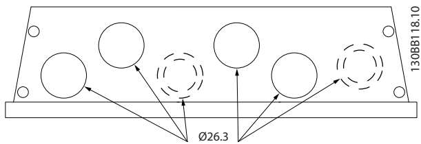
图 5.7 机箱 A5 的电缆入口。入口的用途仅为建议，您也可以采用其它方案。
