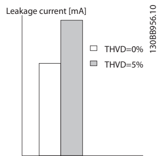
图 2.16 原理图显示了漏电电流将会如何受线路失真的影响。
