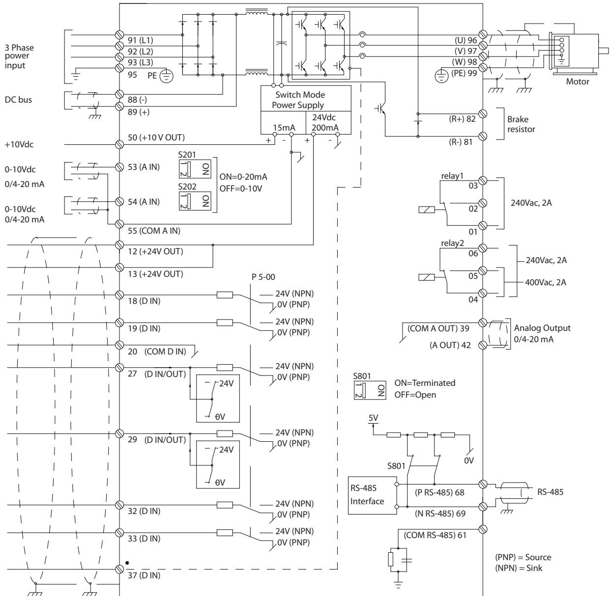
图 5.6 图中显示了所有电气端子。（仅带有安全停止功能的设备才提供端子 37。）
