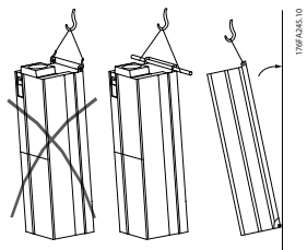
图 5.1 机架规格 D 和 E 的建议起吊方法。
