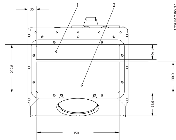
图 5.15 机架规格 D1 + D2
