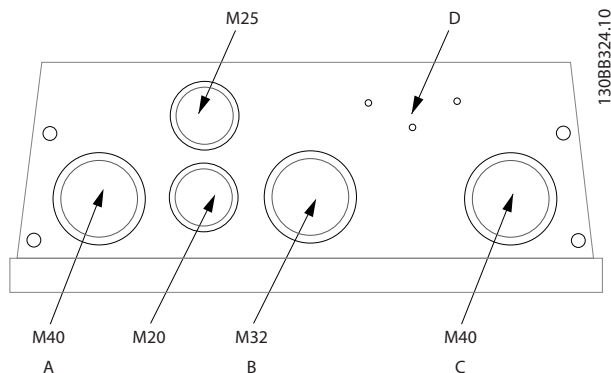
图 5.11 机箱 B2 的电缆入口。入口的用途仅为建议，您也可以采用其它方案。
