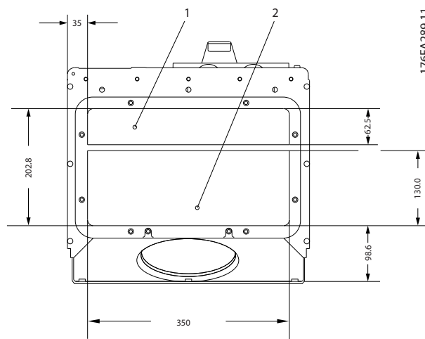
图 5.16 机架规格 E1
