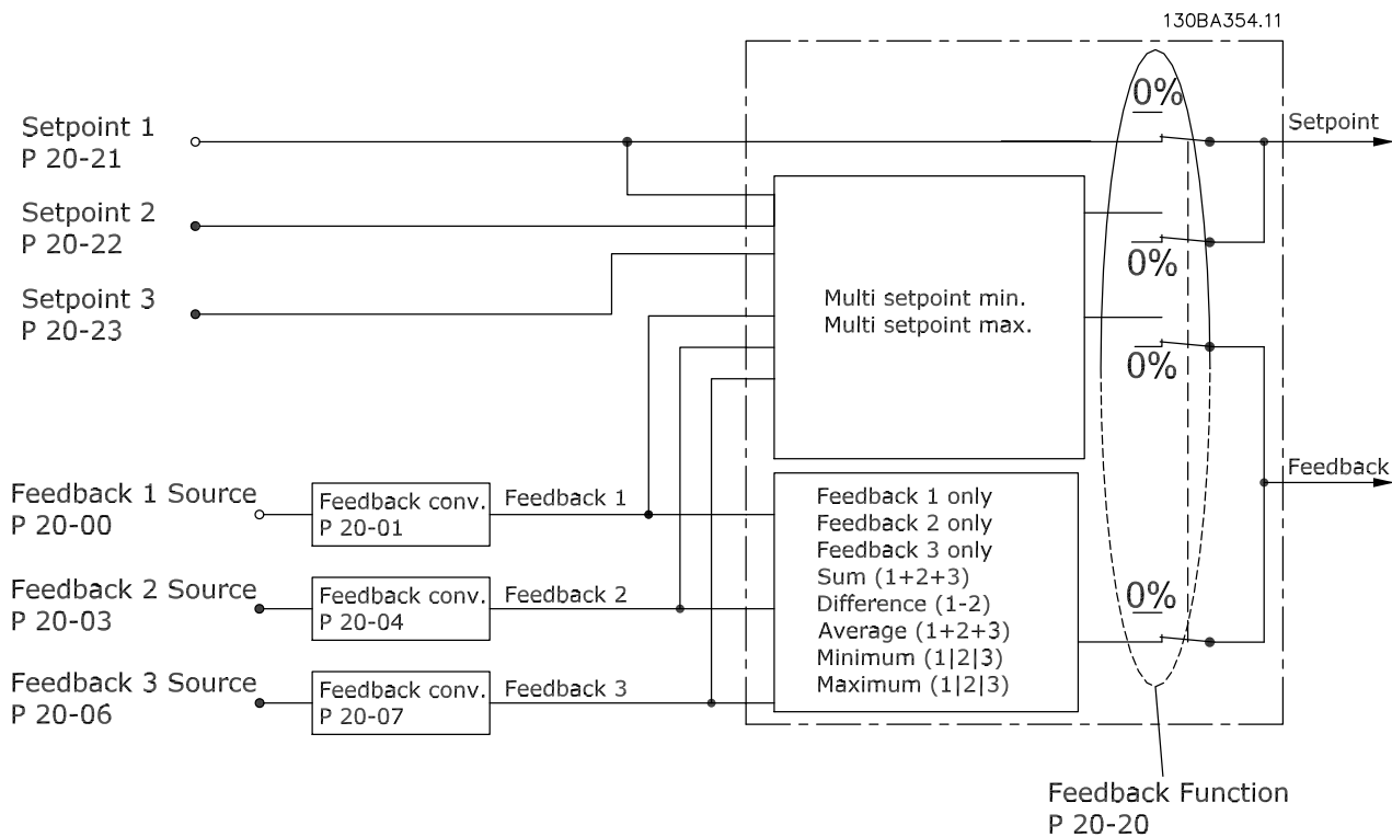
图 2.12 反馈信号处理框图
