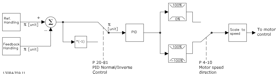
图 2.11 闭环控制器框图
