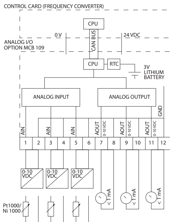
图 3.6 安装在变频器中的模拟输入输出的原理图。
