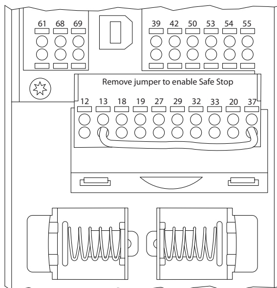
图 7.2 控制卡端子
