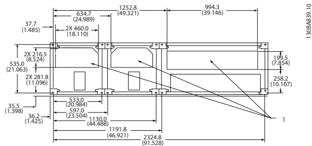
图 5.20 机架规格 F4
