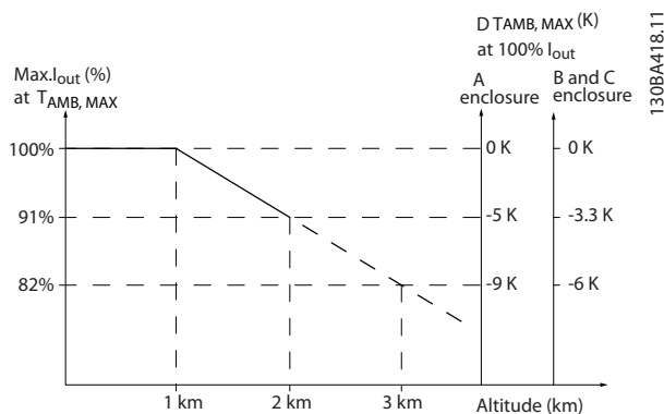
图 8.2 在 T AMB, MAX 下，输出电流降容与海拔的关系（机架规格 A、B 和 C）。当海拔超过 2 km 时，请向 Danfoss 咨询 PELV 事宜。
