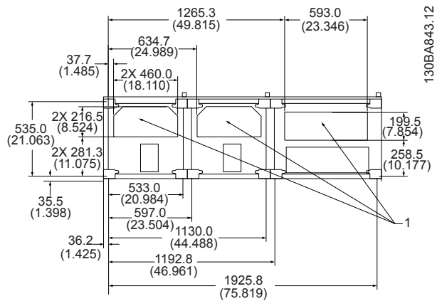
图 5.19 机架规格 F3
