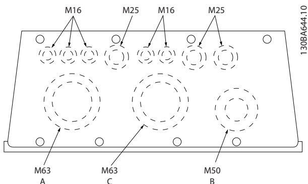
图 5.13 机箱 C2 的电缆入口。入口的用途仅为建议，您也可以采用其它方案。
