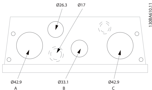
图 5.10 机箱 B2 的电缆入口。入口的用途仅为建议，您也可以采用其它方案。
