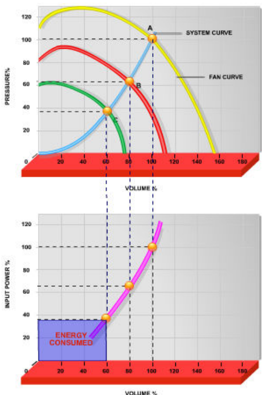
图 2.5 使用变频器将风扇容量降低到 60% 时，在通常应用中可以达到超过 50% 的能量节省。
