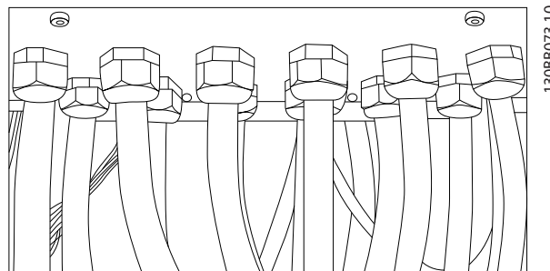
图 5.14 正确安装密封板的示例。
