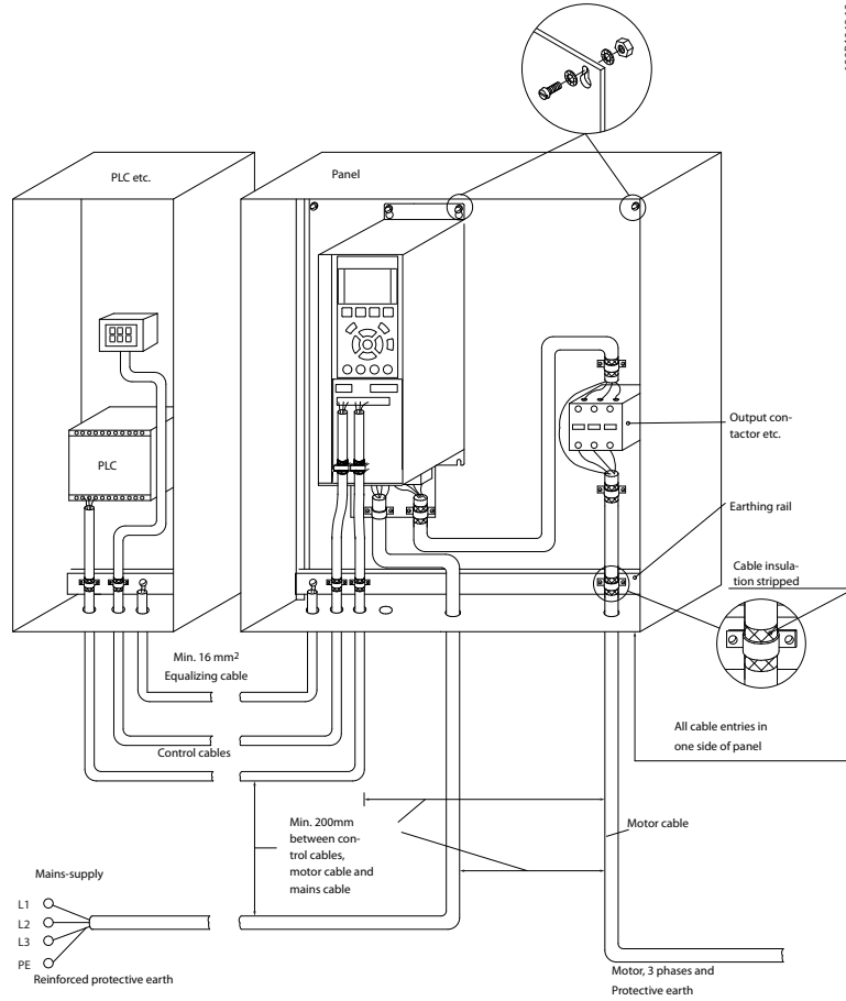
图 5.25 在机柜中对变频器执行符合 EMC 规范的电气安装。
