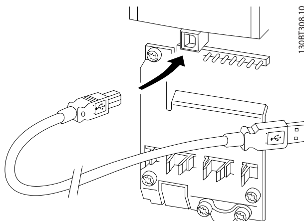
图 5.24 有关控制电缆连接的信息，请参阅有关控制端子的章节。
