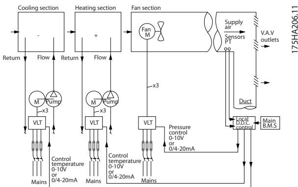
图 2.8 该图显示了一个由变频器控制的鼓风机系统。
