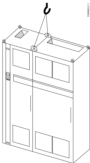
图 5.2 建议的起吊方法, 机架规格 F1 (460V, 600 到 900 HP; 575/690V, 900 到 1150 HP)。
