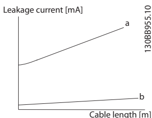
图 2.15 原理图显示了漏电电流将会如何受电缆长度和功率规格的影响。Pa > Pb。
