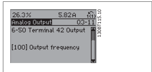
그림 1.12: 6단계: 파라미터 6-50 단자 42 출력을 선택합니다. [OK] 키를 누릅니다.
