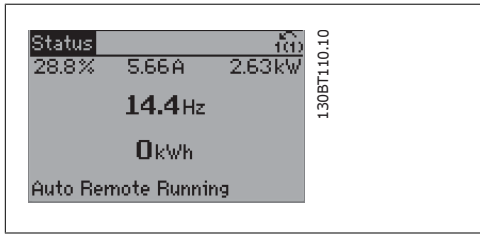
그림 1.7: 1단계: 주파수 변환기의 전원을 켭니다 (황색 LED 가 켜집니다).
