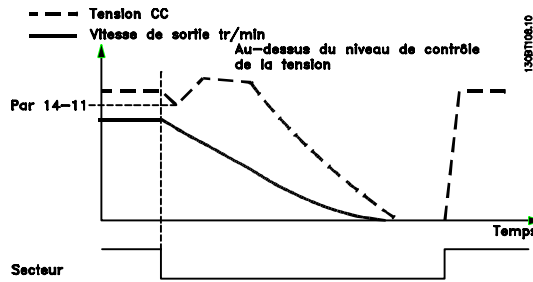
Illustration 3.3: Décélération contrôlée - Panne secteur plus longue. Décélération tant que l'énergie du système le permet, puis mise en roue libre du moteur.
