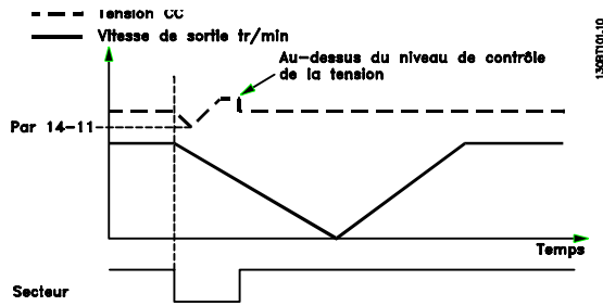
Illustration 3.2: Décélération contrôlée - Brève panne de secteur. Décélération jusqu'à l'arrêt, puis accélération jusqu'à la référence.
