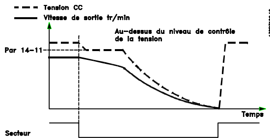
Illustration 3.5: Sauvegarde cinétique - Panne secteur plus longue. Le moteur est en roue libre dès que l'énergie du système est trop basse.
