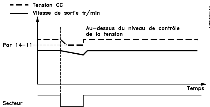
Illustration 3.4: Sauvegarde cinétique - Brève panne de secteur. Fonctionnement tant que l'énergie du système le permet.
