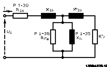
Afbeelding 3.1: Motorequivalentiediagram voor een asynchrone motor
