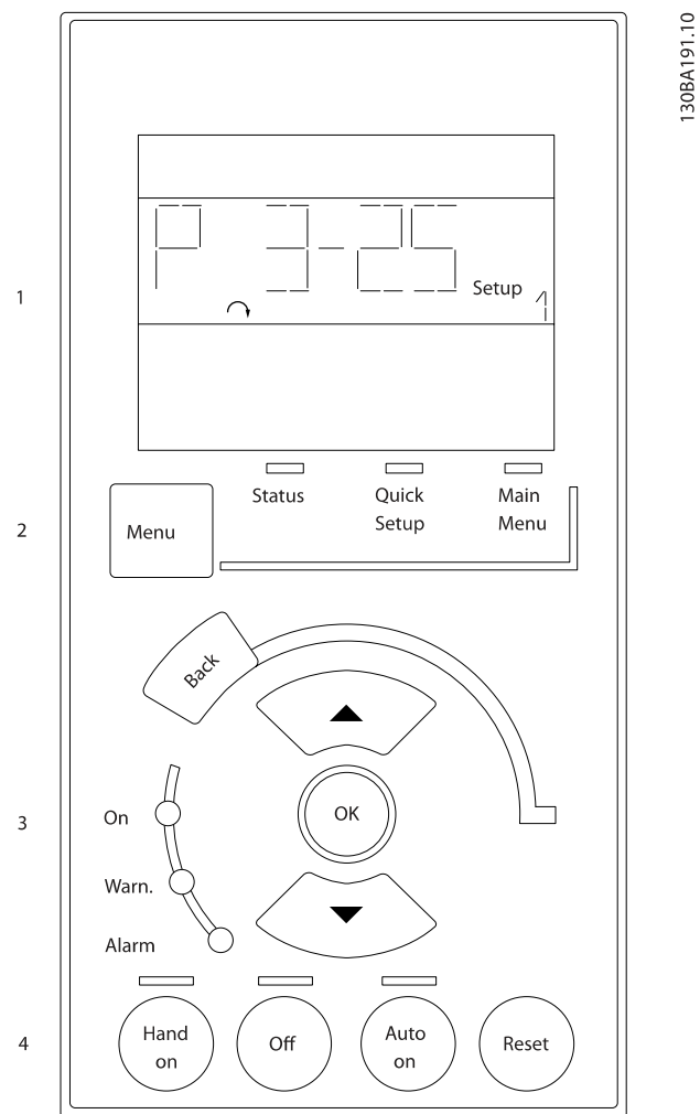
Abbildung 2.1: Numerische LCP Bedieneinheit LCP 101
