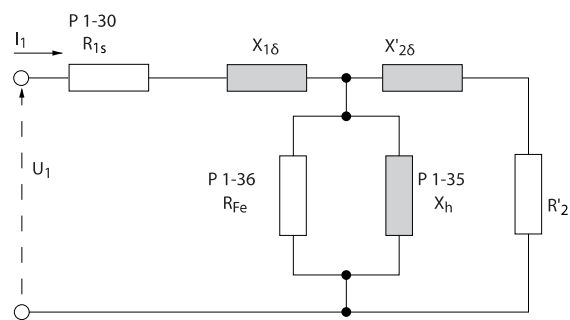
Ilustración 3.1: Diagrama equivalente del motor para un motor asíncrono
