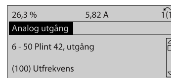
Bild 2.11: Steg 6: Välj par. 6-50. Tryck på [OK].
