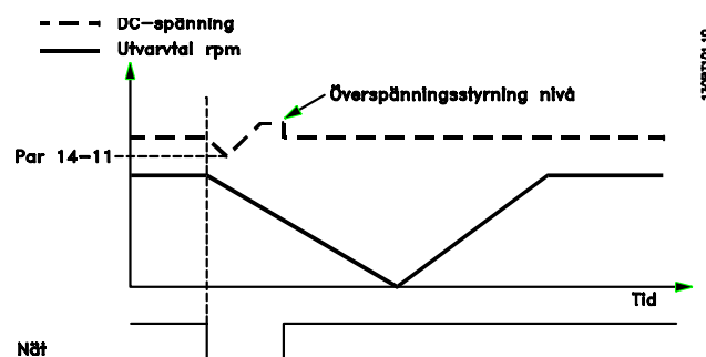
Bild 3.2: Kontrollerad nedrampning - kortslutningsfel i nätet. Nedrampning till stopp följt av upprampning till referens.
