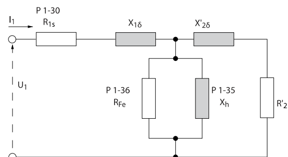
Bild 3.1: Motsvarande diagram för en asynkronmotor
