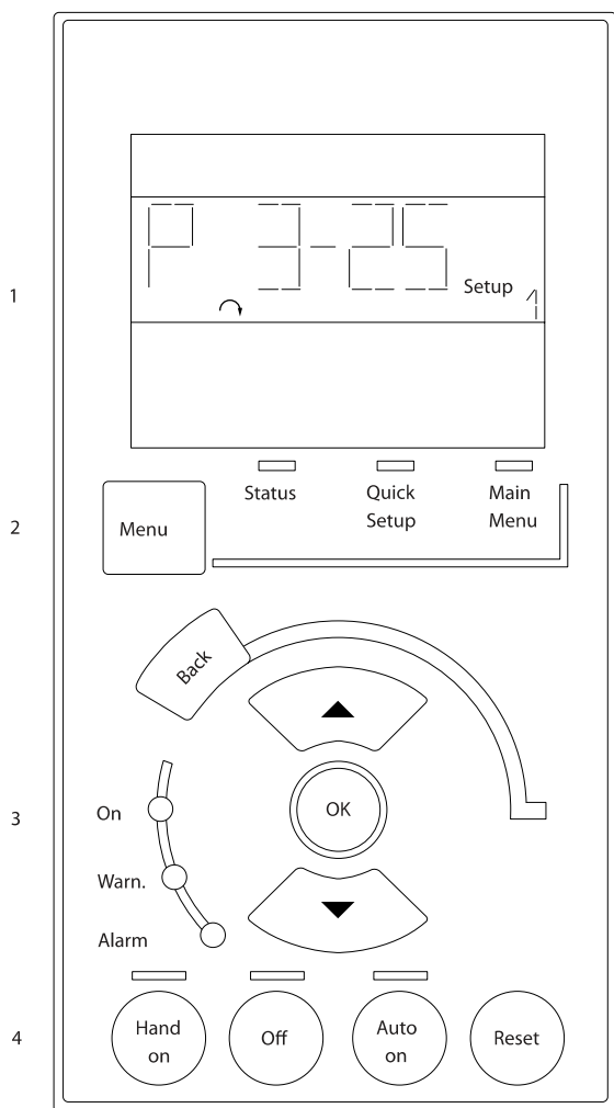
Afbeelding 2.1: Numeriek LCP (NLCP)
