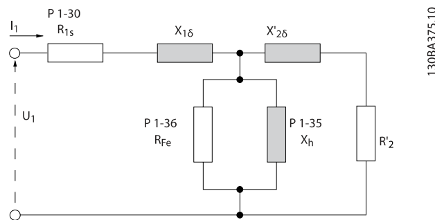
Afbeelding 3.1: Motorequivalentiediagram voor een asynchrone motor
