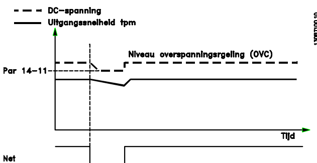
Afbeelding 3.4: Kinetische backup – korte netstoring. Doorgaan zolang de energie in het systeem dit toelaat.
