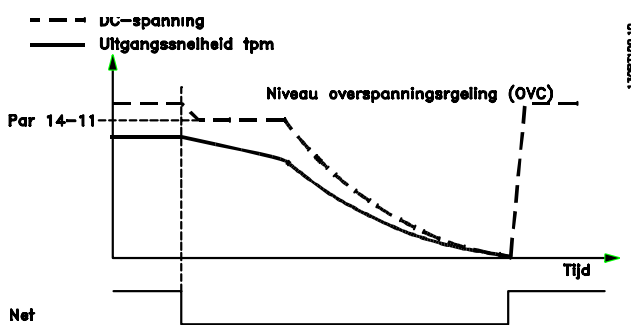
Afbeelding 3.5: Kinetische backup – langere netstoring. De motor zal gaan vrijlopen zodra de energie in het systeem te laag wordt.
