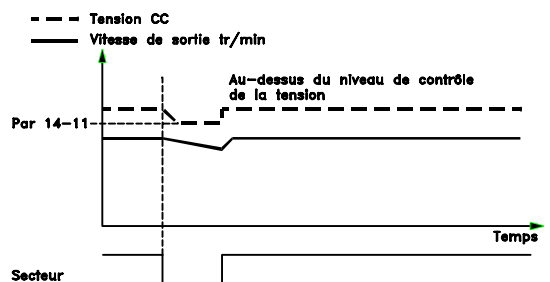
Illustration 3.4 Sauvegarde cinétique - Brève panne de secteur. Fonctionnement tant que l'énergie du système le permet.
