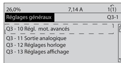
Illustration 2.10 Étape 5 : utiliser les touches de navigation haut/bas pour défiler vers le bas p. ex. jusqu'à Q3-11 Sorties ANA. Appuyer sur [OK].
