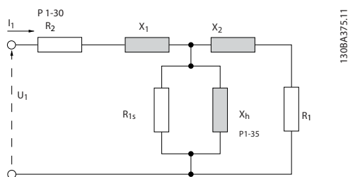
Illustration 3.1 Diagramme d'équivalence moteur pour un moteur asynchrone
