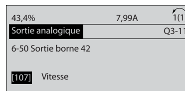
Illustration 2.12 Étape 7 : utiliser les touches de navigation haut/bas pour se déplacer parmi les différents choix. Appuyer sur [OK].
