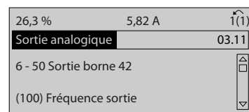
Illustration 2.11 Étape 6 : choisir le par. 6-50. Appuyer sur [OK].
