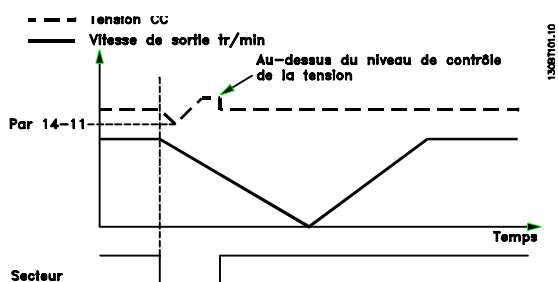
Illustration 3.2 Rampe de décélération contrôlée - brève panne de secteur Rampe de décélération jusqu'à l'arrêt, puis rampe d'accélération jusqu'à la référence.
