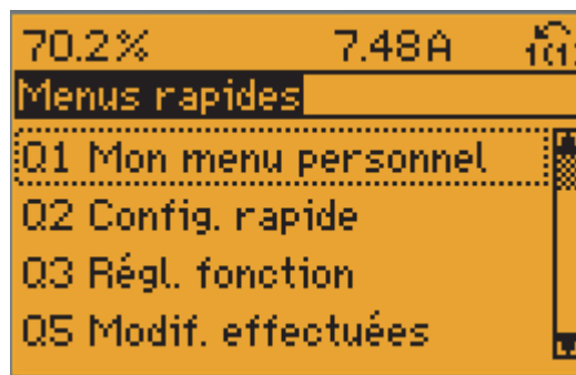
Illustration 2.5 Affichage du menu rapide.
