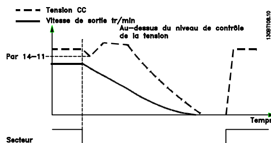
Illustration 3.3 Rampe de décélération contrôlée - panne secteur plus longue Rampe de décélération tant que l'énergie du système le permet, puis mise en roue libre du moteur.
