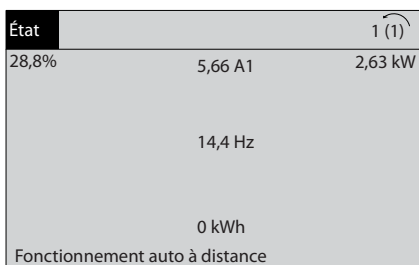
Illustration 2.6 Étape 1 : mettre le variateur de fréquence sous tension (voyant jaune allumé).
