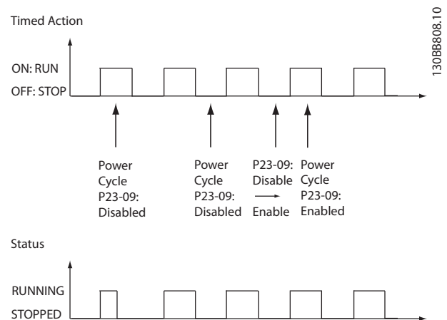
Afbeelding 3.6 Schema reactiveringstest
