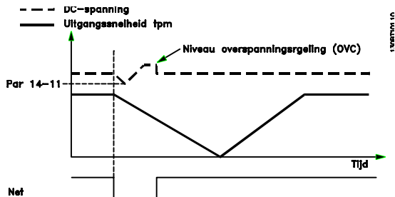
Afbeelding 3.2 Gecontroleerde uitloop – korte netstoring. Uitlopen tot stop gevolgd door aanlopen tot referentie.
