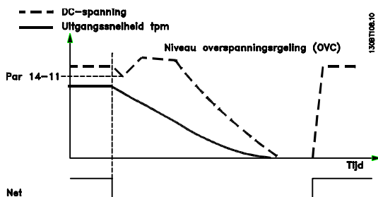
Afbeelding 3.3 Gecontroleerde uitloop – langere netstoring. Uitlopen zolang de energie in het systeem dit toelaat; vervolgens zal de motor vrijlopen.
