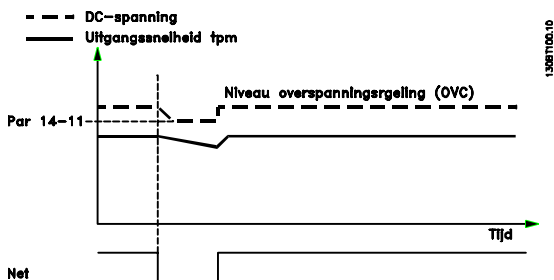
Afbeelding 3.4 Kinetische backup – korte netstoring. Doorgaan zolang de energie in het systeem dit toelaat.
