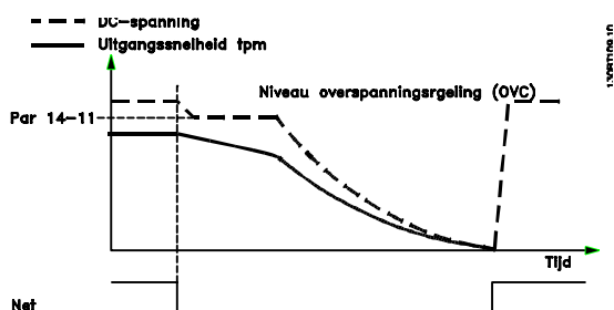
Afbeelding 3.5 Kinetische backup – langere netstoring. De motor zal gaan vrijlopen zodra de energie in het systeem te laag wordt.
