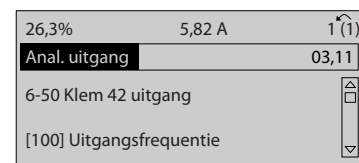
Afbeelding 2.11 Stap 6: Selecteer par. 6-50. Druk op [OK].
