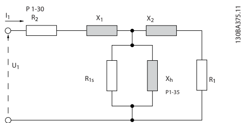
Afbeelding 3.1 Motorequivalentiediaagram voor een asynchrone motor
