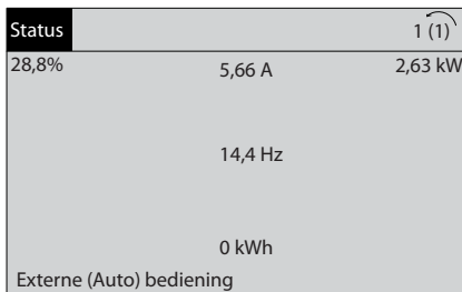
Afbeelding 2.6 Stap 1: Schakel de frequentieomvormer in (gele led gaat branden).
