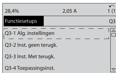
Afbeelding 2.9 Stap 4: De Functiesetupopties worden weergegeven. Selecteer Q3-1 Alg. instellingen . Druk op [OK].
