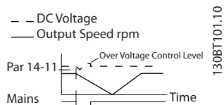
Рисунок 3.2 Управляемое замедление - короткое замыкание сети. После замедления и остановки следует разгон до заданного значения.
