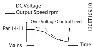
Рисунок 3.5 Кинетический резерв, более длительное замыкание сети. Двигатель останавливается выбегом, как только энергия в системе падает слишком низко.
