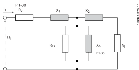
Рисунок 3.1 Эквивалентная схема асинхронного двигателя
