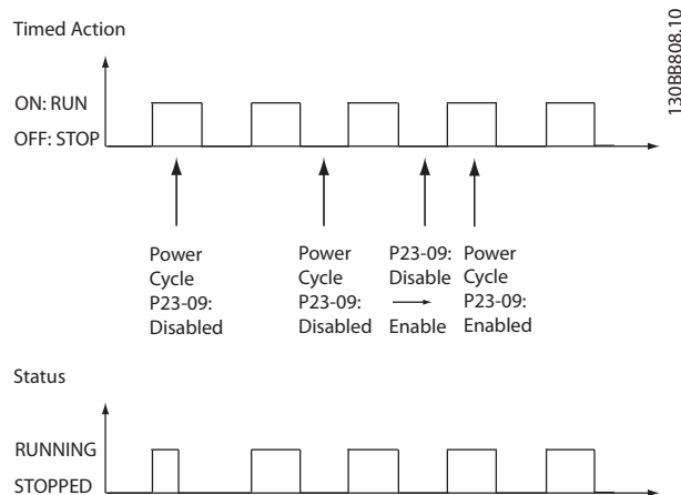
Рисунок 3.6 Схема тестов на восстановление
