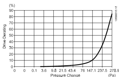
Рисунок 3.31: Корпус E Снижение значений относит. Изменение давления (Малый вентилятор), P315T5 и P450T7-P500T7
