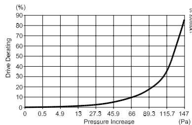
Рисунок 3.30: Корпус D Снижение значений относит. Изменение давления
