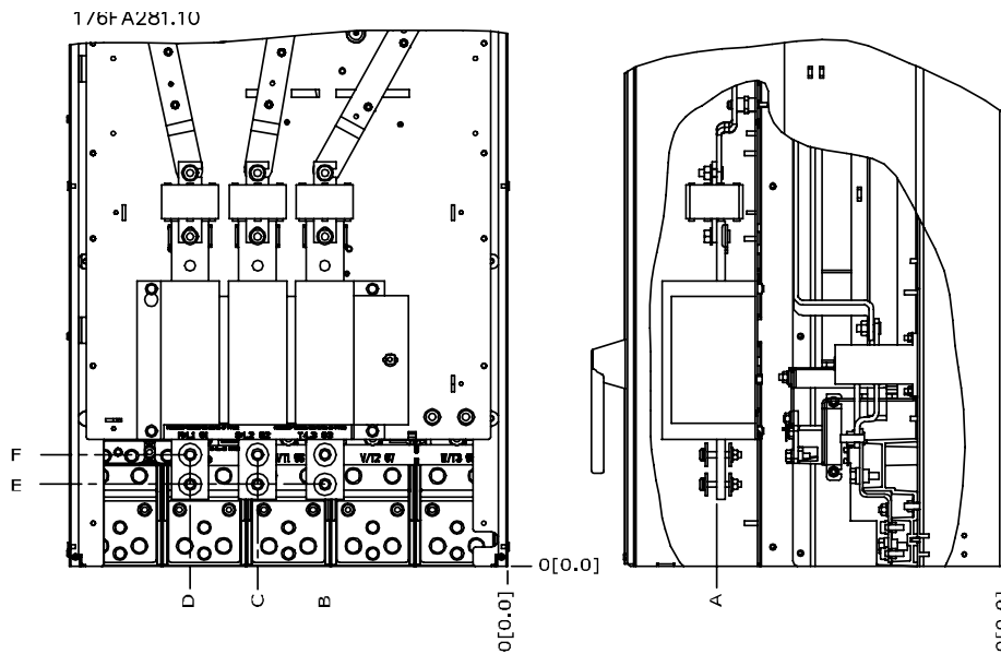
Рисунок 3.21: Расположение клемм электропитания корпуса IP00 с разъединителем
