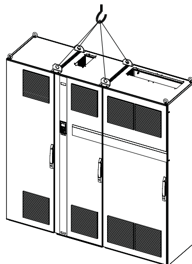
Рисунок 3.6: Рекомендуемый метод подъема, типоразмер F3.
