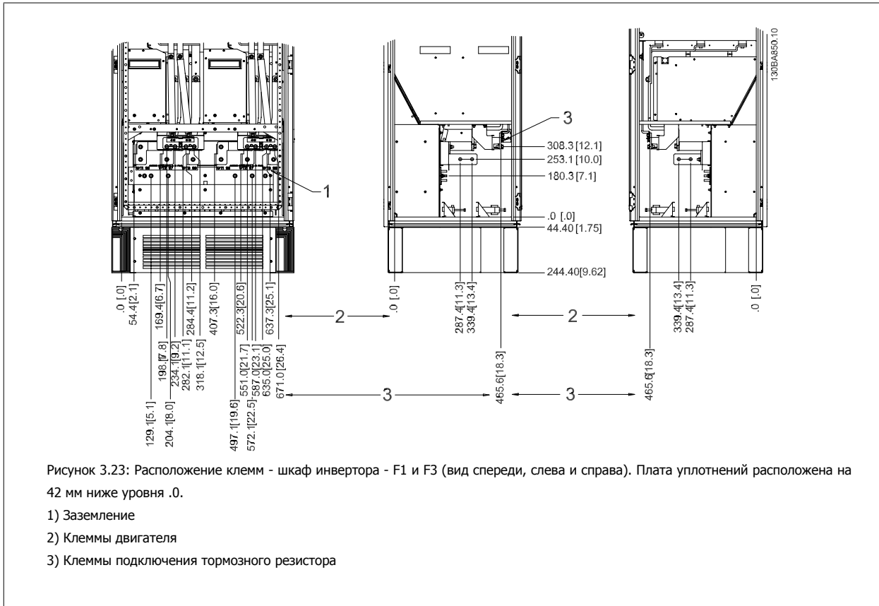
Расположение клемм - размеры корпуса F1 и F3
