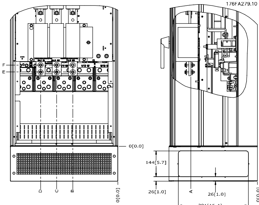
Рисунок 3.18: IP21 (NEMA type 1) и IP54 (NEMA type 12) расположение клемм электропитания корпуса
