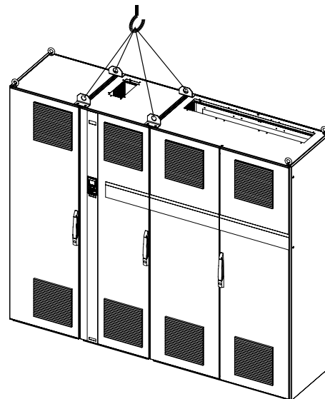
Рисунок 3.7: Рекомендуемый метод подъема, размер корпуса F4.
