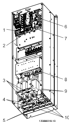
Рисунок 4.4: Compact IP 00 (Шасси) с разъединителем, плавким предохранителем и фильтром В4-помех размер корпуса D4
