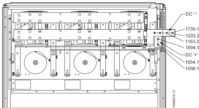
Рисунок 3.26: Расположение клемм – Реген клеммы - F2 и F4
