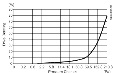
Рисунок 3.32: Корпус E Снижение значений относит. Изменение давления (Большой вентилятор), P355T5-P450T5 и P560T7-P630T7
