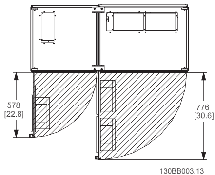
Рисунок 3.10: Пространство перед корпусом IP21/IP54 тип корпуса, размер корпуса F1
