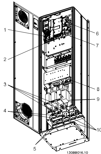
Рисунок 4.2: Compact IP 21 (NEMA 1) и IP 54 (NEMA 12) с разъединителем, плавким предохранителем и фильтром ВЧ-помех, размер корпуса D2
