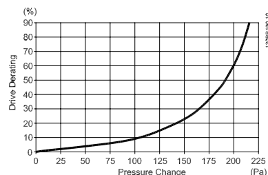
Рисунок 3.33: Корпус F1, F2, F3, F4 Снижение значений относит. Изменение давления
