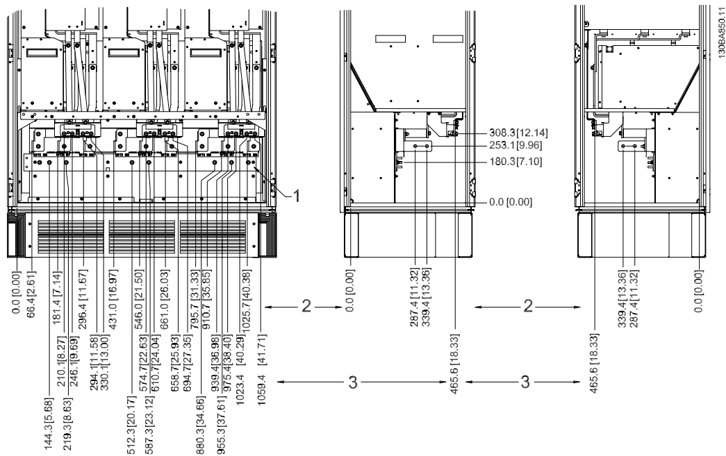
Рисунок 3.25: Расположение клемм - шкаф инвертора - F2 и F4 (вид спереди, слева и справа). Плата уплотнений расположена на 42 мм ниже уровня .0.
