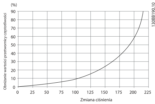
Ilustracja 4.23: Obniżenie wartości znamionowych ramy F w funkcji zmiany ciśnienia Przepływ powietrza przez przetwornicę: 985 m 3 /h (580 cfm)
