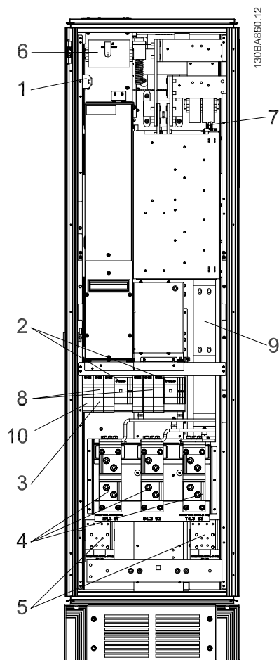
Ilustracja 4.31: Szafka prostownika, rozmiar ramy F17
