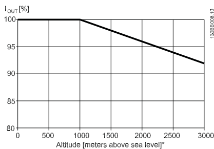
Déclassement du courant de sortie en fonction de l'altitude à T_{AMB, MAX} pour les châssis de taille D, E et F.
