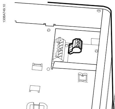
Illustration 5.36: Bornes pour le raccordement de relais pour C3 et C4. Situées dans l'angle supérieur droit du variateur de fréquence.
