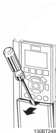
Illustration 5.37: Accès aux bornes de commande pour protections A2, A3, B3, B4, C3 et C4
