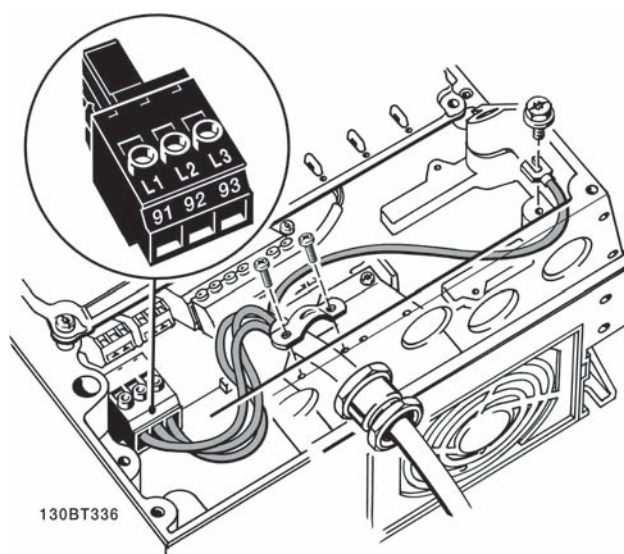
Illustration 5.6: Connexion au secteur et à la terre sans sectionneur secteur. Noter qu'un étrier de serrage est utilisé.
