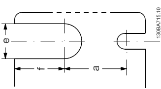
Illustration 4.2: Trous de fixation supérieurs et inférieurs. (B4+C3+C4 uniquement)
