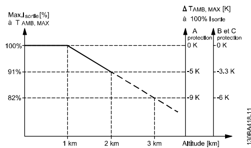
Illustration 10.1: Déclassement du courant de sortie en fonction de l'altitude à T_{AMB, MAX} pour les châssis de taille A, B et C. À des altitudes de plus de 2000 m, merci de contacter Danfoss en ce qui concerne la norme PELV.
