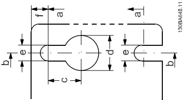
Ilustración 4.1: Agujeros de montaje superior e inferior.
