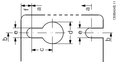
圖 4.1: 頂部與底部安裝孔。
