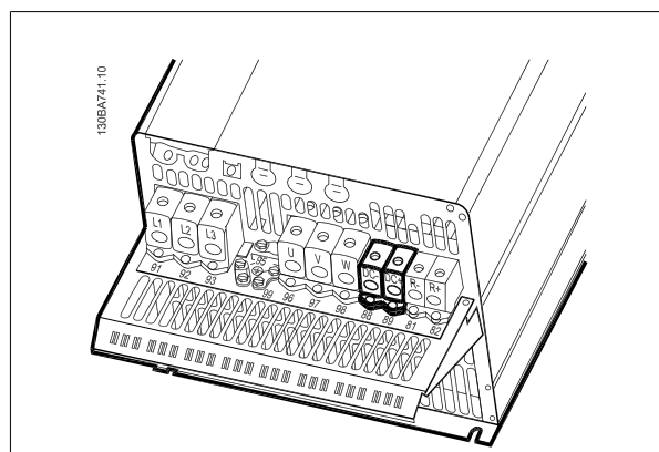
Рисунок 5.28: Подключение шины постоянного тока для корпуса C4.
