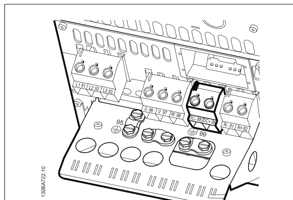
Рисунок 5.26: Подключение шины постоянного тока для корпуса B4.
