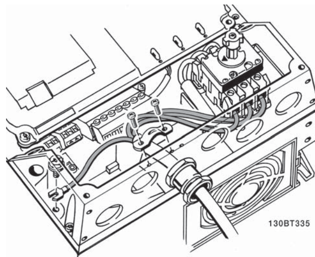
Ilustrasi 5.7: Cara menyambung ke hantaran listrik dan pembumian dengan saklar pemutus sumber listrik.
