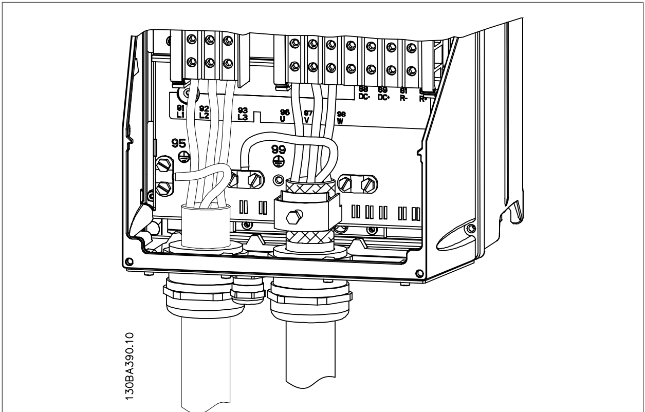
Ilustrasi 5.22: Pertama-tama putus dahulu hubungan pembumian motor, kemudian pasang kabel U, V, dan W pada terminal dan kencangkan. Pastikan bahwa isolasi luar kabel motor sudah dilepas dari penjepit EMC.
