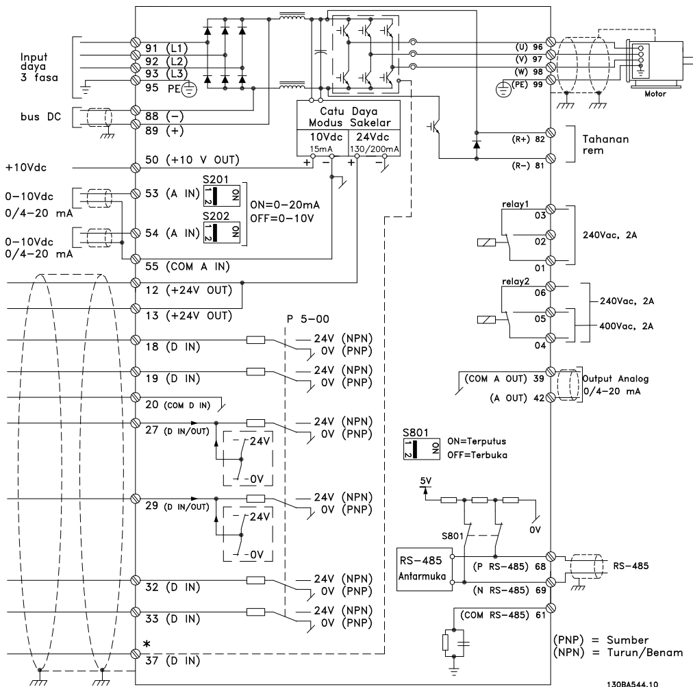
Ilustrasi 5.41: Diagram yang menunjukkan semua terminal listrik. (Terminal 37 hanya berlaku untuk unit dengan Fungsi Stop Aman saja.)
