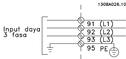
Ilustrasi 5.1: Terminal untuk hantaran listrik dan pembumian.
