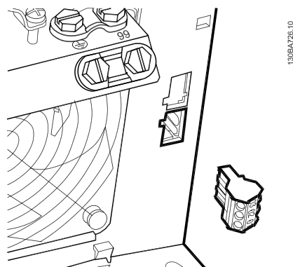
Ilustrasi 5.34: Terminal untuk sambungan relai B3 Hanya satu input relai yang terpasang dari pabrik. Ketika relai yang kedua diperlukan, lepaskan knock-out.
