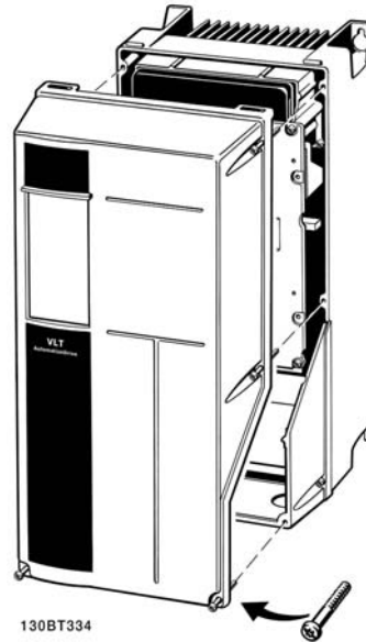
Ilustrasi 5.38: Jalan masuk penutup A5, B1, B2, C1 dan C2 ke terminal kontrol
