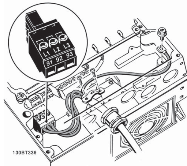
Ilustrasi 5.6: Cara menyambung ke hantaran listrik dan pembumian tanpa saklar pemutus hantaran listrik. Ingat bahwa di sini digunakan penjepit kabel.
