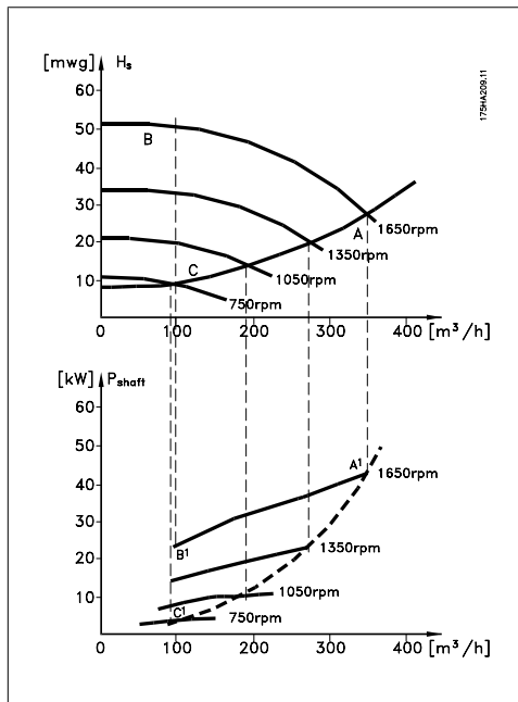
Características da bomba
