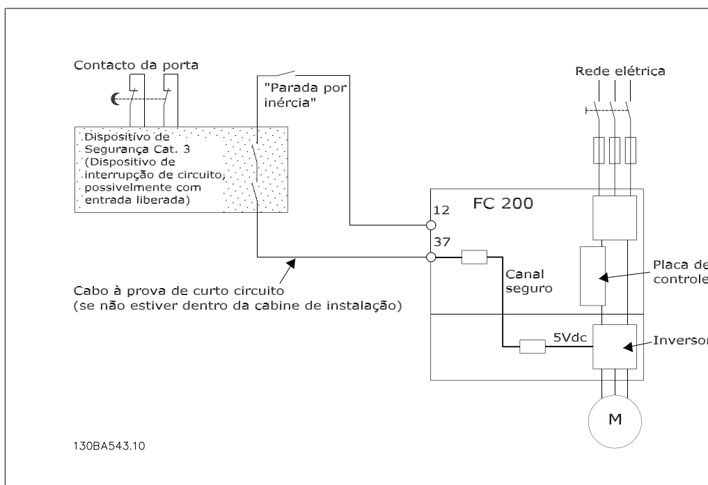
Ilustração 5.18: Ilustração dos aspectos essenciais de uma instalação para obter uma Categoria de Parada 0 (EN 60204-1), com Cat. de segurança 3 (En 954-1)
