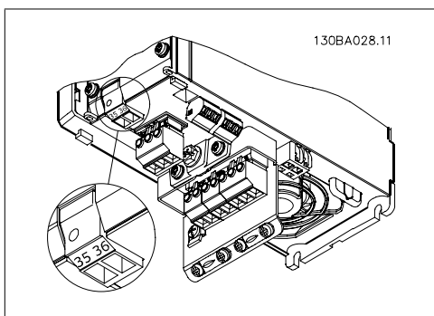
Ilustração 3.11: Conexão à alimentação de backup de 24 V (A2-A3).
