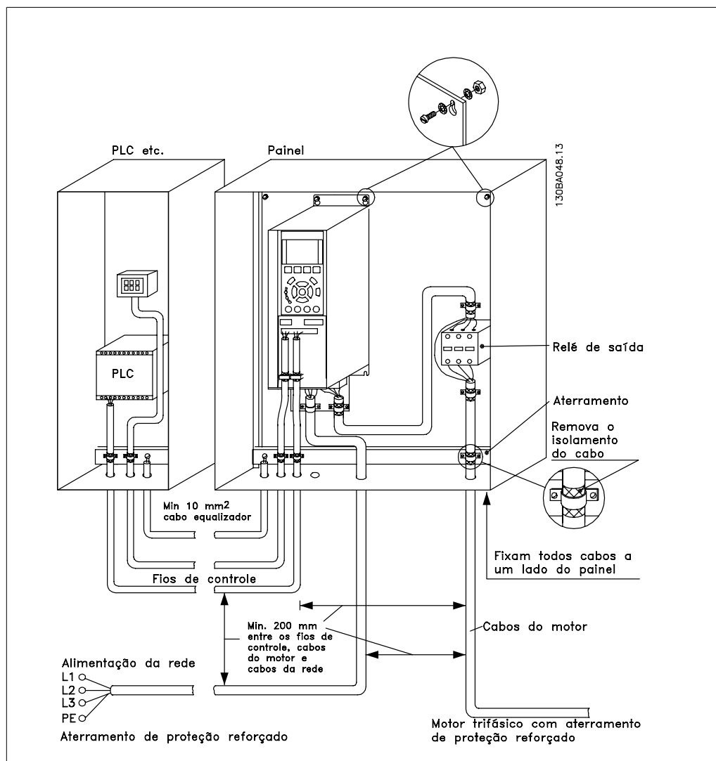
Ilustração 5.20: Instalação elétrica correta de EMC de um conversor de frequência.
