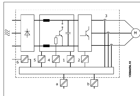
Ilustração 2.2: Isolação galvânica
