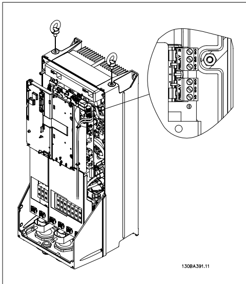
Ilustração 5.19: Terminais para conexão de relé (Gabinetes metálicos C1 e C2).
