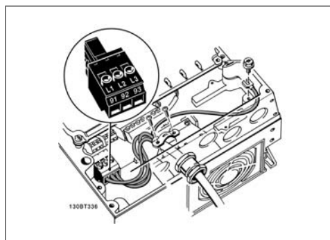
Ilustração 5.2: Como fazer a conexão à rede elétrica e ao ponto de aterramento (gabinete metálico A5).
