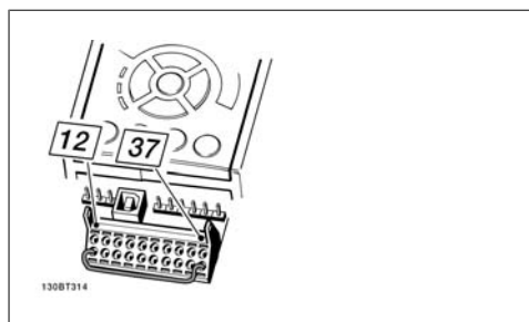
Ilustração 5.17: Coloque um jumper de conexão entre o terminal 37 e os 24 VCC.
