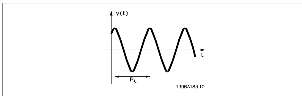
Ilustração 2.1: Figura 1: Sistema marginalmente estável
