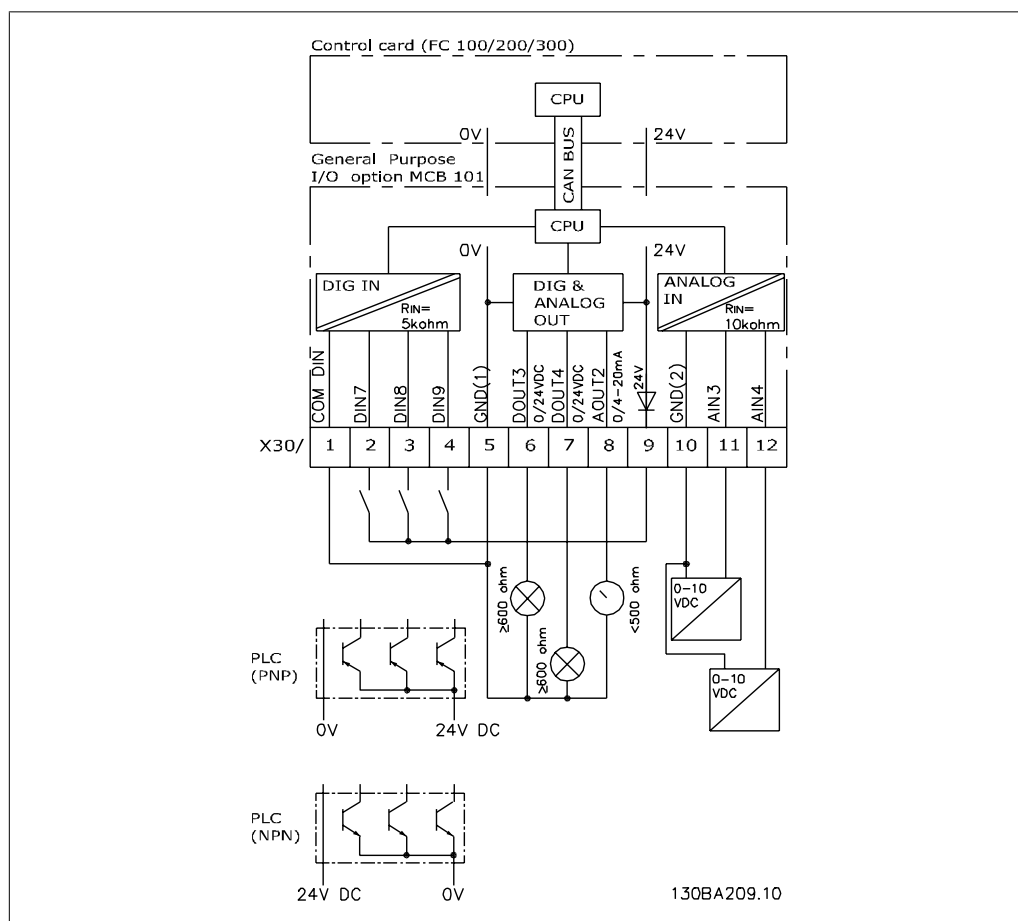
Ilustração 3.10: Diagrama de Princípios
