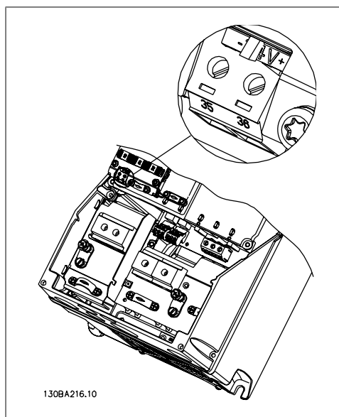
Ilustração 3.12: Conexão à alimentação de 24 V de backup (A5-C2).
