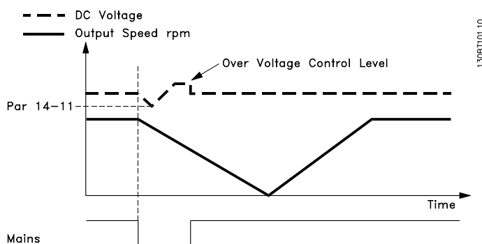
图 2.2: 受控减速—主电源短时间故障。减速直到停止, 接着减速到参考值。
