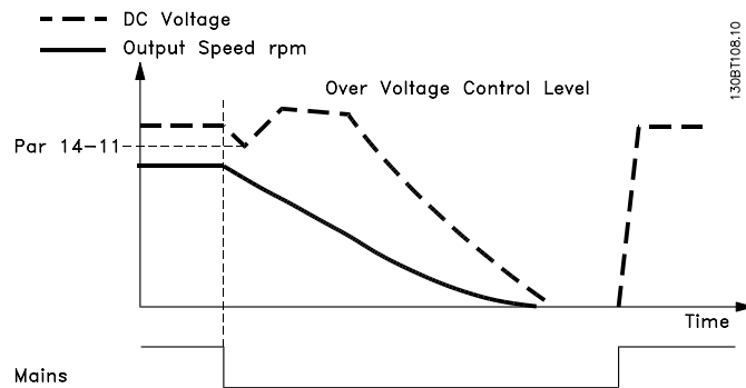
图 2.3: 受控减速—主电源长时间故障。只要系统中的能量允许,便进行减速,之后电动机将惯性停车。
