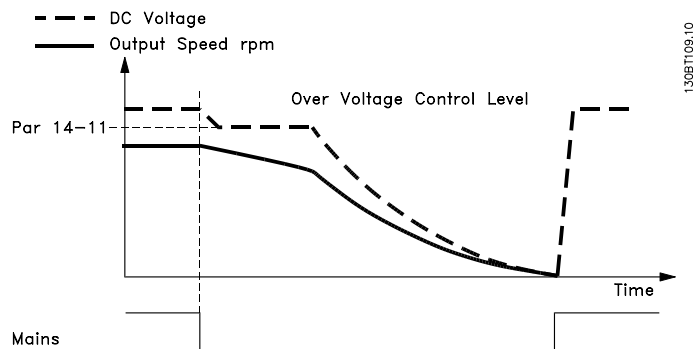
图 2.5: 借能运行, 主电源长时间故障。一旦系统中的能量过低,电动机就会惯性停车。
