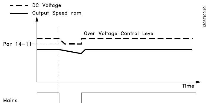
图 2.4: 借能运行, 主电源短时间故障。只要系统中的能量允许,便保持运行。
