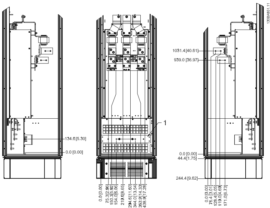
Bild 4.17: Plintplaceringar - Filter (framifrån, från vänster och höger). Boxplåten är 42 mm nedom .0-nivån.
