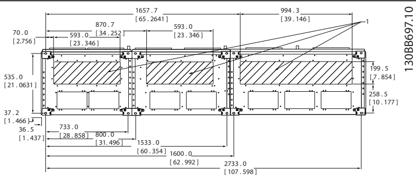
F8-F13: Kabelingångar sedda underifrån frekvensomformaren - 1) Placera genomföringar i de markerade områdena
