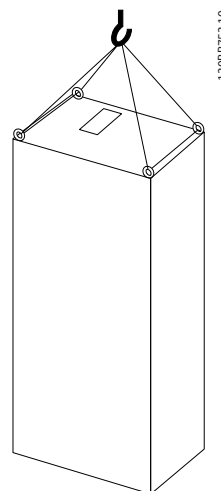
Bild 3.1 Rekommenderad lyftmetod, kapsling F8.
