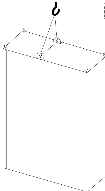
Bild 3.2 Rekommenderad lyftmetod, kapsling F9/F10.
