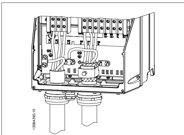
Рисунок 3.14: Подключение двигателя к преобразователям в корпусах C1 и C2 (IP 21/NEMA, тип 1, и IP 55/66/ NEMA, тип 12).
