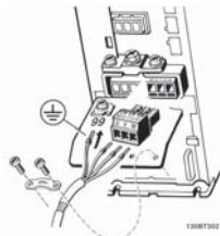
Рисунок 3.9: Подключение двигателей к преобразователям в корпусах A1, A2 и A3
