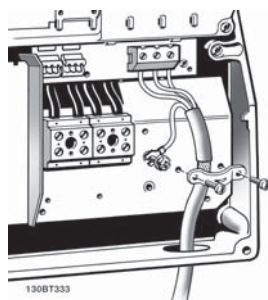
Рисунок 3.11: Подключение двигателей к преобразователям в корпусах B1 и B2 (IP 21/ NEMA, тип 1, IP 55/ NEMA, тип 12 и IP66/ NEMA, тип 4X).
