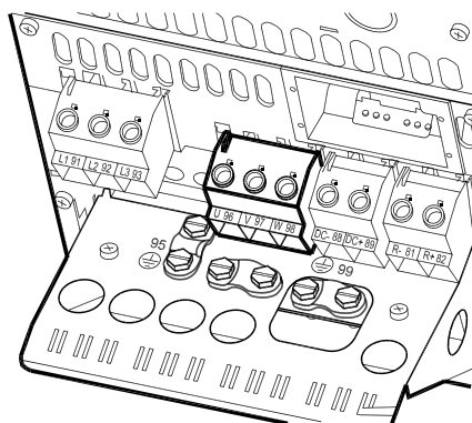
Рисунок 3.13: Подключение двигателя в корпусе B4.
