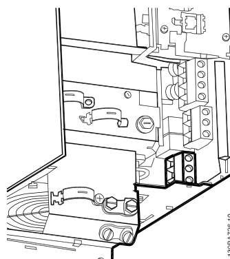
Рисунок 3.12: Подключение двигателя в корпусе B3.
