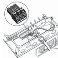
Рисунок 3.10: Подключение двигателя к преобразователю в корпусе A5 (IP 55/66/NEMA, тип 12).
