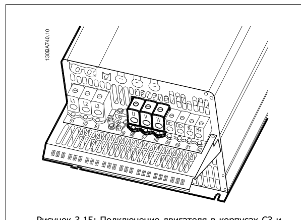
Рисунок 3.15: Подключение двигателя в корпусах C3 и C4.
