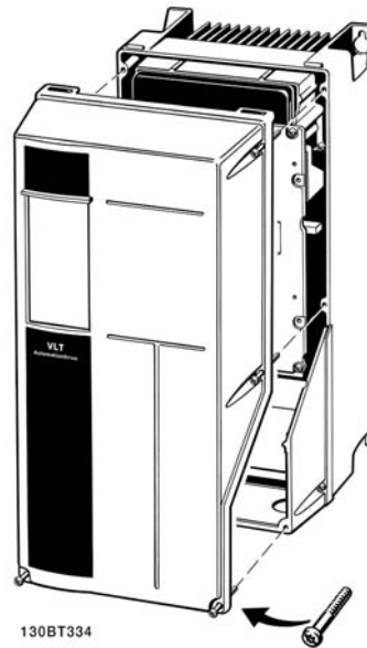
图 3.20: 访问 A5、B1、B2、C1 和 C2 机箱的控制端子
