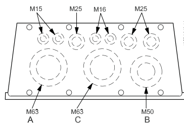
Obrázek 3.17: Otvory pro kabely pro velikost rámečku C1. Navrhované umístění otvorů je pouze doporučení a je možné použít i jiná řešení.
