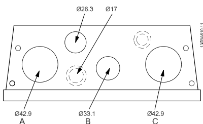
Obrázek 3.16: Otvory pro kabely pro velikost rámečku B2. Navrhované umístění otvorů je pouze doporučení a je možné použít i jiná řešení.
