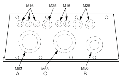
Obrázek 3.18: Otvory pro kabely pro velikost rámečku C2. Navrhované umístění otvorů je pouze doporučení a je možné použít i jiná řešení.
