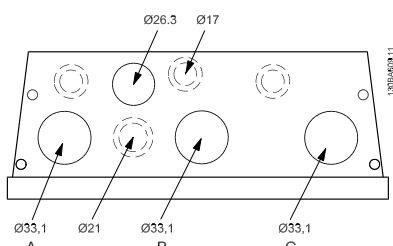
Obrázek 3.15: Otvory pro kabely pro velikost rámečku B1. Navrhované umístění otvorů je pouze doporučení a je možné použít i jiná řešení.
