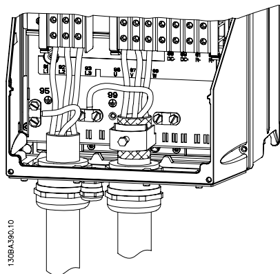
Obrázek 3.13: Připojení k motoru pro velikosti rámečků C1 a C2 (IP 21/ NEMA typ 1 a IP 55/66/ NEMA typ 12)
