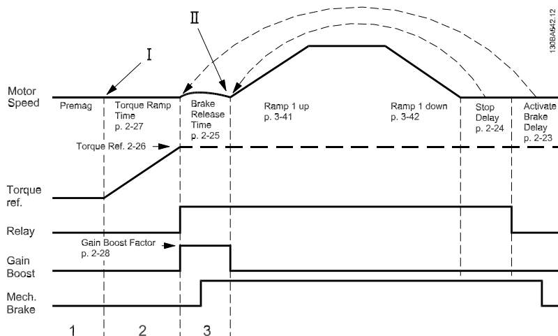
Kuva 4.1: Jarrun vapautusprosessi nostimen mekaanisen jarrun ohjausta varten
