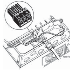
Kuva 3.8: Moottorin kytkentä koolle A5 (IP 55/66/NEMA-tyyppi 12)
