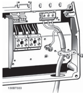
Kuva 3.9: Moottorin kytkentä ko'oilte B1 ja B2 (IP 21/ NEMA-tyyppi 1, IP 55/ NEMA-tyyppi 12 ja IP66/ NEMA-tyyppi 4X)
