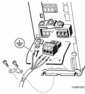
Kuva 3.7: Moottorin kytkentä malleille A1, A2 ja A3
