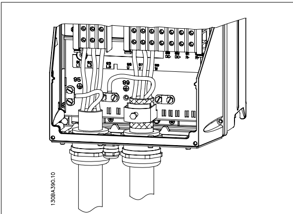
图 3.12: 机架规格 C1 和 C2 (IP 21/NEMA 类型 1 和 IP 55/66/ NEMA 类型 12) 的电动机接线
