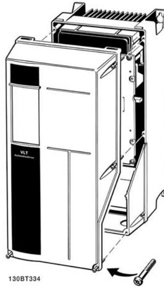
图 3.19: 访问 A5、B1、B2、C1 和 C2 机箱的控制端子
