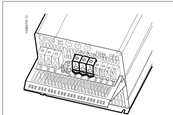
图 3.13: 机架规格 C3 和 C4 的电动机接线。
