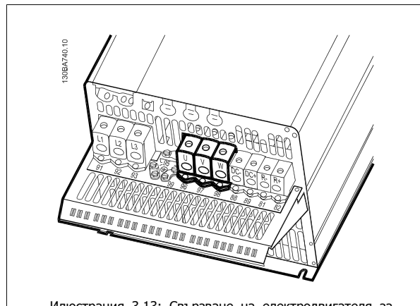
Илюстрация 3.13: Свързване на електродвигателя за размер на рамка C3 и C4.
