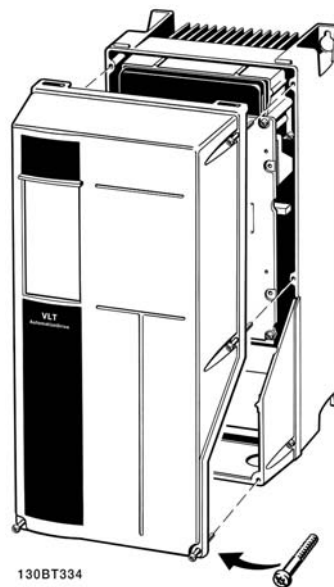
Илюстрация 3.19: Достъп до клемите на управлението за обвивки A5, B1, B2, C1 и C2
