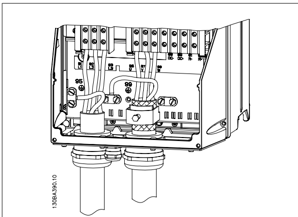
Илюстрация 3.12: Свързване на електродвигателя за размер на рамка C1 и C2 (IP 21/ NEMA тип 1 и IP 55/66/ NEMA тип 12)
