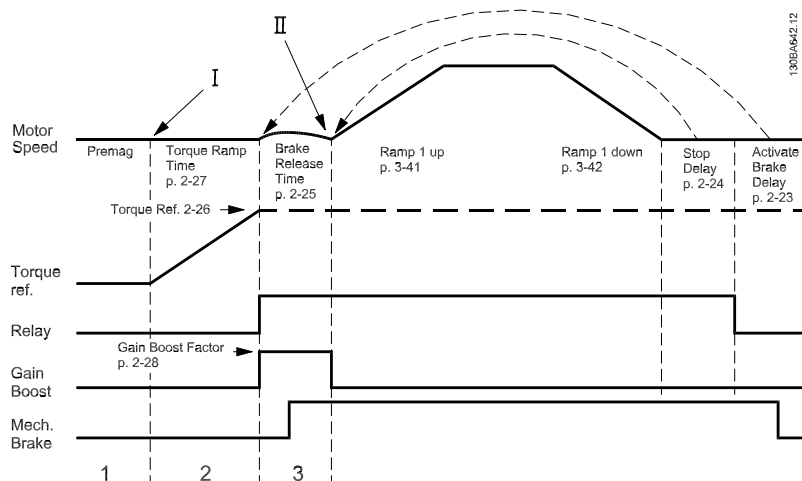
Ilustrația 4.1: Secvență de eliberare a frânei pentru controlul frânei mecanice la ridicare
