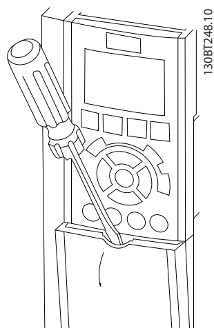
图 2.9 访问 A2、A3、B3、B4、C3 和 C4 机箱的控制端子
