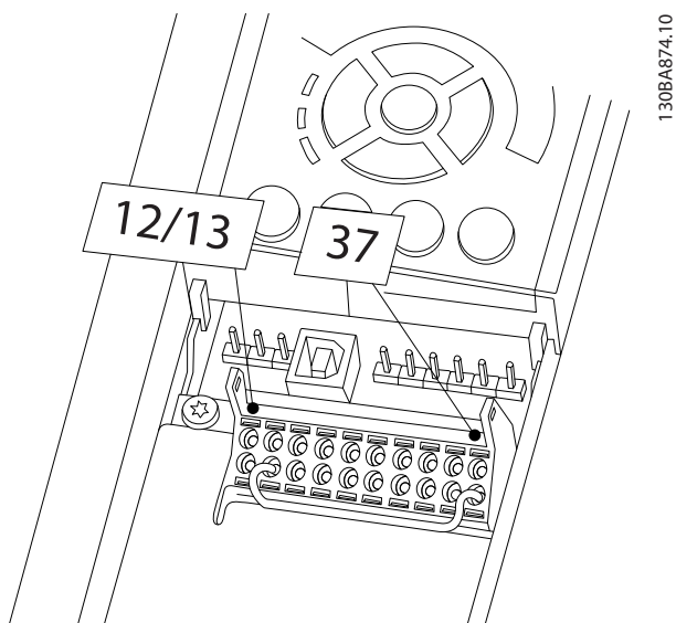
图 2.15 端子 12/13 (24V) 与 37 之间的跳线
