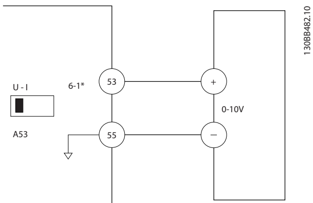
图 5.1 由外部设备提供 0-10V 控制信号的接线示例（左为变频器，右为外部设备）
