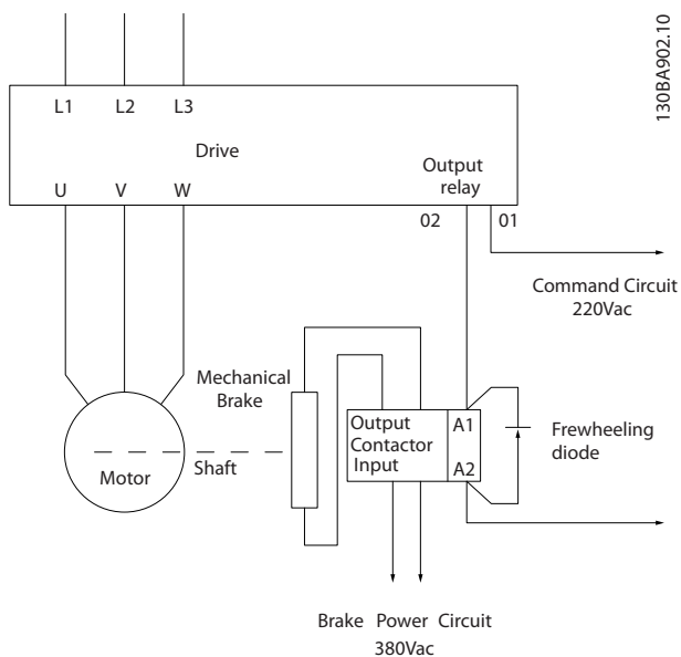
图 2.17 将机械制动连接到变频器
