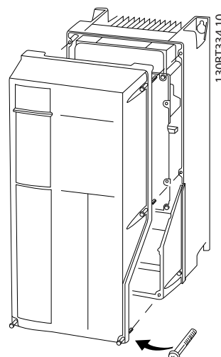
图 2.10 访问 A4、A5、B1、B2、C1 和 C2 机箱的控制端子
